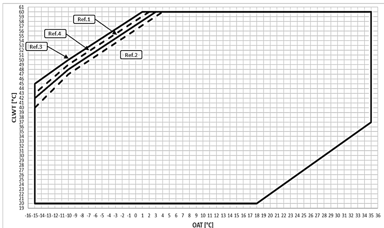
Fig. 8 – EWYT~B-X – OP.204 Límites Operativos del Modo de Calentamiento
