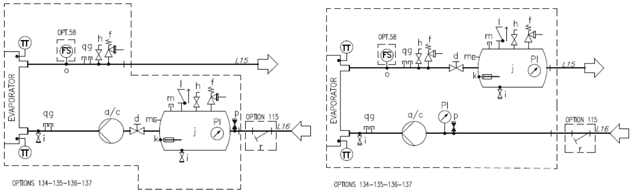
Fig. 16 – Diagrama hidráulico para bomba única / dos bombas con tanque (EWYTx5B) (opc. 134-135) (presión operativa máxima 6 bares)
