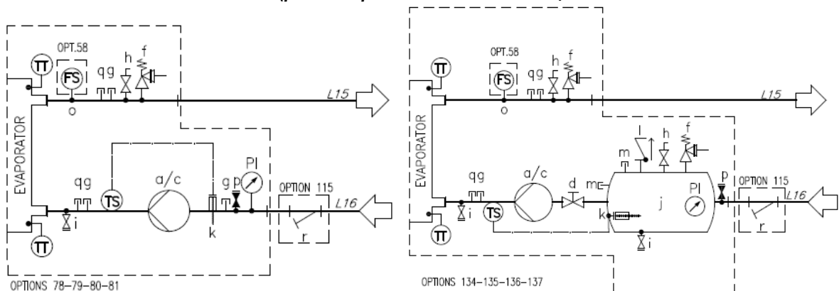
Fig. 17 – Diagrama hidráulico para bomba doble (EWYTx5B) (opc. 80-81/136-137) (presión operativa máxima 6 bares)
