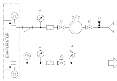
Fig. 14 – Diagrama hidráulico sin bomba(s) a bordo (presión operativa máxima 20 bares)
