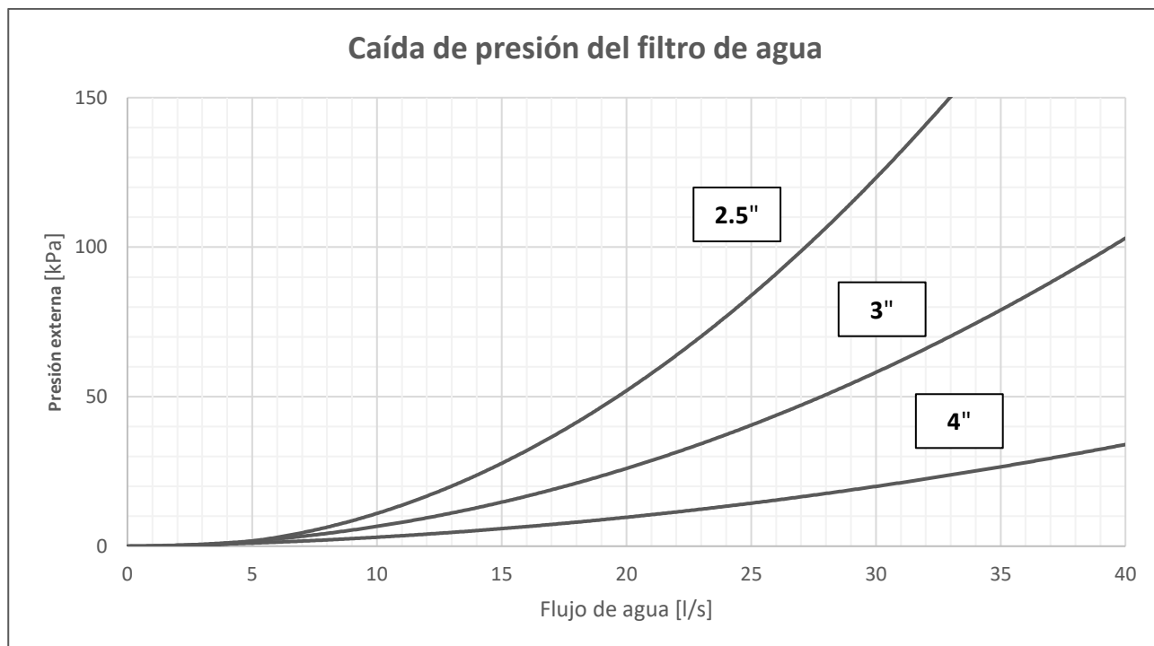
Fig. 13 – Pérdida de presión del filtro de agua
