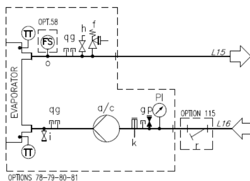
Sl. 15 – Hidraulički dijagram za jednu pumpu / dvostruku pumpu (EWYTx5B) (opt. 78-79) (maks. radni tlak 6 bara)
