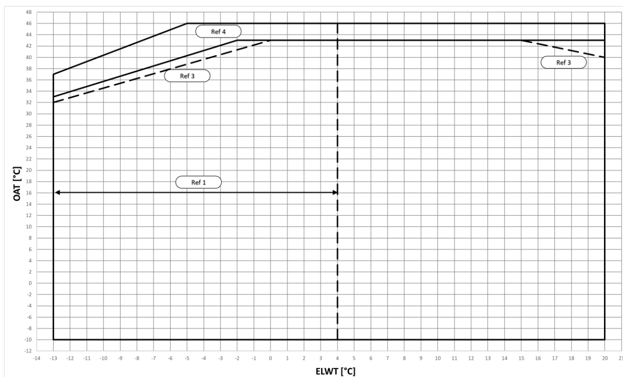
Sl. 1 – Radne granice EWYTx5B-S načina hlađenja
