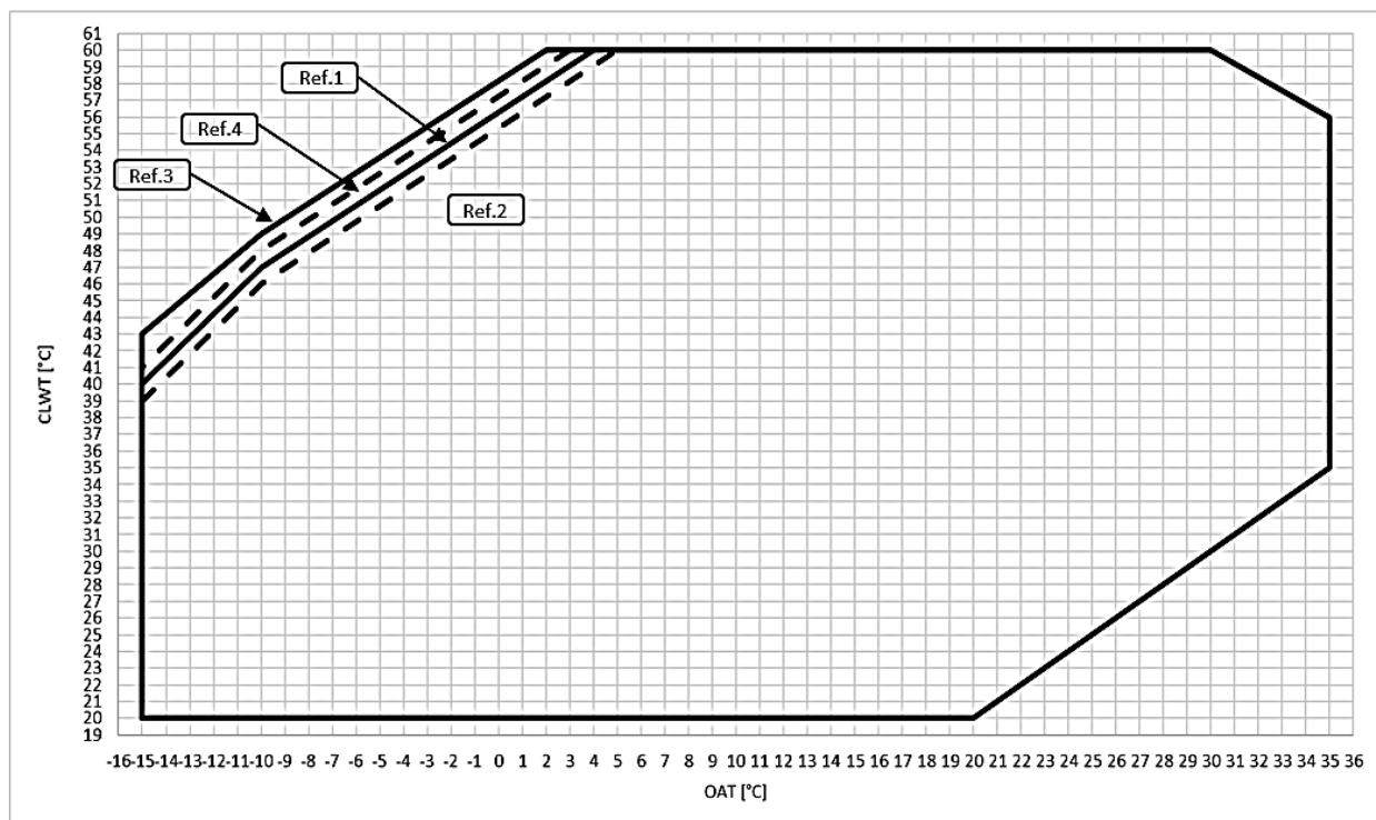
Sl. 7 – EWYT~B-S – OP.204 Ograničenja rada načina grijanja
