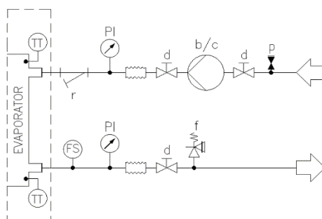
Sl. 14 – Hidraulički dijagram bez pumpe na brodu (maks. radni tlak 20 bar)
