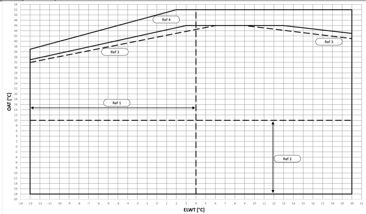
Fig. 3 – Limites operativos do modo de refrigeração EWYTxx0B-S
