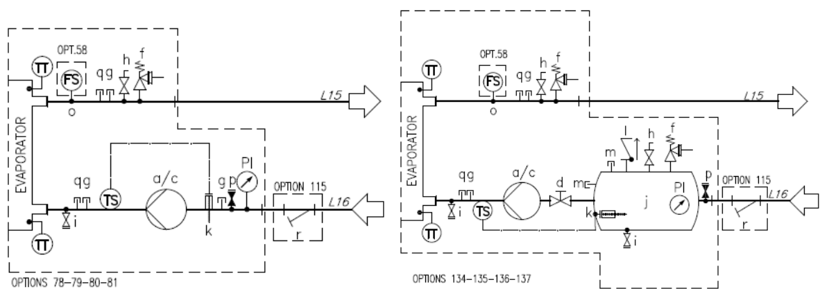
Fig. 18 – Diagrama hidráulico para bomba única / bomba dupla (opc. 78-79-80-81/134-135-136-137) (pressão máxima de funcionamento 6 bar)
