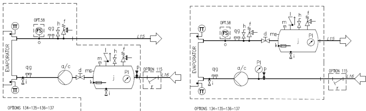
Fig. 16 – Diagrama hidráulico para bomba única / bomba dupla com tanque (EWYTx5B) (opc. 134-135) (pressão máxima de funcionamento 6 bar)
