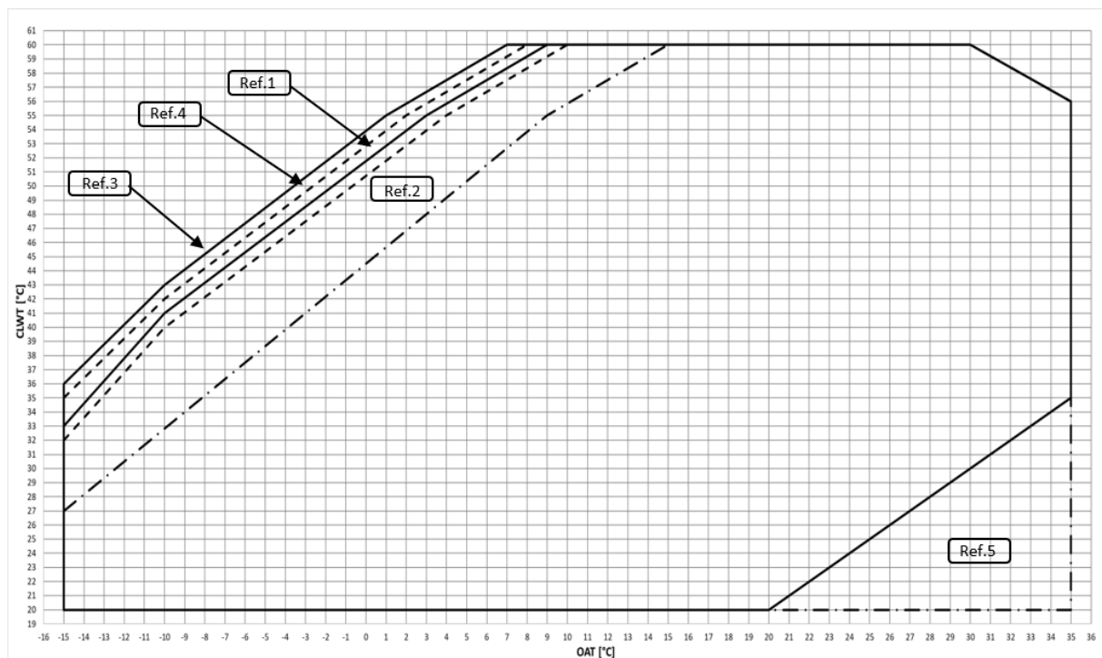
Fig. 5 – Limites operativos do modo de aquecimento EWYT-B-S
