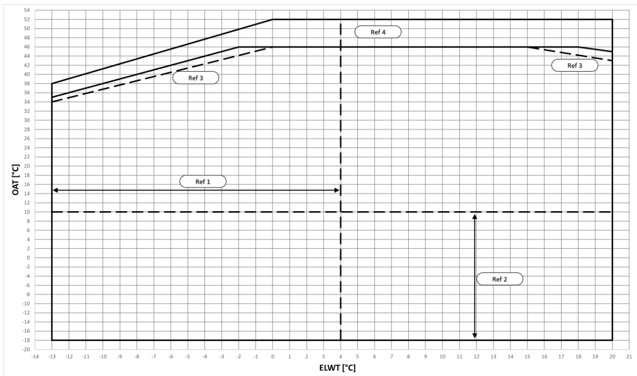
Fig. 4 – Limites operativos do modo de refrigeração EWYTxx0B-X
