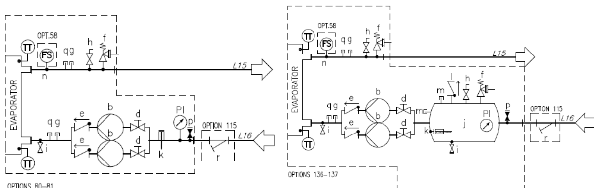
Fig. 17 – Diagrama hidráulico para bomba dupla (EWYTx5B) (opc. 80-81/136-137) (pressão máxima de funcionamento 6 bar)
