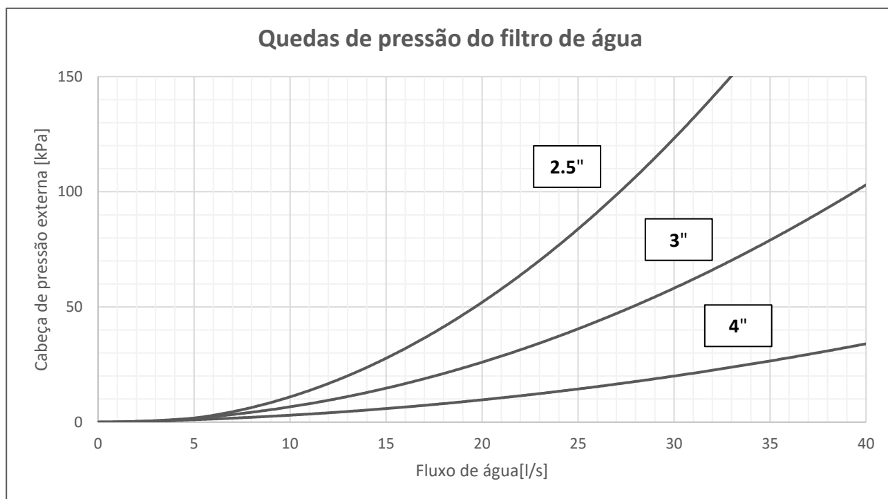
Fig. 13 – Queda de pressão no filtro de água
