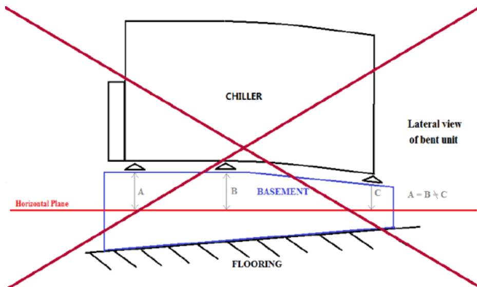
Fig. 10 – Nivelamento da unidade
