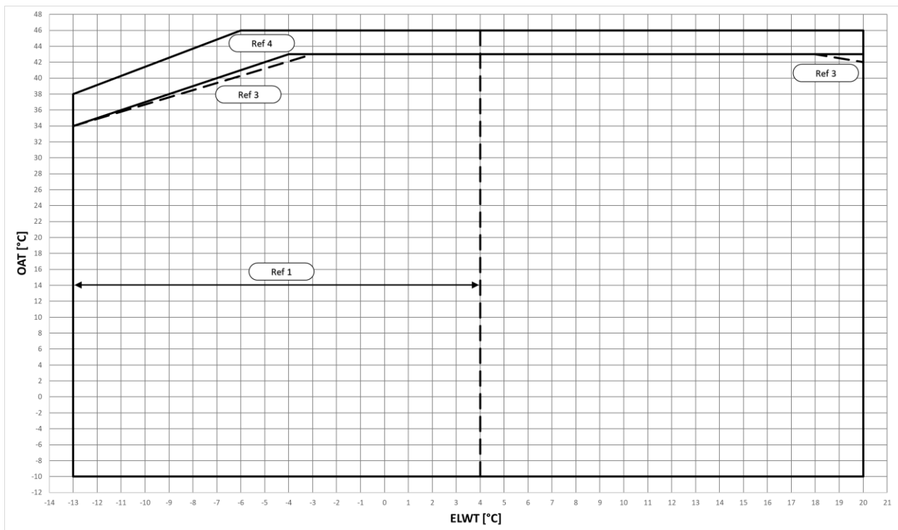
Fig. 2 – Limites operativos do modo de refrigeração EWYTxx5B-X
