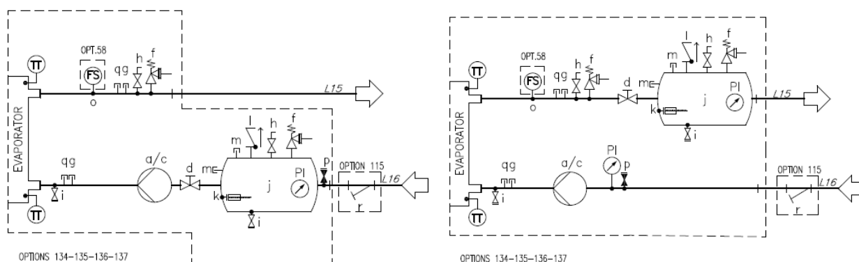
Slika 16 – Hidravlična shema za eno črpalko / dvojno črpalko z rezervoarjem (EWYTx5B) (opc. 134-135)
