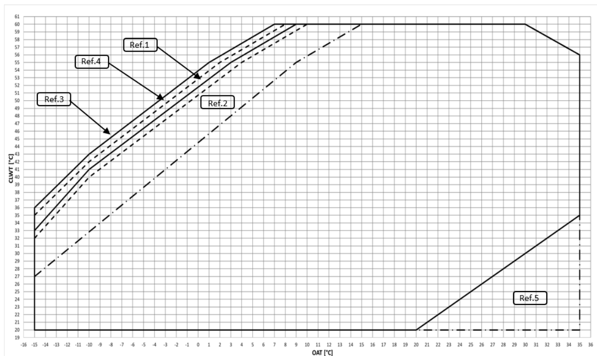
Slika 5 – EWT ~B-S Delovne omejitve načina ogrevanja
