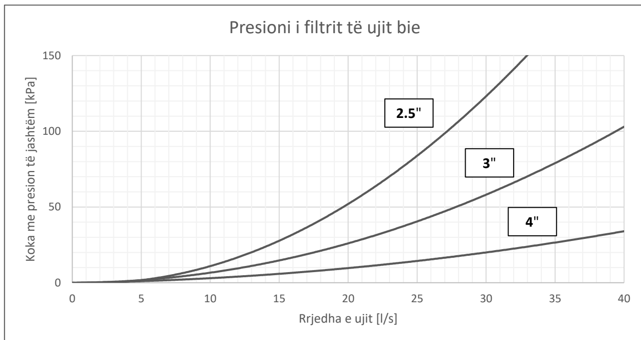
Fig.13– Rënia e presionit të filtrit të ujit
