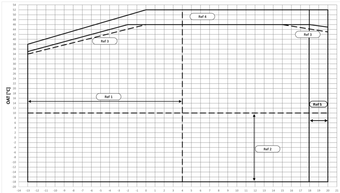
Fig. 4 – EWYTx0B-X Límites Operativos del Modo de Enfriamiento
