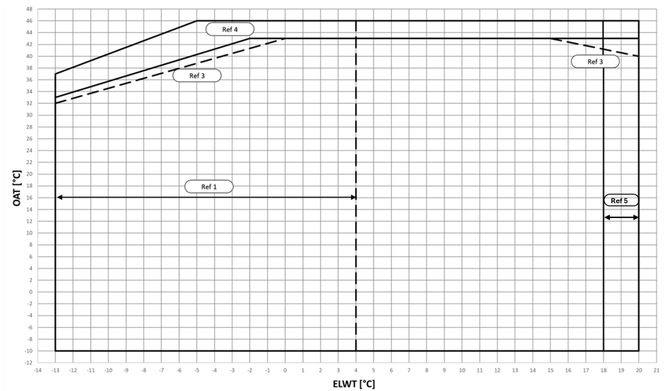
Fig. 1 – EWYTx5B-S Límites Operativos del Modo de Enfriamiento
