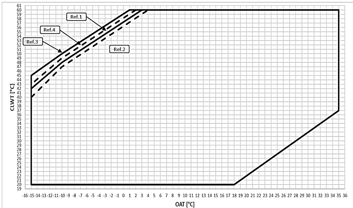
Fig. 8 – EWYT~B-X – OP.204 Límites Operativos del Modo de Calentamiento
