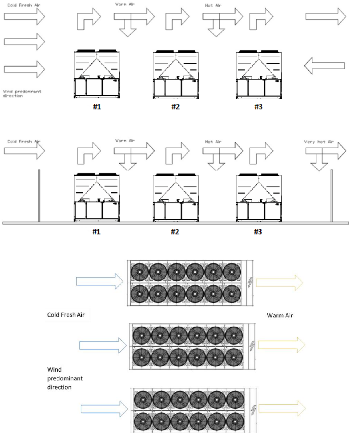
Fig. 12 – Instalación de múltiples unidades (modo de enfriamiento)
