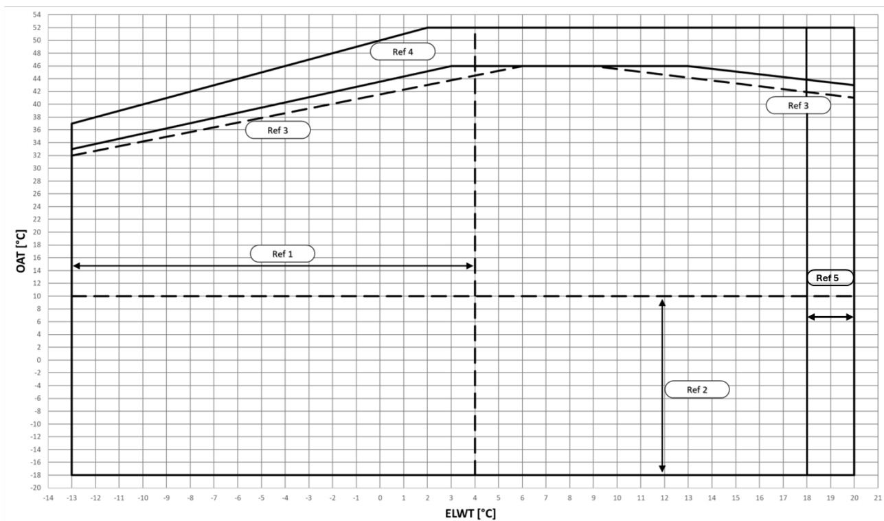
Fig. 3 – EWYTx0B-S Límites Operativos del Modo de Enfriamiento
