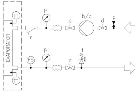
SI. 14 – Hidraulički dijagram bez pumpi na brodu (maks. radni tlak 20 bar)
