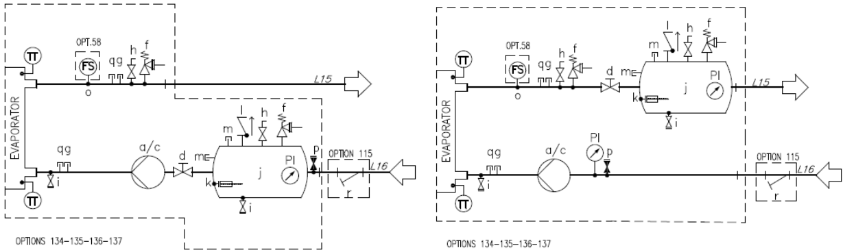
SI. 16 – Hidraulički dijagram za jednu pumpu / dvostruku pumpu s spremnikom (EWYTx5B) (opt. 134-135) (maks. radni tlak 6 bara)
