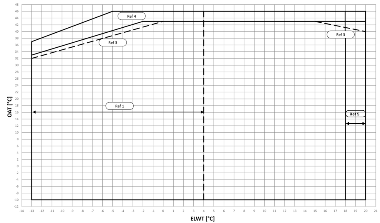
Sl. 1 – Radne granice EWYTx5B-S načina hlađenja
