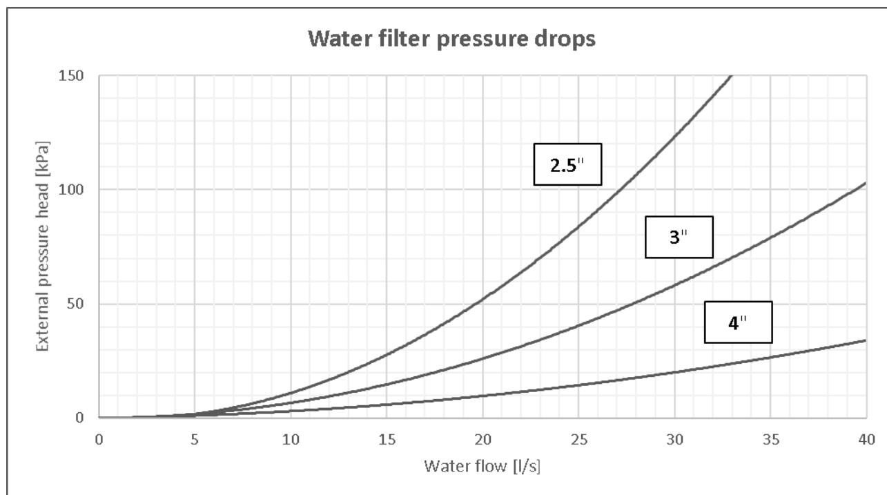
Sl. 13 – Pad tlaka filtra za vodu
