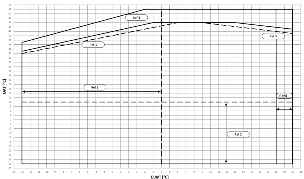
SI. 3 – Radne granice EWYTx0B-S načina hlađenja
