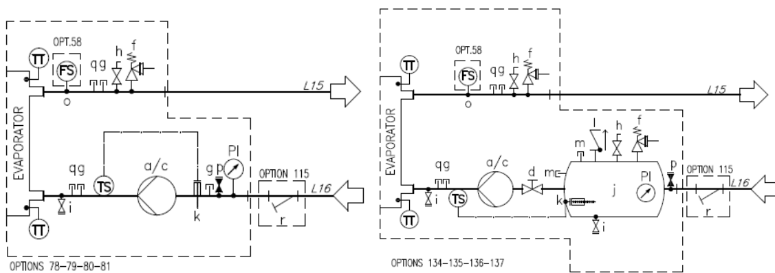
Sl. 18 – Hidraulički dijagram za jednu pumpu / dvostruku pumpu (opcija 78-79-80-81/134-135-136-137) (maks. radni tlak 6 bara)
