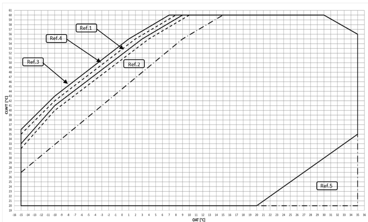
SI. 5 – Radne granice EWYT ~ B-S načina grijanja
