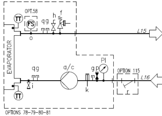
SI. 15 – Hidraulički dijagram za jednu pumpu / dvostruku pumpu (EWYTx5B) (opt. 78-79) (maks. radni tlak 6 bara)
