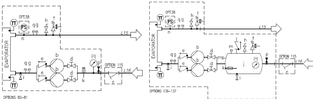
SI. 17 – Hidraulički dijagram za dvostruku pumpu (EWYTx5B) (opcija 80-81/136-137) (maks. radni tlak 6 bara)
