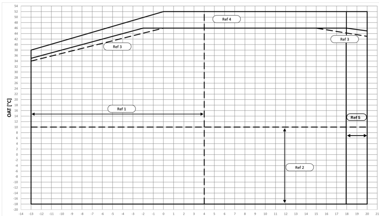
SI. 4 – Radne granice EWYTx0B-X moda hlađenja
