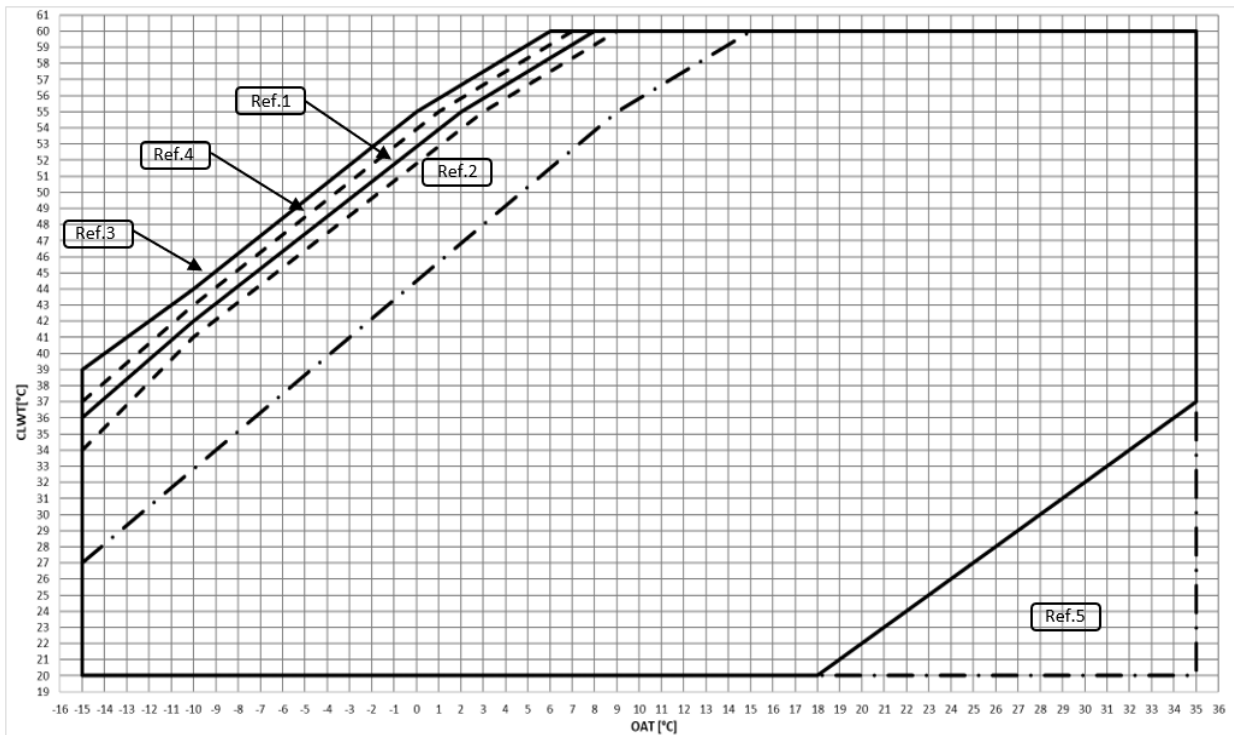
SI. 6 – Radne granice EWYT ~ B-X načina grijanja
