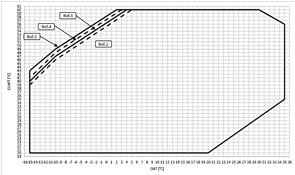
SI. 7 – EWYT~B-S – OP.204 Ograničenja rada načina grijanja
