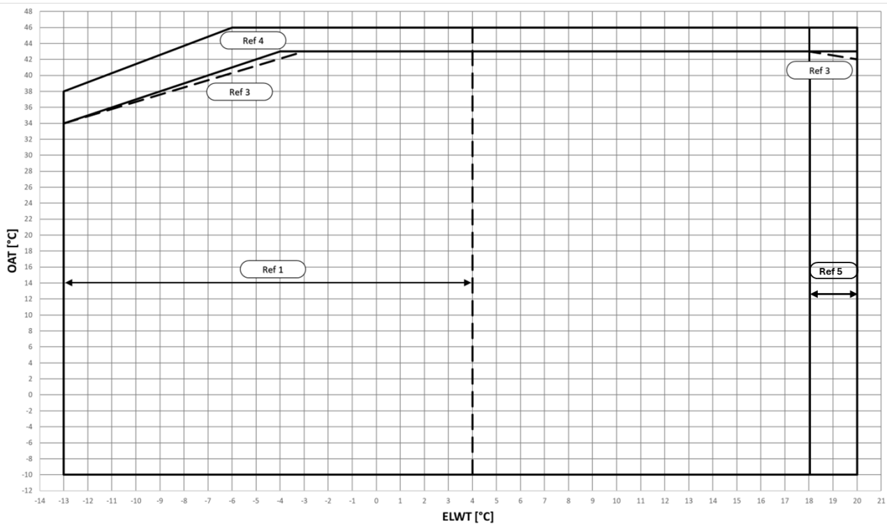
SI. 2 – Radne granice EWYTx5B-X moda hlađenja
