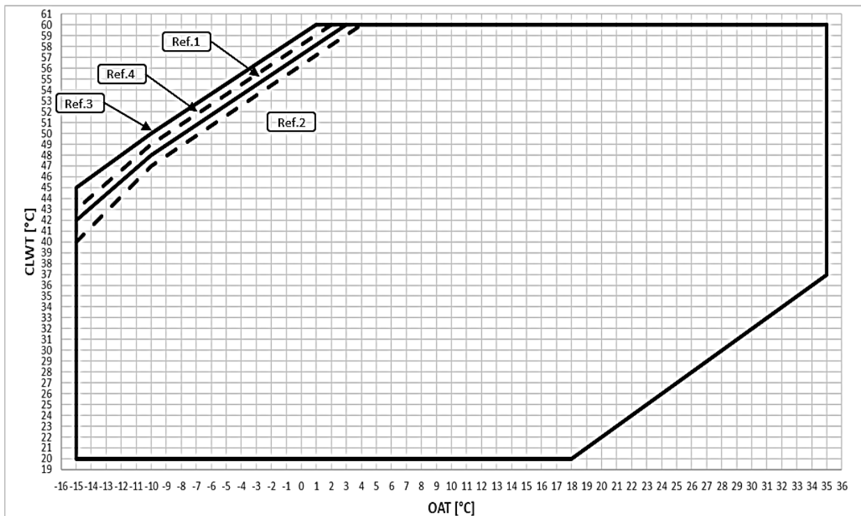
Sl. 8 – EWYT ~B-X – OP.204 Ograničenja rada načina grijanja
