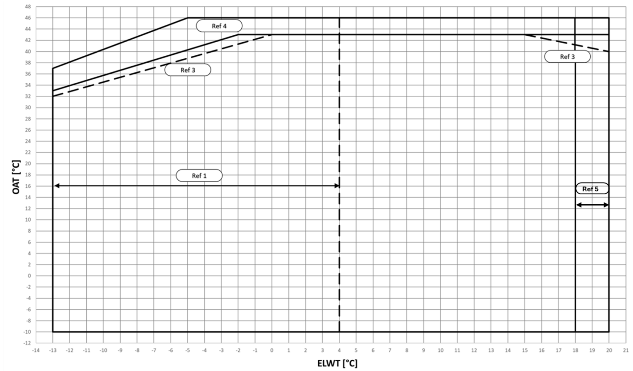
Fig. 1 - Limiti operativi della modalità di raffreddamento di EWYTx5B-S
