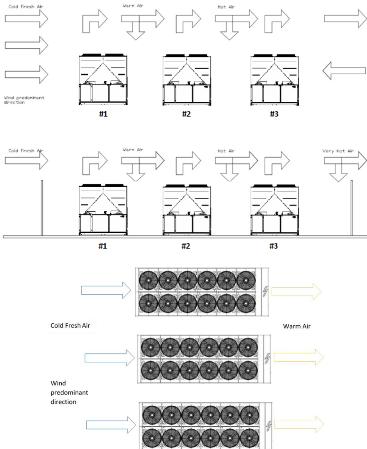
Fig. 12 - Installazione di più unità (modalità di raffreddamento)
