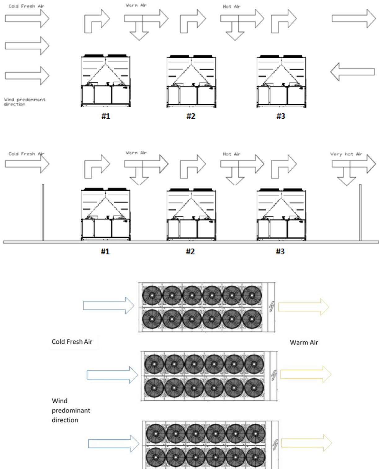
Fig. 12 – Instalação de várias unidades (modo de refrigeração)
