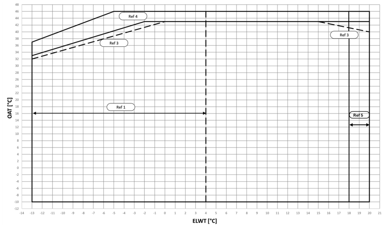
Fig. 1 – Limites operativos do modo de refrigeração EWYTx5B-S
