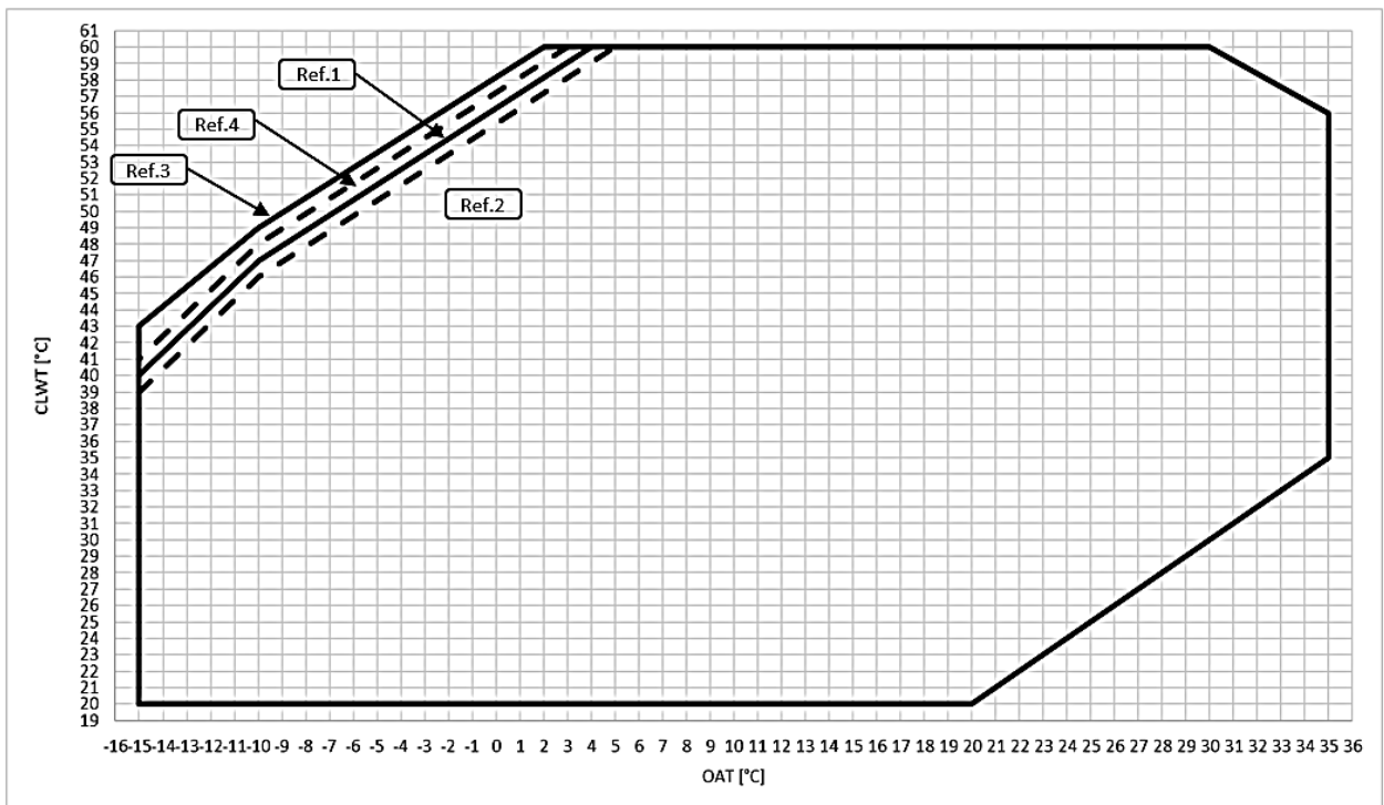
Fig. 7 – Limites operativos do modo de aquecimento OP.204 – EWYT-B-S
