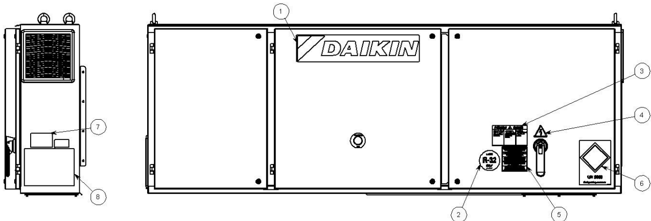
Fig. 23 – Descrição das etiquetas aplicadas no painel elétrico EWYTx0B
