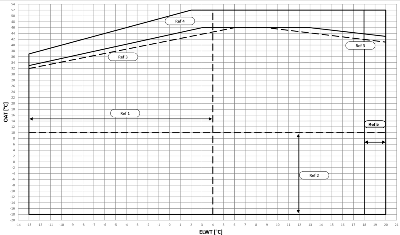
Fig. 3 – Limites operativos do modo de refrigeração EWYTx0B-S
