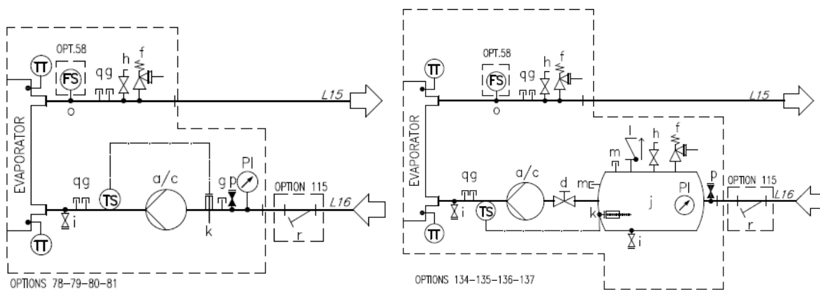
Fig. 18 – Diagrama hidraulică pentru o singură pompă /pompă dublă (opt. 78-79-80-81/134-135-136-137) (presiune max. de operare 6 bari)
