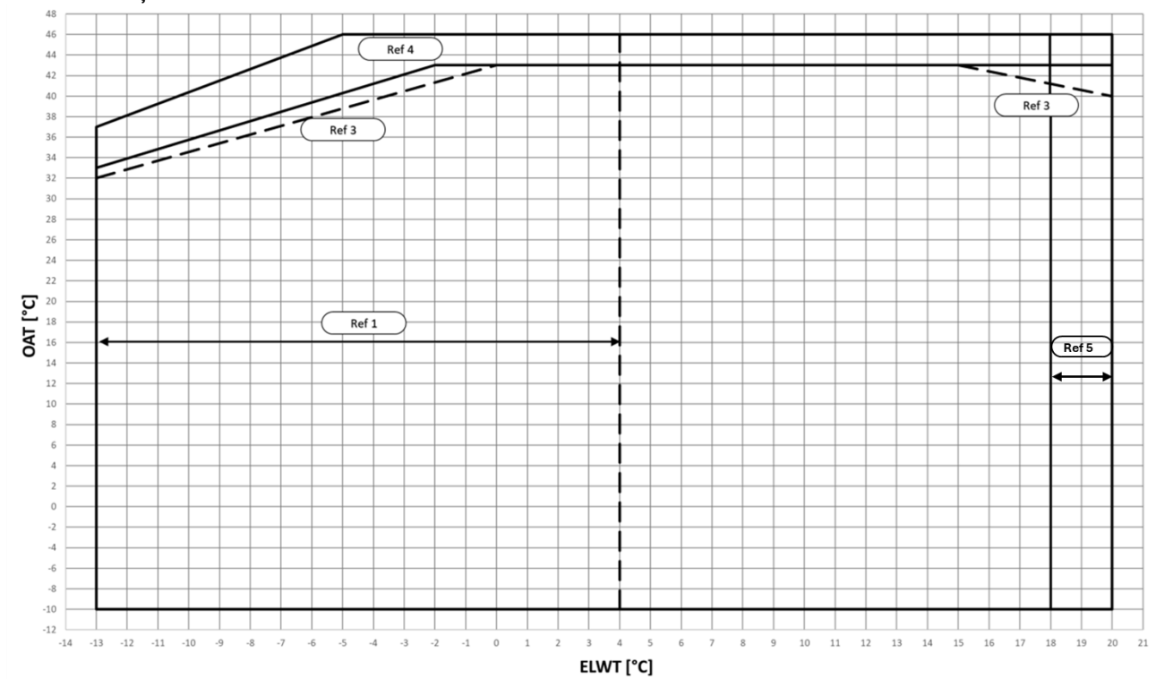
Fig. 1 – EWYTx5B-S Limitele Operationale ale Modulului de Racire
