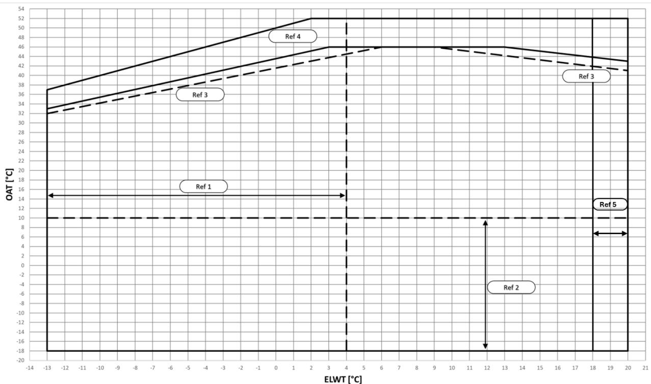
Fig. 3 – EWYTx0B-S Limitele Operationale ale Modului de Racire
