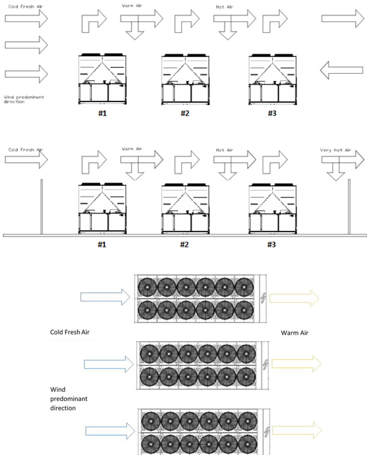
Fig. 12 – Instalarea mai multor răcitoare
