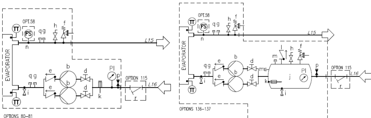
Obr. 17 – Hydraulická schéma dvojitého čerpadla (EWYTx5B) (možnosť 80 – 81/136 – 137) (max. prevádzkový tlak 6 barov)
