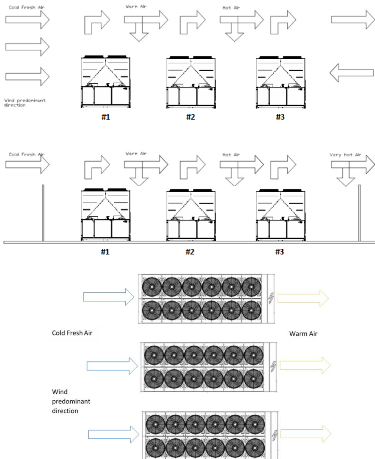
Obr. 12 – Inštalácia viacerých jednotiek (režim chladenia)
