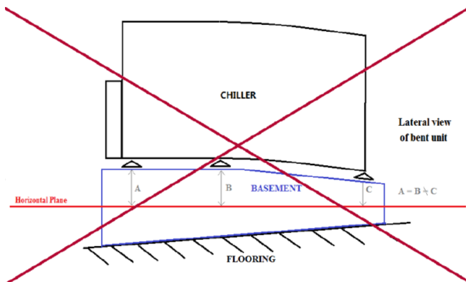
Obr. 10 – Vyrovnanie jednotky
