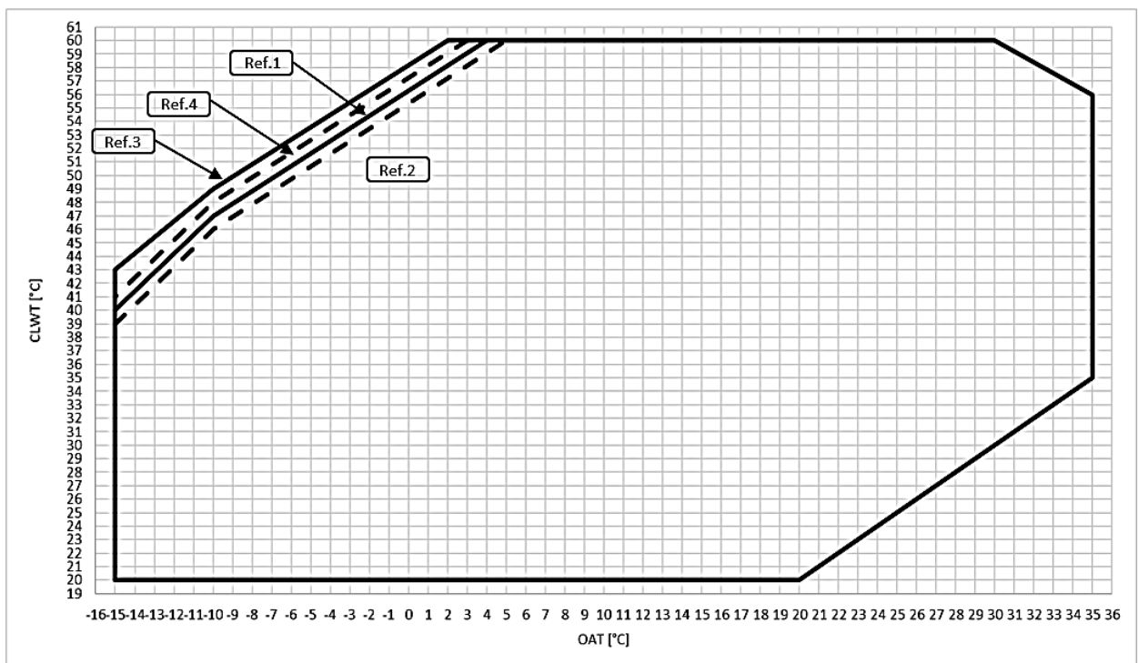
Obr. 7 – Prevádzkové limity režimu ohrevu EWYT~B-S – OP.204
