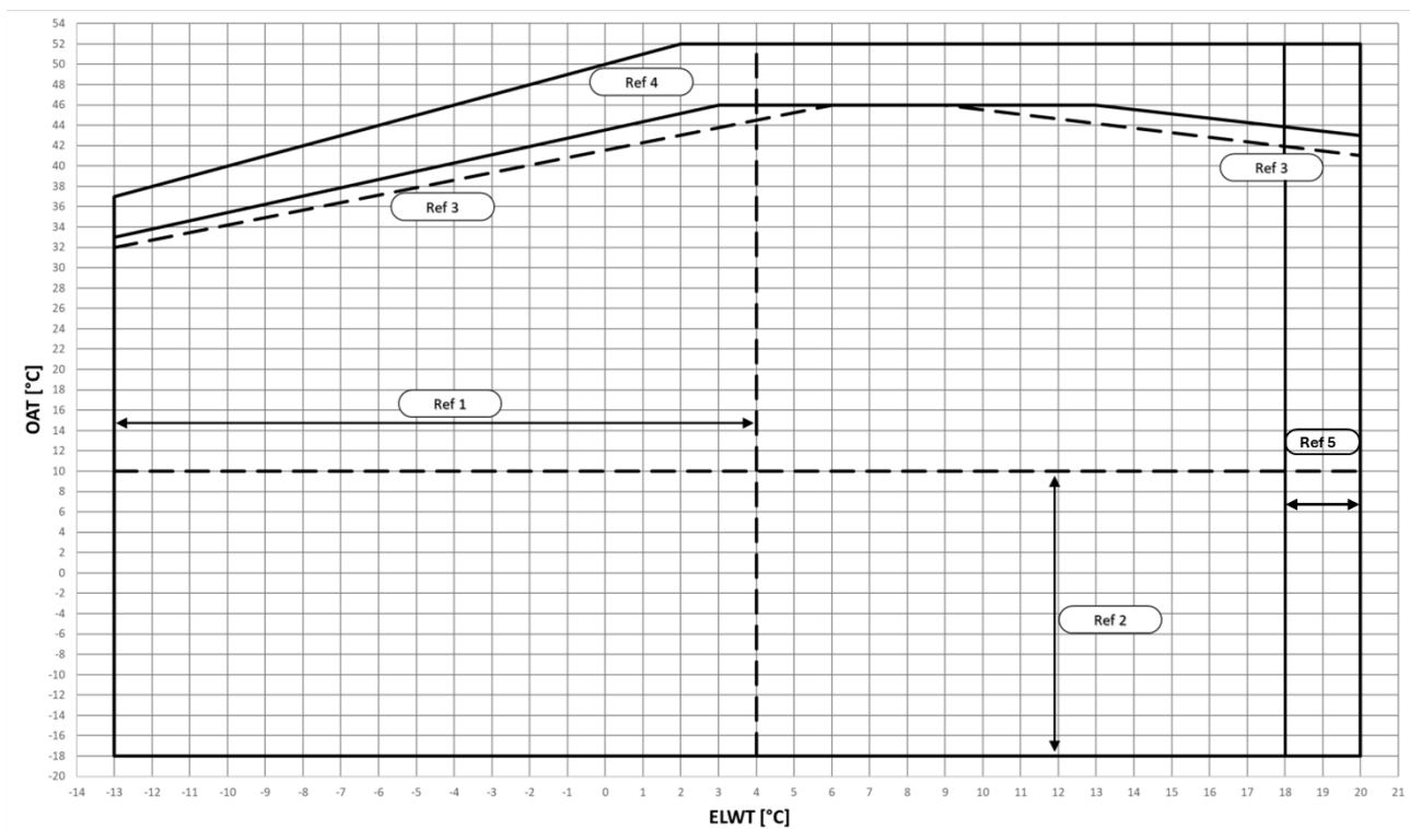
Obr. 3 – Prevádzkové limity režimu chladenia EWYTx0B-S
