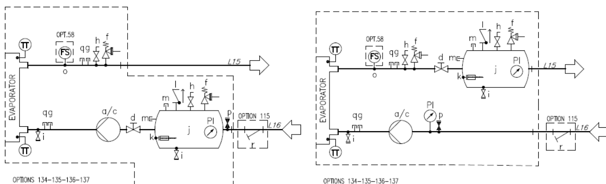
Fig.16– Diagrami hidraulik për pompën e vetme / pompën e dyfishtë me rezervuar (EWYTx5B) (opt. 134-135) (presioni maksimal i funksionimit 6 bar)
