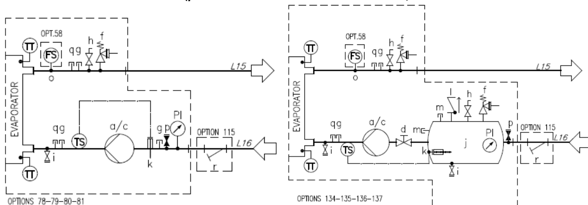
Fig.17– Diagrami hidraulik për pompën e dyfishtë (EWYTx5B) (opt. 80-81/136-137) (presioni maksimal i funksionimit 6 bar)
