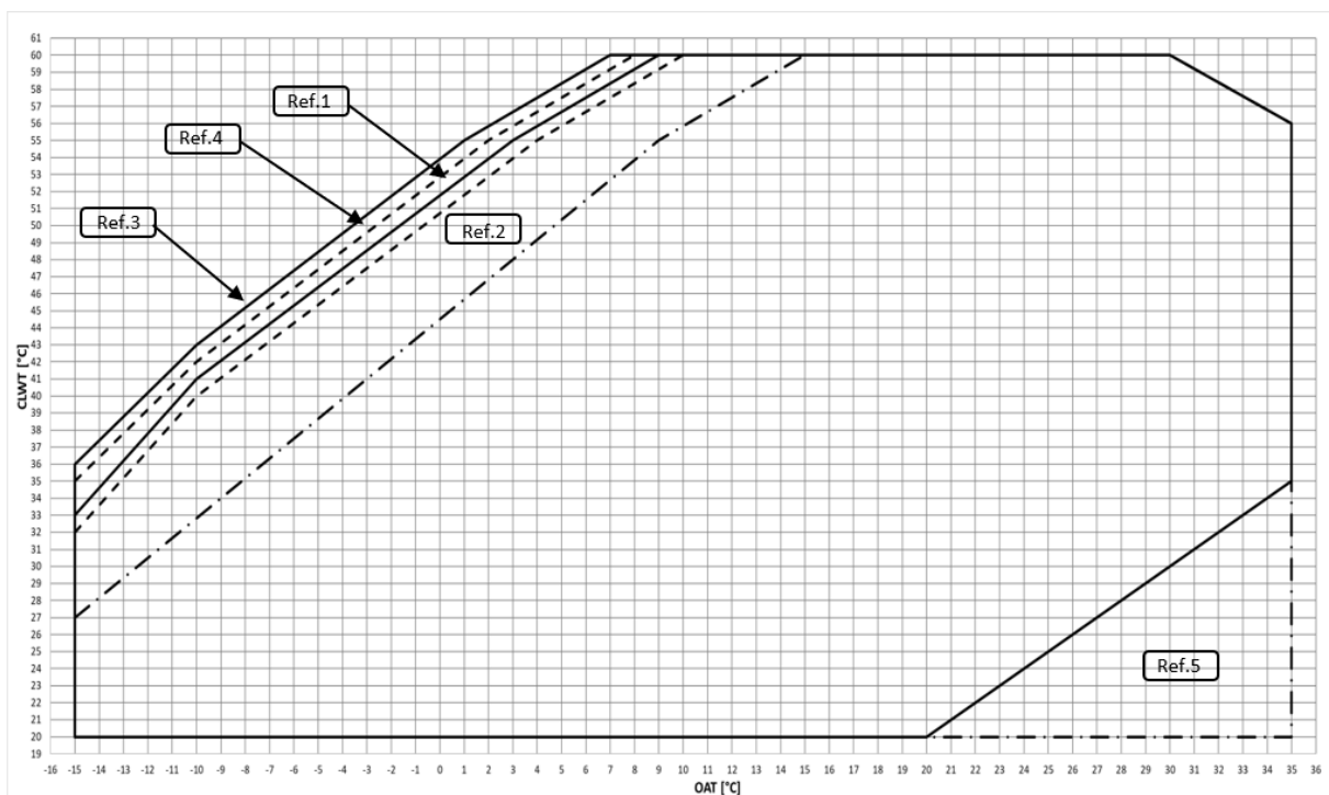
Fig.5- Kufijtë e funksionimit të modalitetit të ngrohjes EWYT~BS
