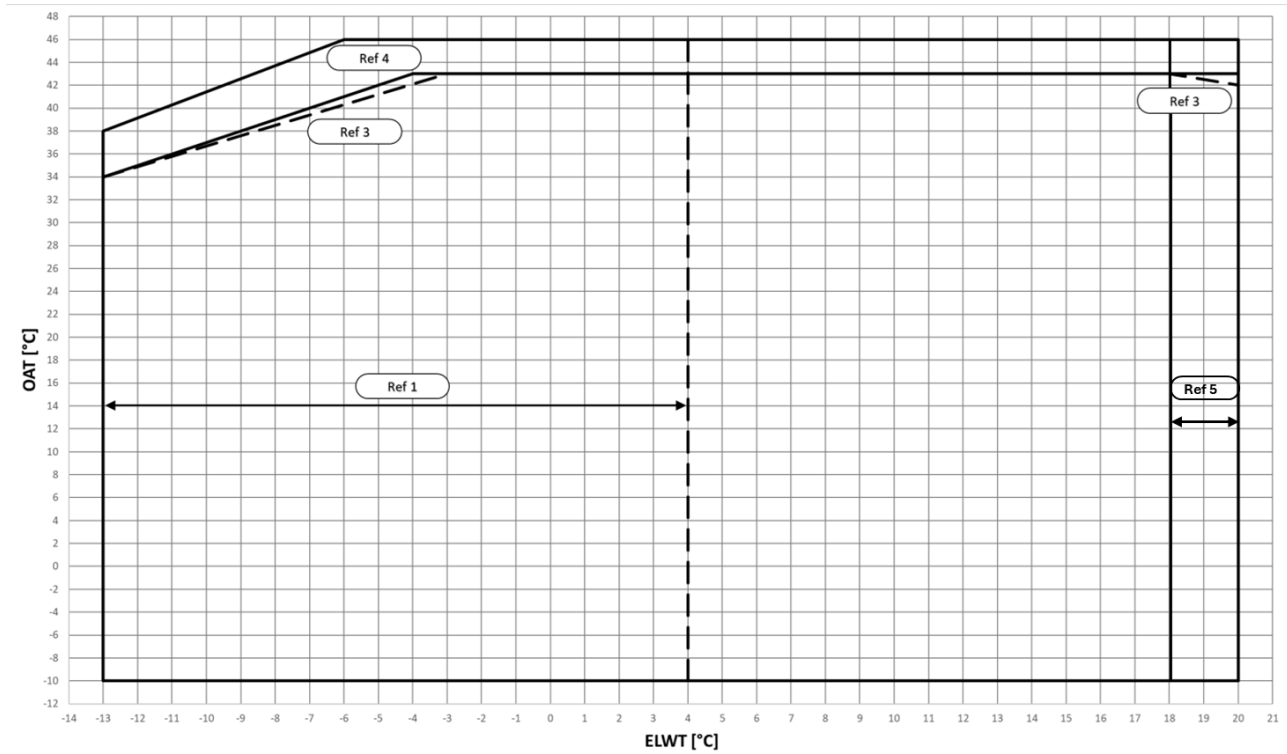
Fig.2- Kufijtë e funksionimit të modalitetit të ftohjes EWYTx5B-X
