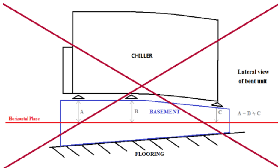
Fik.10- Nivelimi i njësisë
