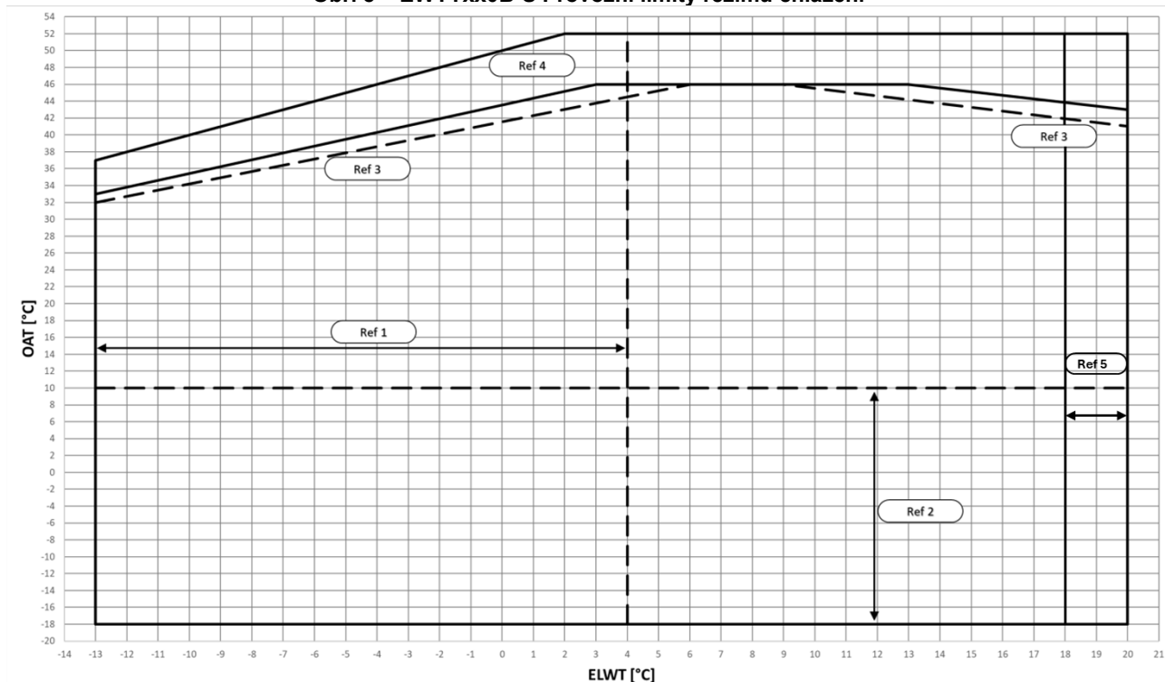
Obr. 9 – EWYTx0B-X Provozní limity režimu chlazení
