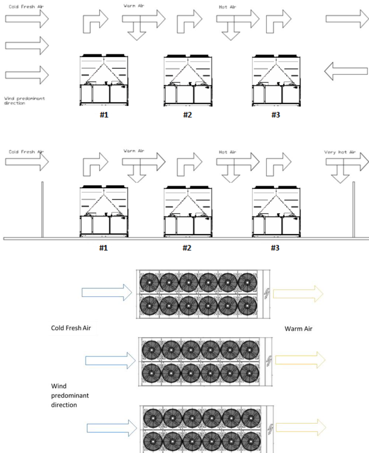
Obr. 17 – Instalace s několika jednotkami (režim chlazení)
