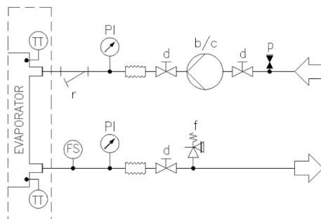
Obr. 21 – Hydraulické schéma pro jednotné čerpadlo / dvojité čerpadlo (EWYTx5B) (vol. 78-79) (max. provozní tlak 6 bar)
