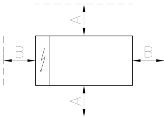
Obr. 16 – Požadavky minimálního prostoru
