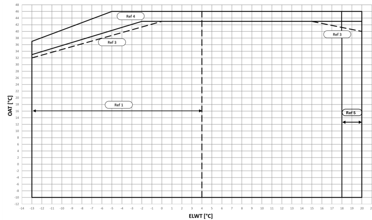
Obr. 6 – EWYTx5B-S Provozní limity režimu chlazení
