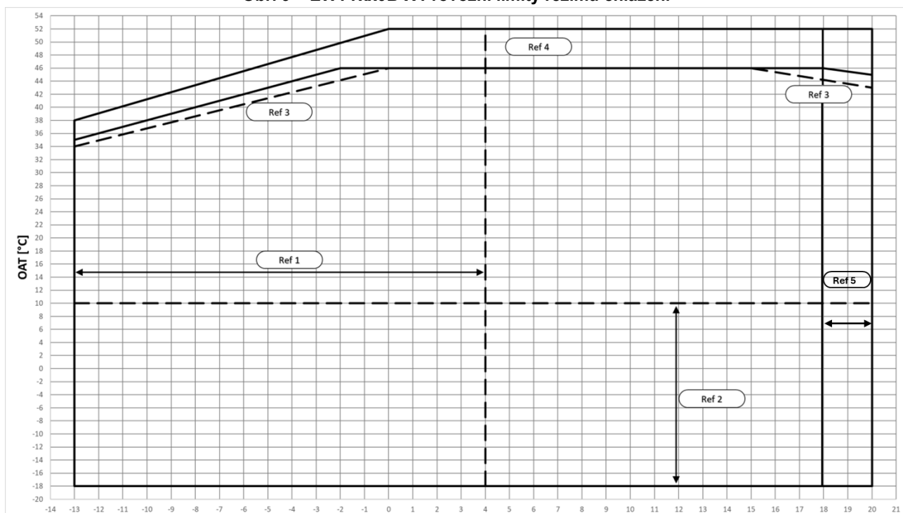
Obr. 9 – EWYTx0B-X Provozní limity režimu chlazení
