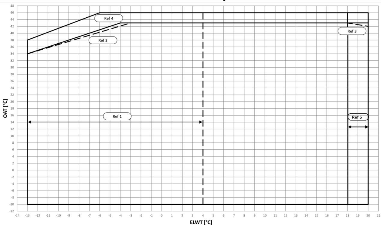
Obr. 7 – EWYTxx5B-X Provozní limity režimu chlazení
