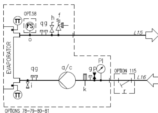
Obr. 22 – Hydraulické schéma pro jednotné čerpadlo / dvojité čerpadlo s nádrží (EWYTx5B) (vol. 134-135) (max. provozní tlak 6 bar)
