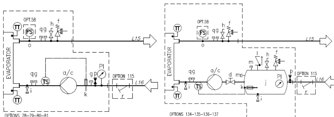
Obr. 24 – Hydraulické schéma pro jednotné čerpadlo / dvojité čerpadlo (vol. 78-79-80-81/134-135-136-137) (max. provozní tlak 6 bar)
