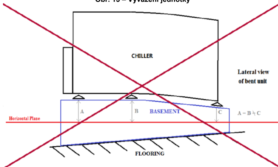
Obr. 15 – Vyvážení jednotky
