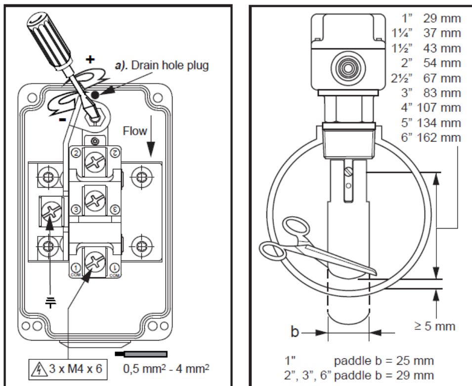
Obr. 19– Nastavení průtokového spínače (model F61TB-9100 – Johnson Controls)
