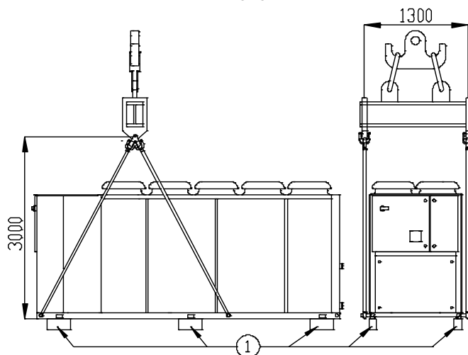
Obr. 14 – Pokyny pro zdvihání
