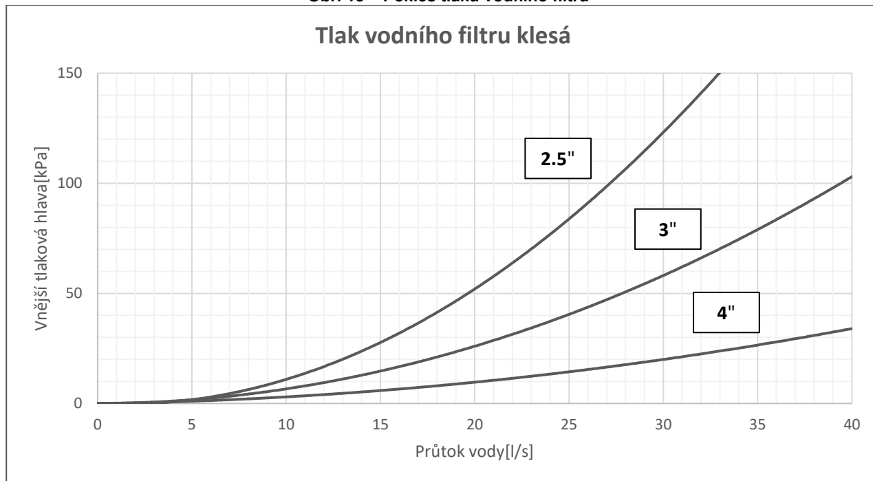
Obr. 18 – Pokles tlaku vodního filtru
