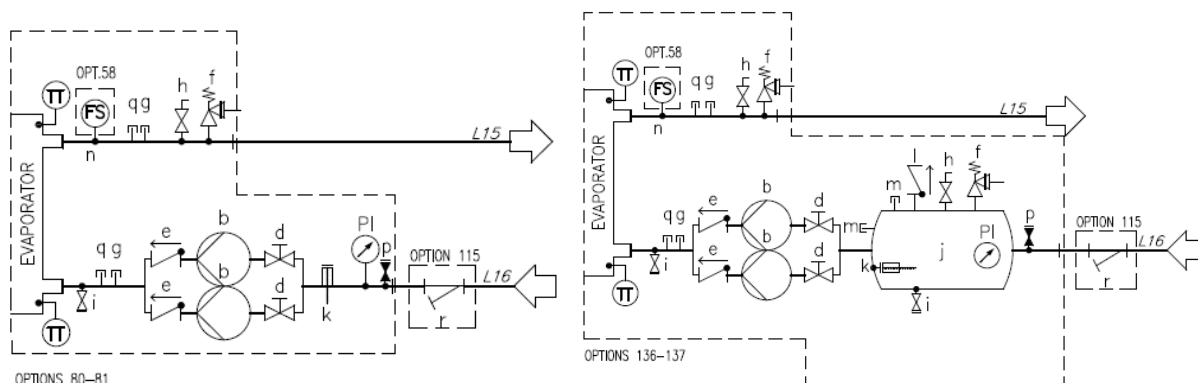
Obr. 23 – Hydraulické schéma pro dvojité čerpadlo (EWYTx5B) (vol. 80-81/136-137) (max. provozní tlak 6 bar)
