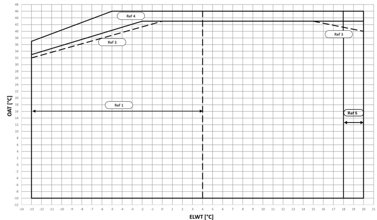
Abb. 6 – EWYTxx5B-S Betriebsgrenzen im Kühlbetrieb
