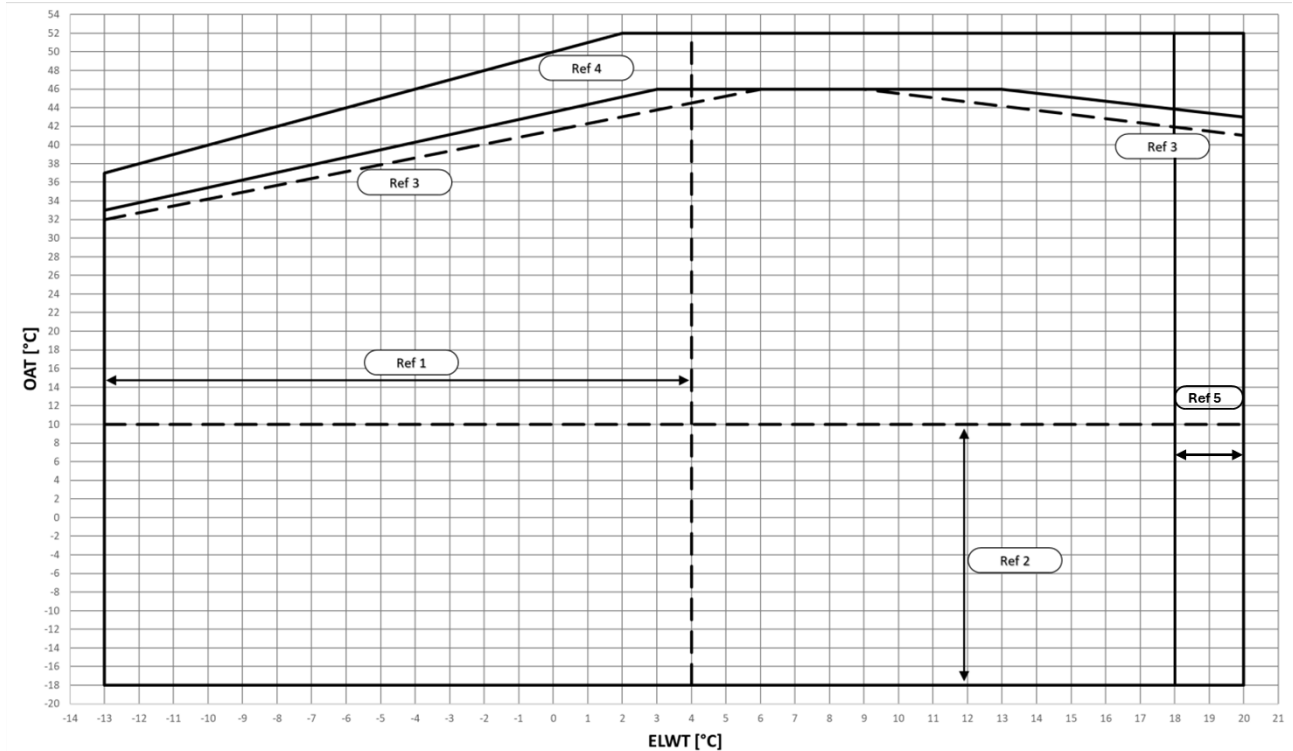
Abb. 9 – EWYTx0B-X Betriebsgrenzen im Kühlbetrieb
