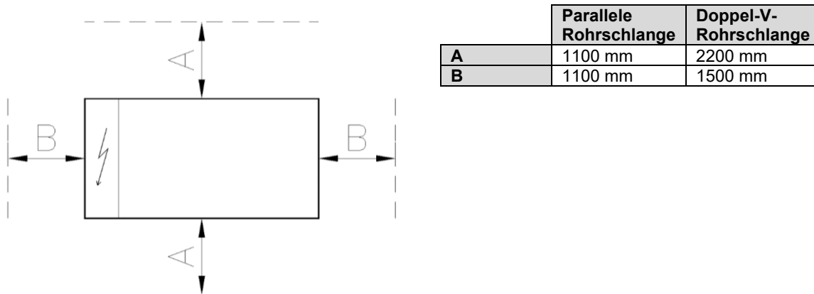
Abb. 16 – Mindestabstände
