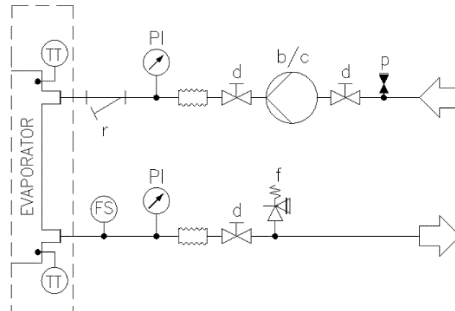
Abb. 21 – Hydraulikschema für Einzel- / Doppelpumpengerät (EWYTx5B) (Opt. 78-79) (max. Betriebsdruck 6 bar)
