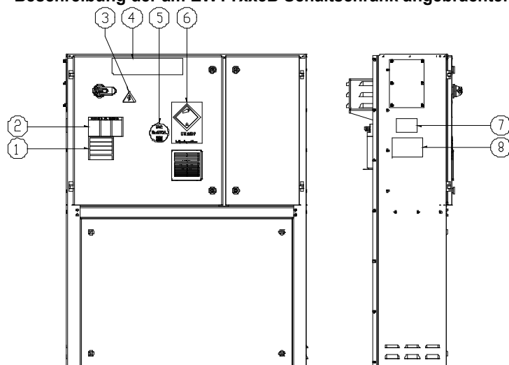
Abb. 4 – Beschreibung der am EWYTx5B Schaltschrank angebrachten Aufkleber
