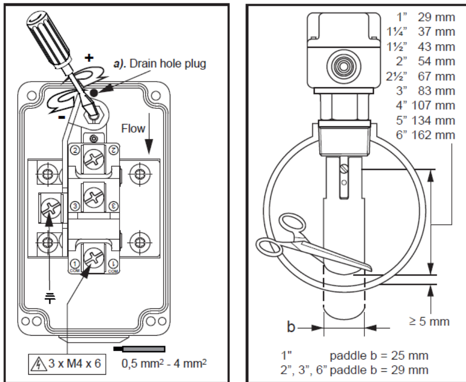
Abb. 19 – Einstellung des Strömungswächters (Modell F61TB-9100 – Johnson Controls)
