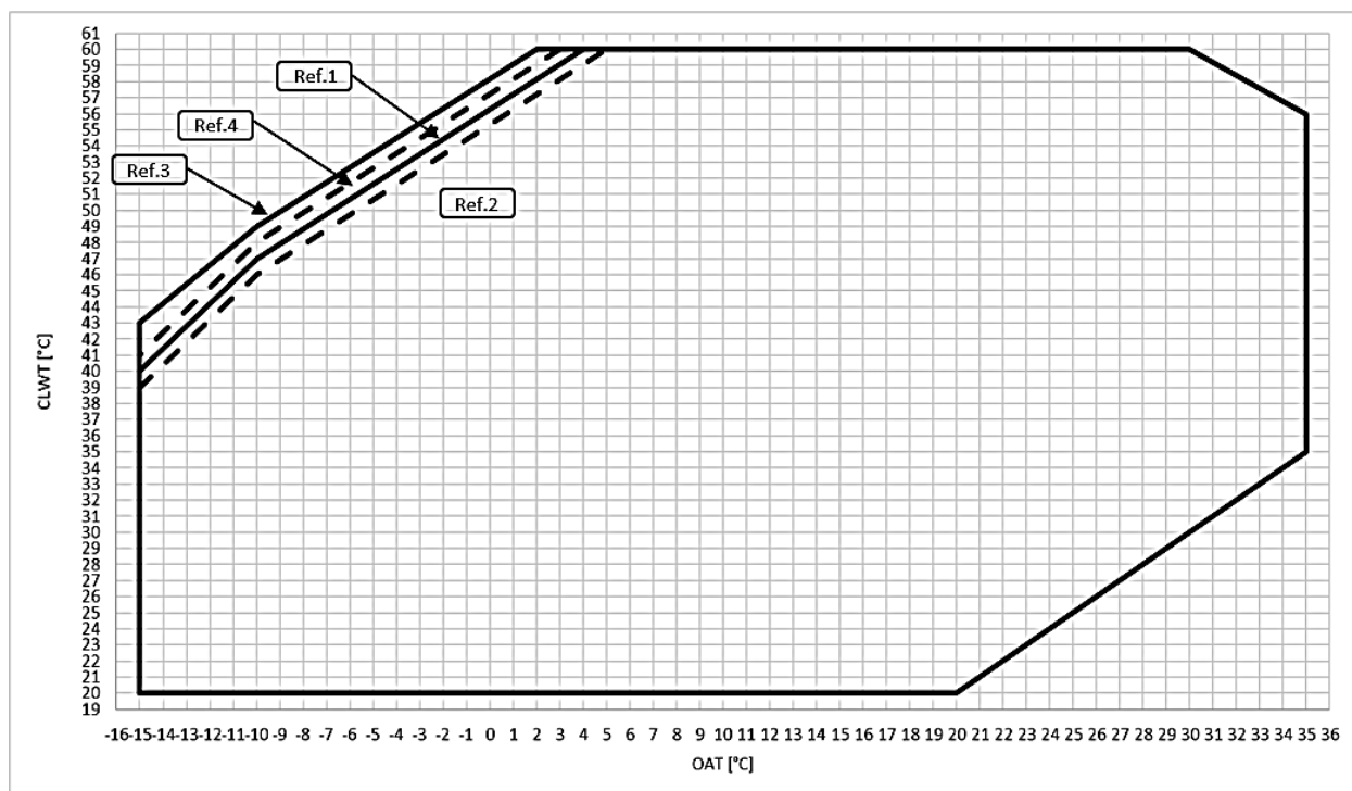
Abb. 13 – EWYT~B-X – OP.204 Betriebsgrenzen im Heizbetrieb
