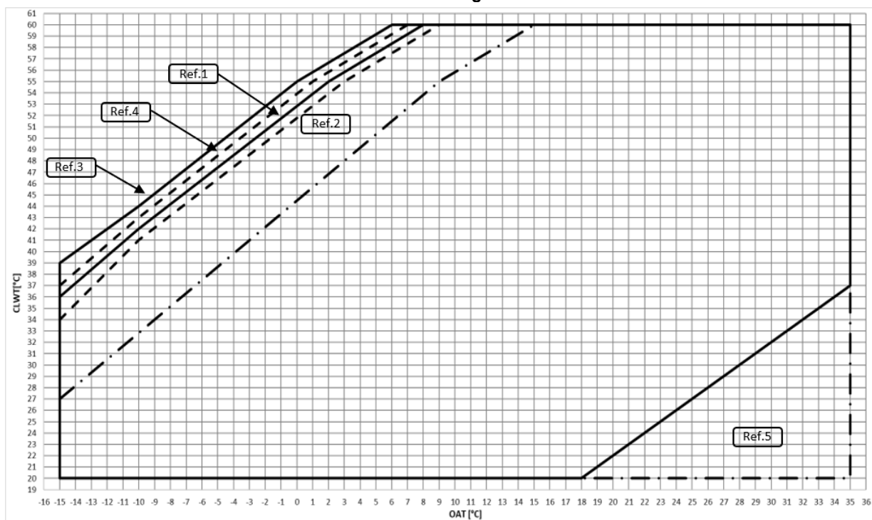
Abb. 11 – EWYT~B-X Betriebsgrenzen im Heizbetrieb
