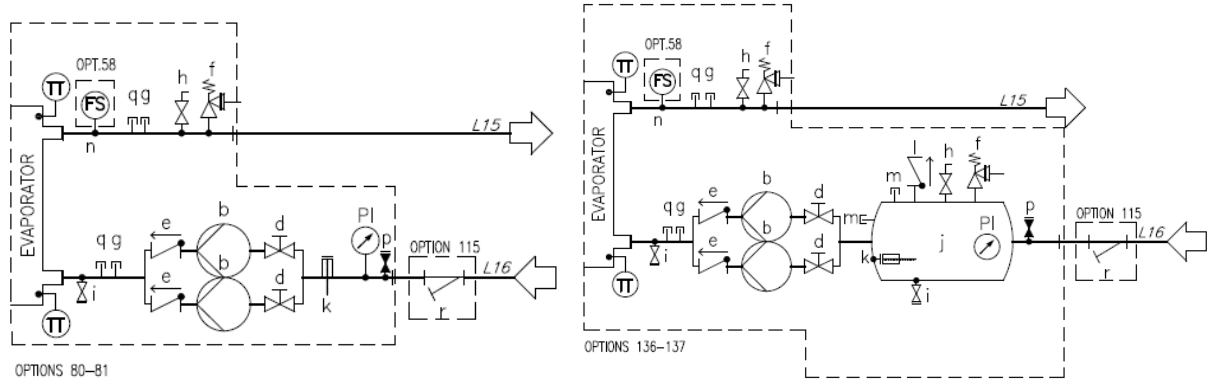
Abb. 24 – Hydraulikschema für Einzel- / Doppelpumpengerät (Opt. 78-79-80-81/134-135-136-137) (max. Betriebsdruck 6 bar)
