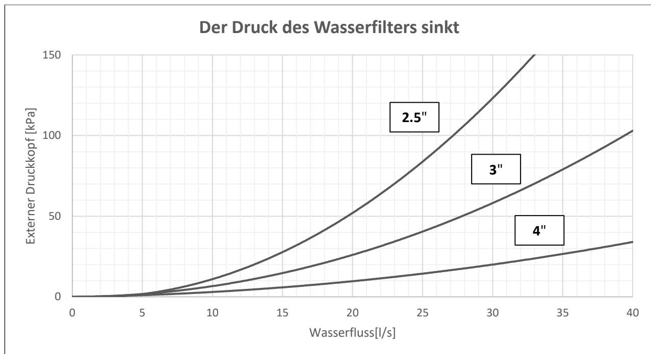
Abb. 18 – Druckabfall des Wasserfilters
