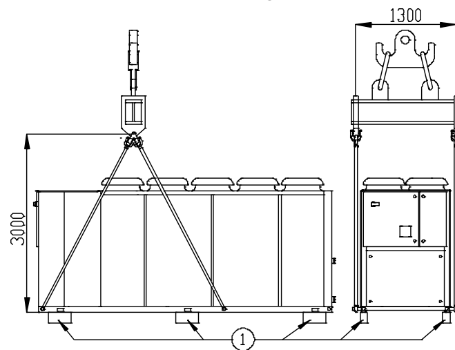
Abb. 14 – Anweisungen zum Heben
