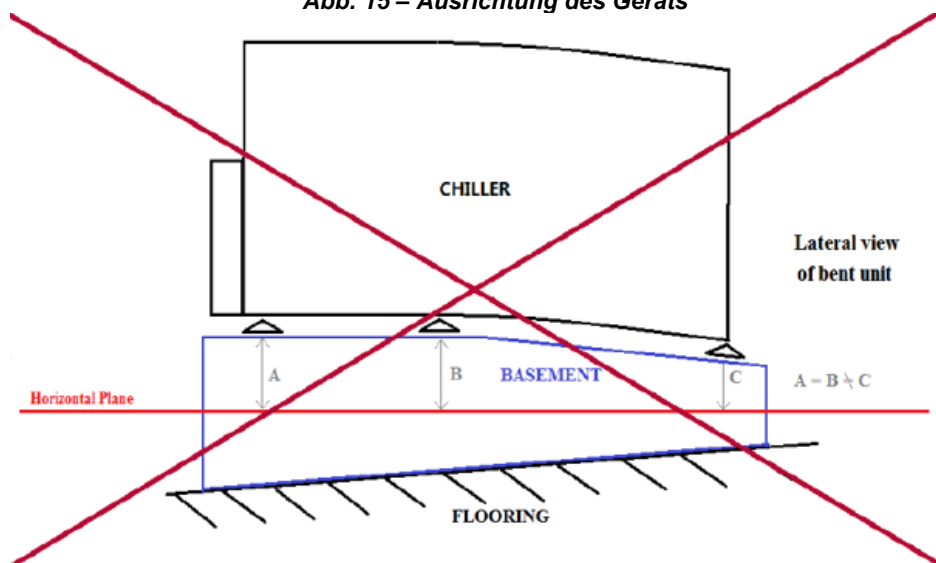
Abb. 15 – Ausrichtung des Geräts
