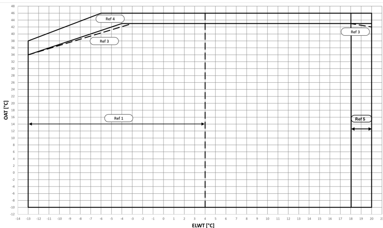
Abb. 7 – EWYTxx5B-X Betriebsgrenzen im Kühlbetrieb
