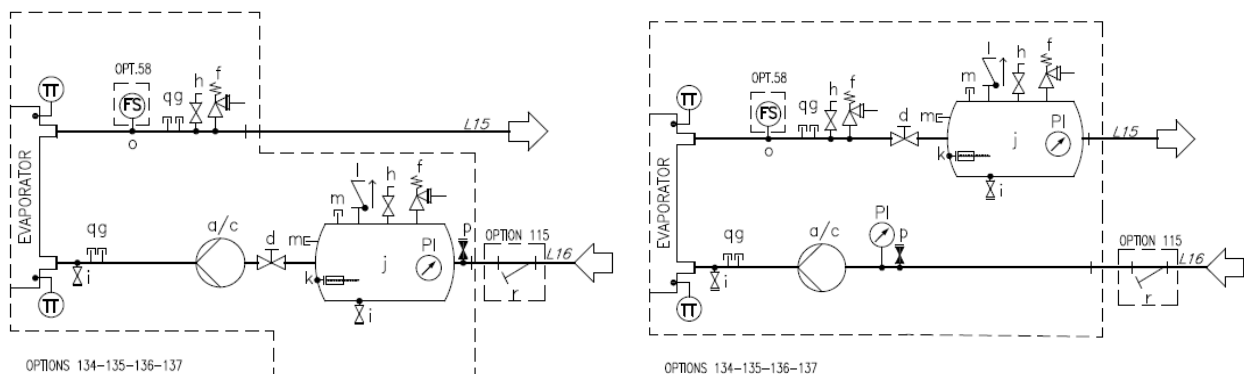
Abb. 22 – Hydraulikschema für Einzel- / Doppelpumpengerät mit Tank (EWYTx5B) (Opt. 134-135) (max. Betriebsdruck 6 bar)
