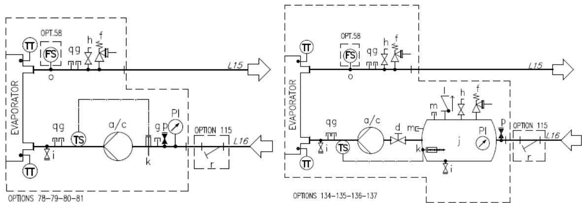
Abb. 24 – Hydraulikschema für Einzel- / Doppelpumpengerät (Opt. 78-79-80-81/134-135-136-137) (max. Betriebsdruck 6 bar)
