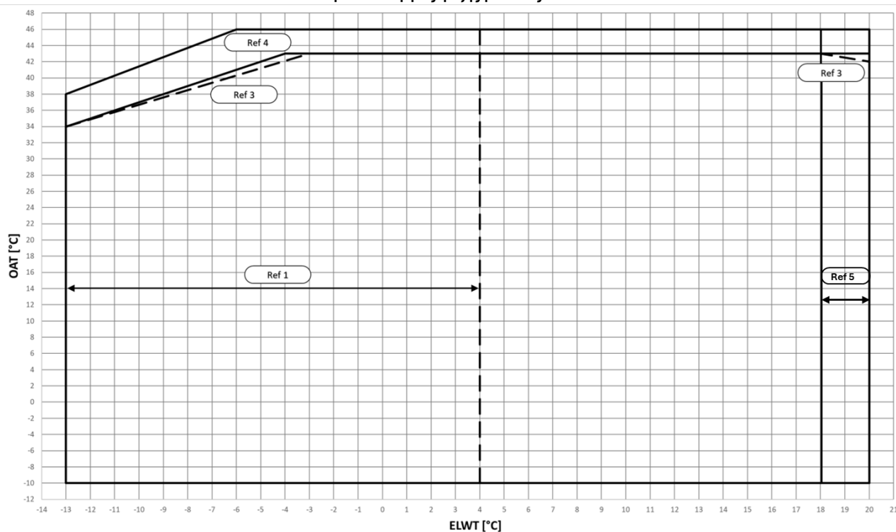
Εικ. 7 – Όρια λειτουργίας ψύξης μονάδας EWYTx5B-X
