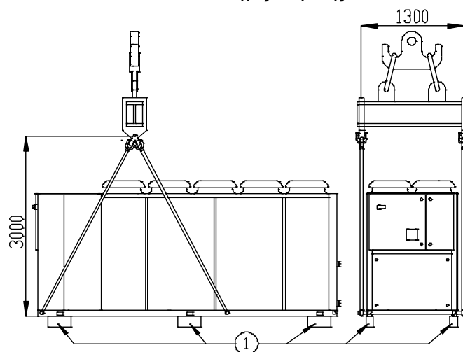
Εικ. 14 – Οδηγίες ανύψωσης
