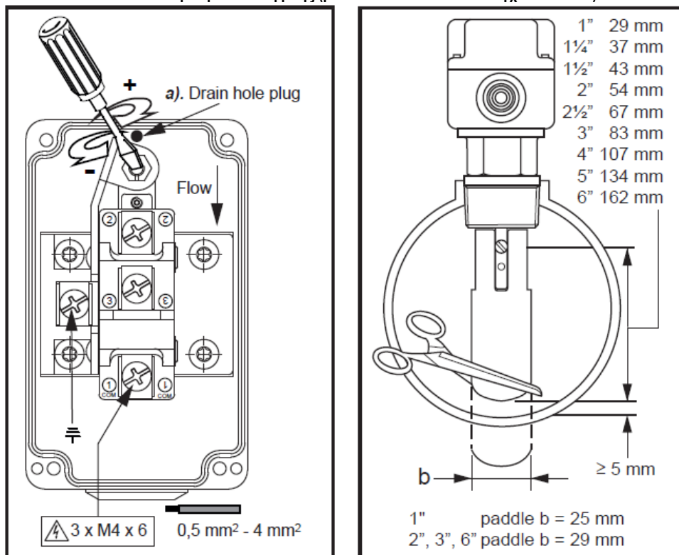
Εικ. 19 – Ρύθμιση διακόπτη ροής (μοντέλο F61TB-9100 – Έλεγχος Johnson)
