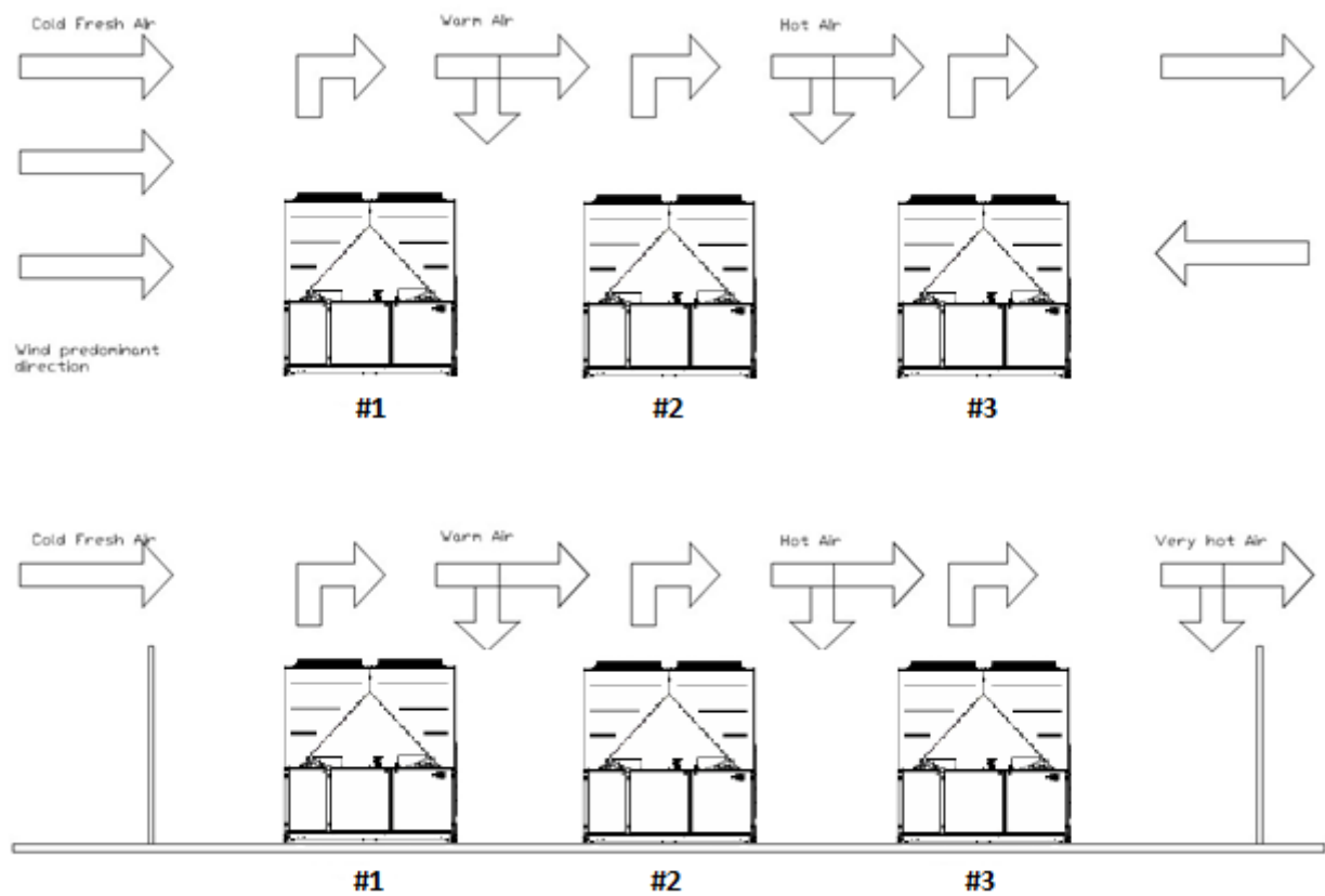
Εικ. 17 – Εγκατάσταση πολλών μονάδων (λειτουργία ψύξης)
