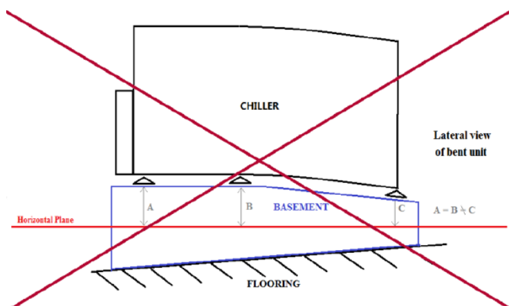
Εικ. 15 – Οριζόντιωση μονάδας
