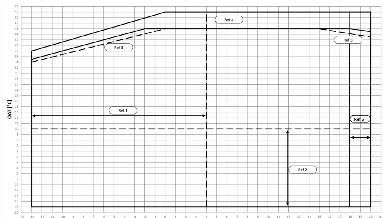
Εικ. 9 – Όρια λειτουργίας ψύξης μονάδας EWYTxx0B-X
