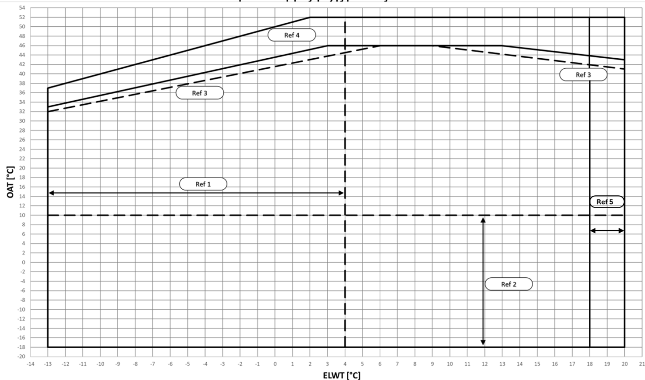
Εικ. 8 – Όρια λειτουργίας ψύξης μονάδας EWYTx0B-S
