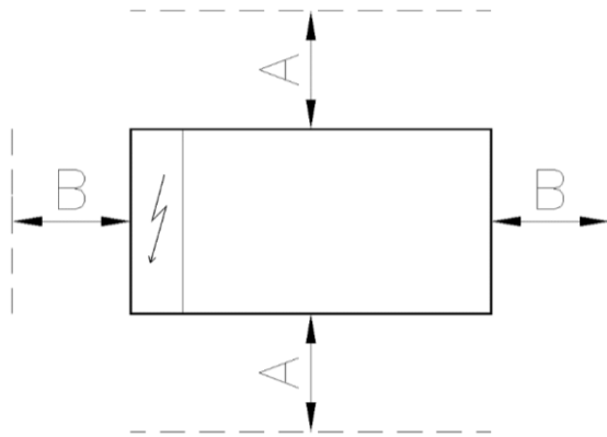
Εικ. 16 – Ελάχιστες απαιτήσεις χώρου
