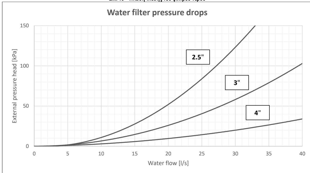
Εικ. 18 – Πτώση πίεσης του φίλτρου νερού
