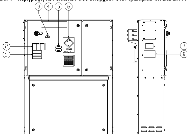
Εικ. 4 – Περιγραφή των ετικετών που υπάρχουν στον ηλεκτρικό πίνακα EWYTxx5B
