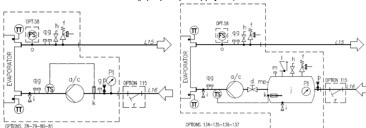
Εικ. 24 – Διάγραμμα υδραυλικού κυκλώματος για μονή αντλία / διπλή αντλία (επιλογές 78-79-80-81/134-135-136-137) (μέγιστη πίεση λειτουργίας 6 bar)
