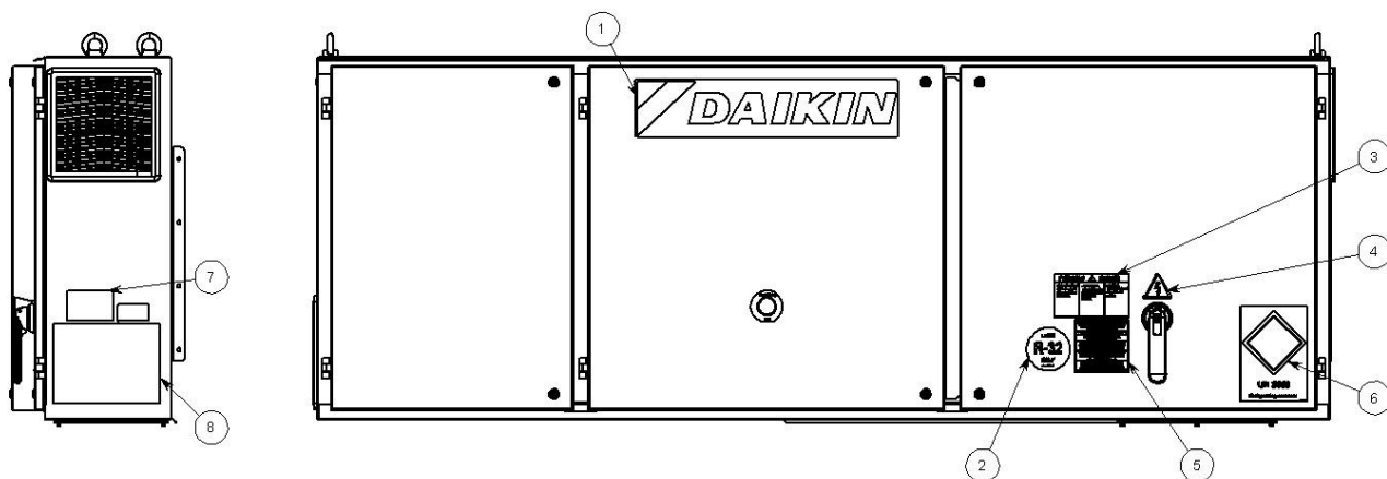
Εικ. 5 – Περιγραφή των ετικετών που υπάρχουν στον ηλεκτρικό πίνακα EWYTxx0B
