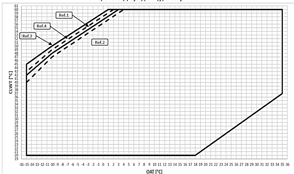
Εικ. 13 – Όρια λειτουργίας θέρμανσης μονάδας EWYT~B-X – OP.204
