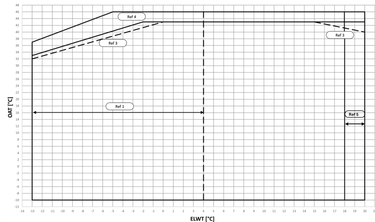
Εικ. 6 – Όρια λειτουργίας ψύξης μονάδας EWYTx5B-S
