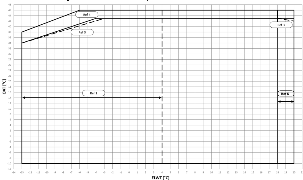
Fig. 7 – EWYTxx5B-X Límites Operativos del Modo de Enfriamiento
