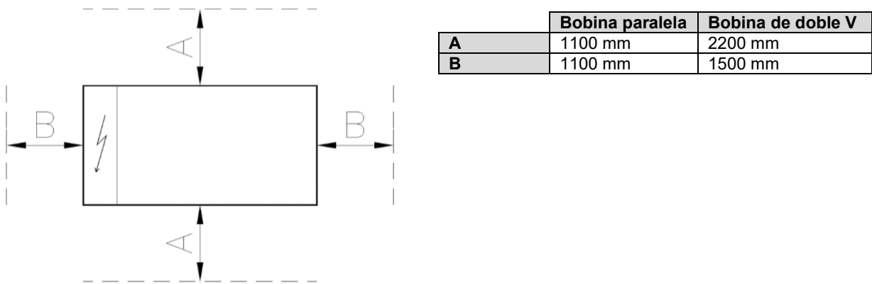
Fig. 16 – Requisitos de espacio mínimo
