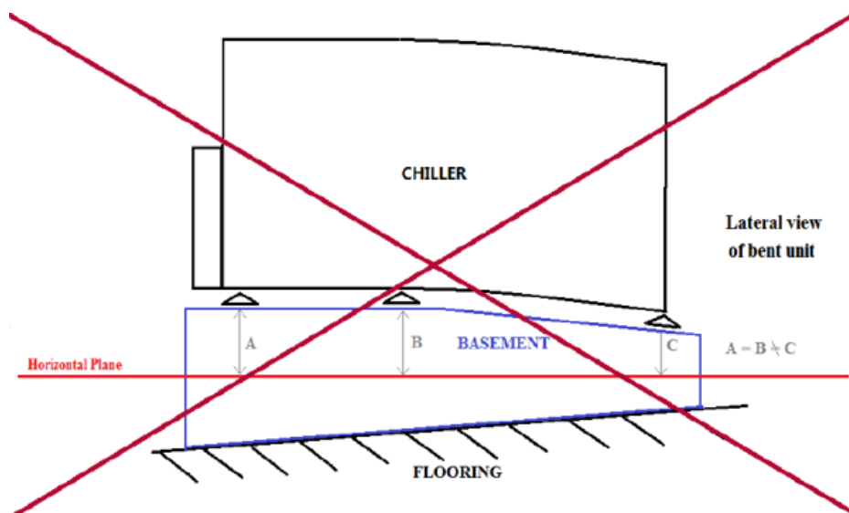
Fig. 15 – Nivelación de la unidad
