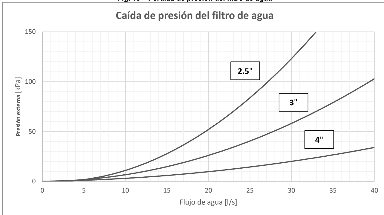
Fig. 18 – Pérdida de presión del filtro de agua
