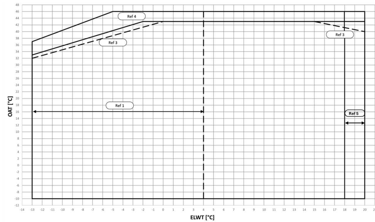
Fig. 6 – EWYTx5B-S Límites Operativos del Modo de Enfriamiento
