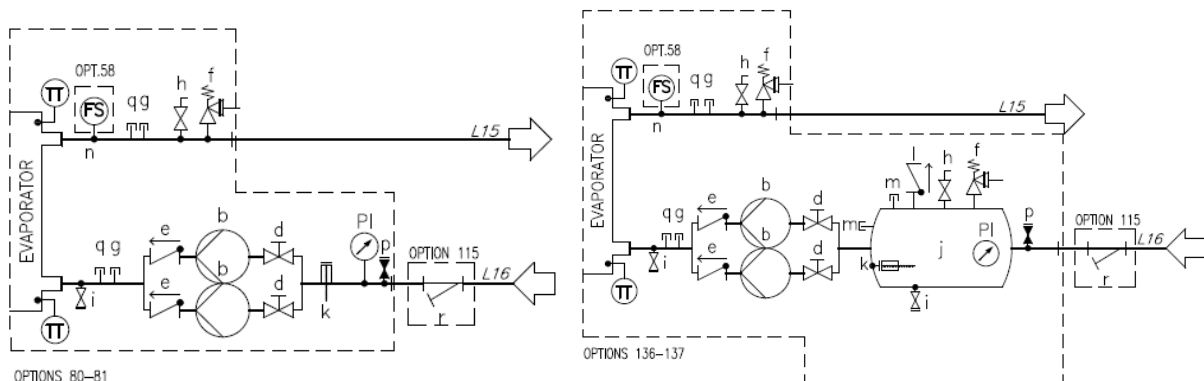
Fig. 23 – Diagrama hidráulico para bomba doble (EWYTx5B) (opc. 80-81/136-137) (presión operativa máxima 6 bares)
