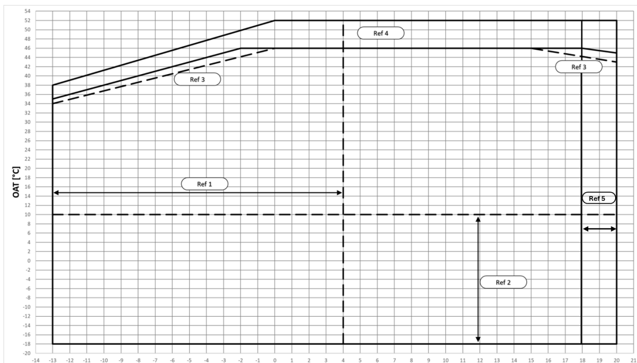
Fig. 9 – EWYTx0B-X Límites Operativos del Modo de Enfriamiento
