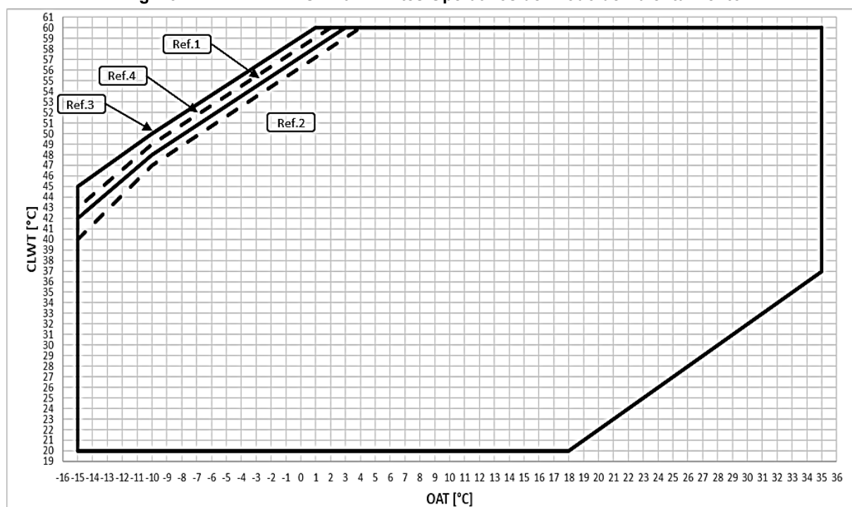
Fig. 13 – EWYT~B-X – OP.204 Límites Operativos del Modo de Calentamiento
