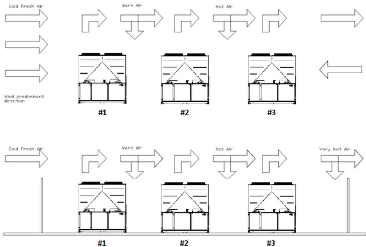
Fig. 17 – Instalación de múltiples unidades (modo de enfriamiento)
