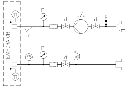
Fig. 21 – Diagrama hidráulico para bomba única / dos bombas (EWYTx5B) (opc. 78-79) (presión operativa máxima 6 bares)
