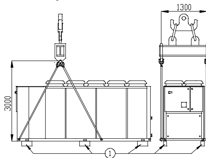
Fig. 14 – Instrucciones de elevación
