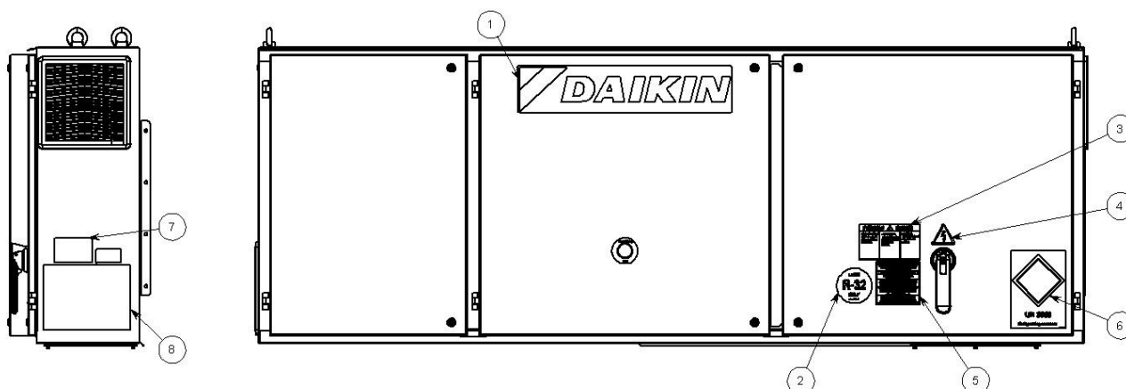
Fig. 5 – Descripción de las etiquetas fijadas al panel eléctrico EWYTxx0B
