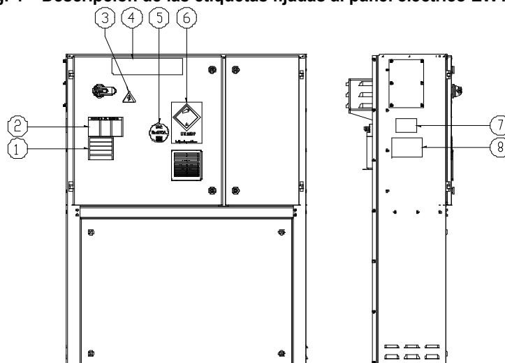
Fig. 4 – Descripción de las etiquetas fijadas al panel eléctrico EWYTxx5B
