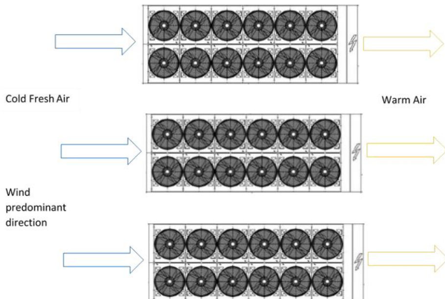
Fig. 17 – Instalación de múltiples unidades (modo de enfriamiento)
