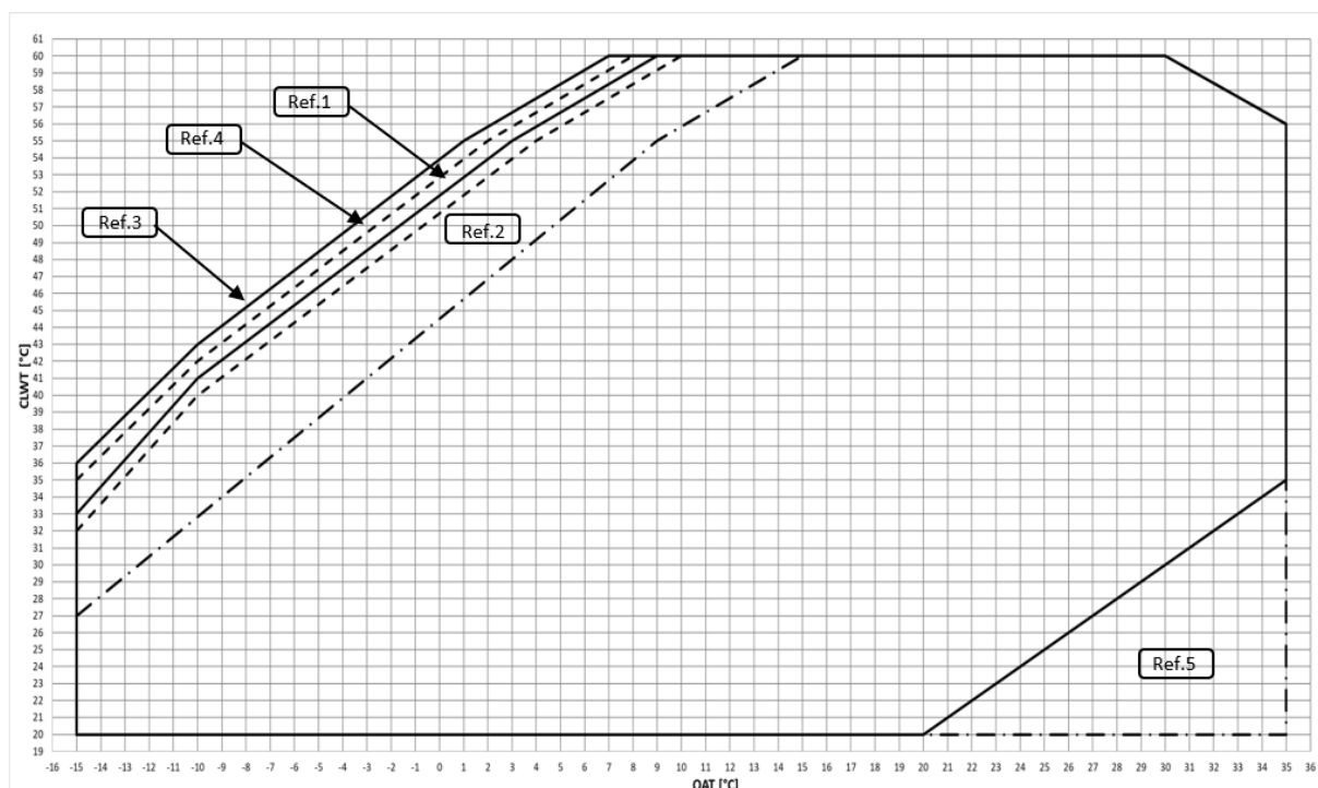
Fig. 11 – EWYT~B-X Límites Operativos del Modo de Calentamiento
