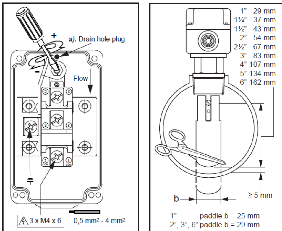
Fig. 19 – Ajuste del interruptor de flujo (modelo F61TB-9100 – Johnson Controls)
