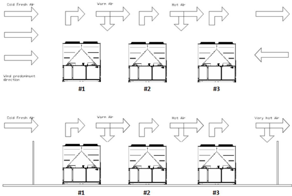
Fig. 17 - Installation d'unités multiples (mode refroidissement)
