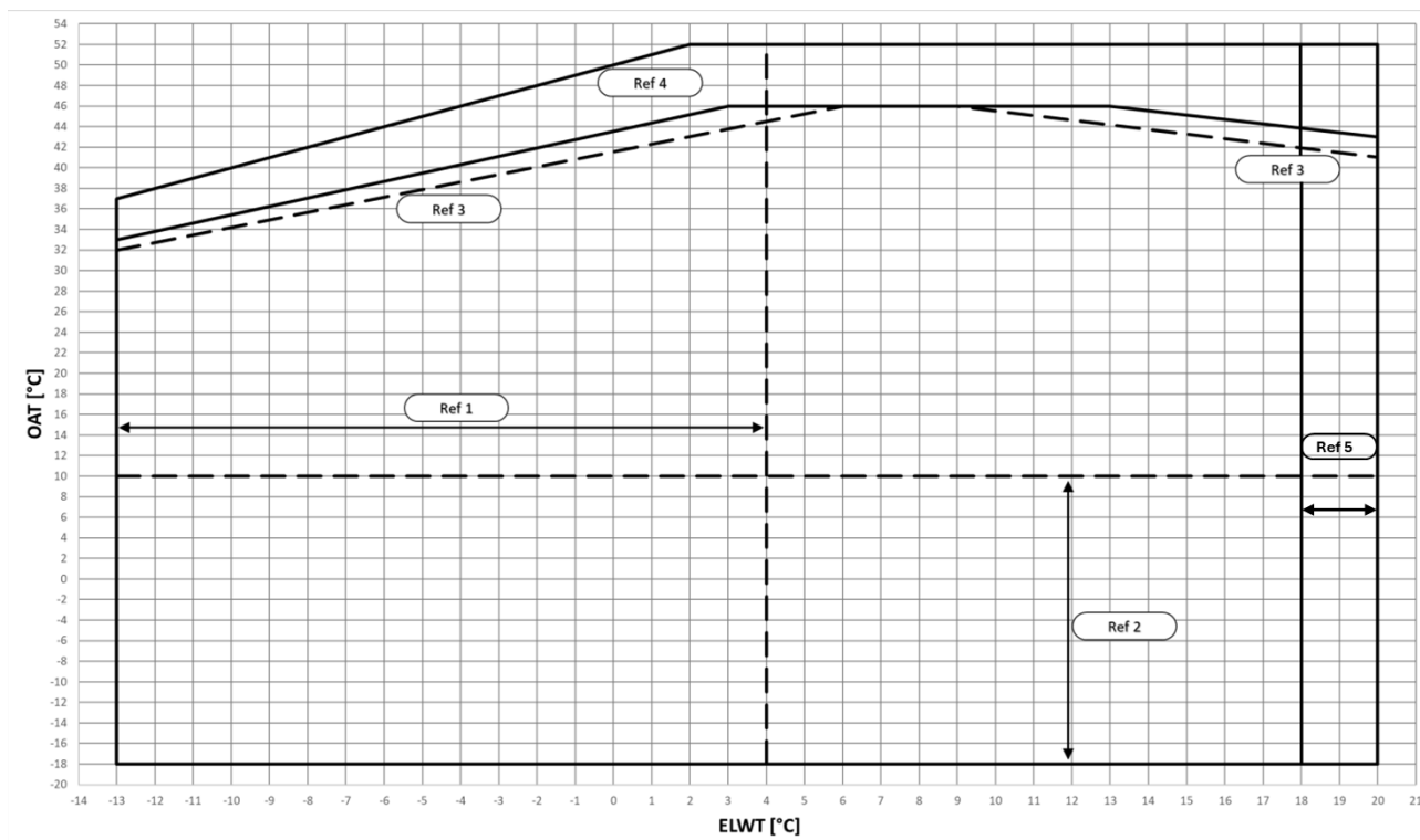
Fig. 9 - Limites opérationnelles du mode refroidissement EWYTx0B-X
