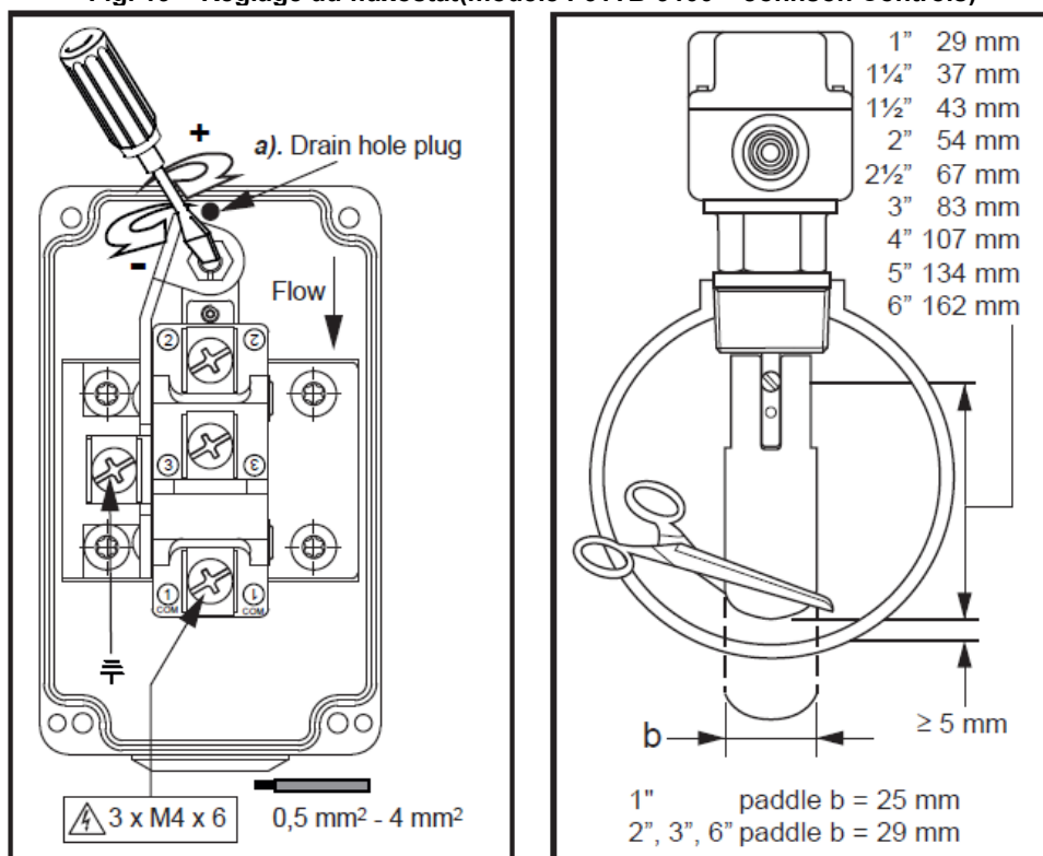
Fig. 19 – Réglage du fluxostat(modèle F61TB-9100 – Johnson Controls)
