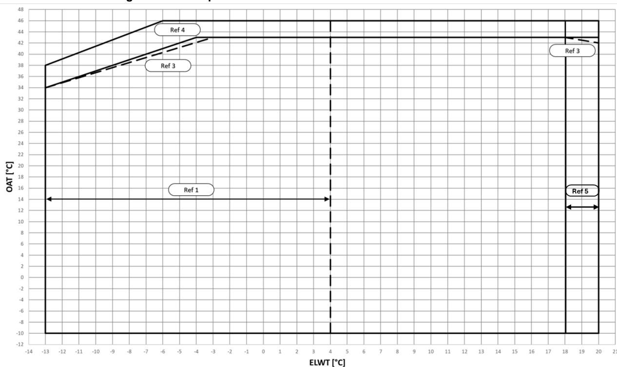
Fig. 7 - Limites opérationnelles du mode refroidissement EWYTx5B-X
