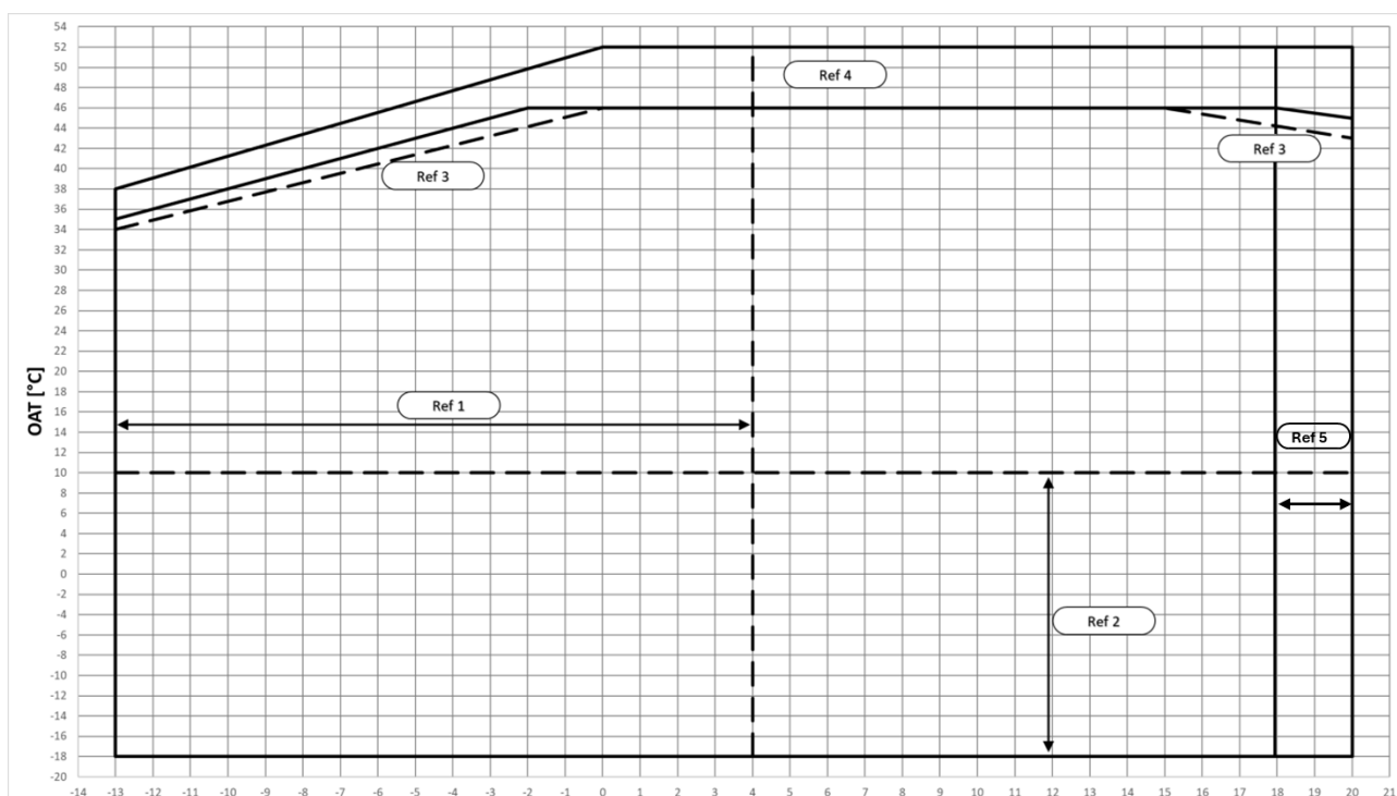
Fig. 9 - Limites opérationnelles du mode refroidissement EWYTx0B-X
