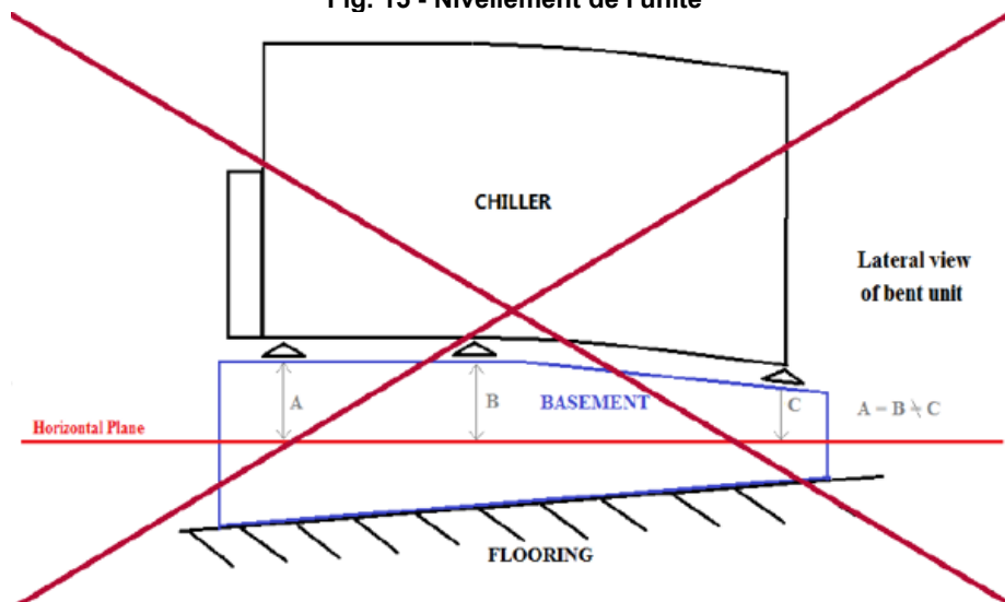
Fig. 15 - Nivellement de l'unité
