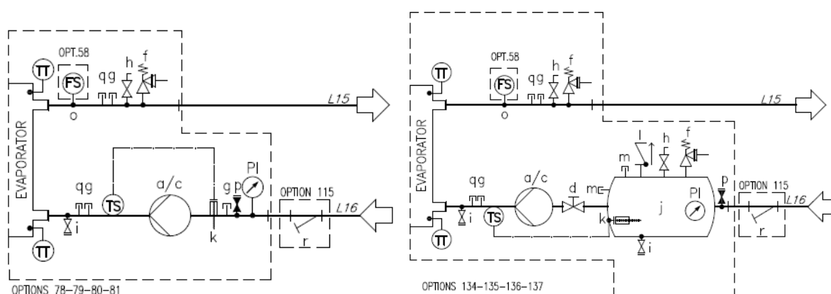
Fig. 24 - Schéma hydraulique pour pompe unique/pompes jumelles (opt. 78-79-80-81/134-135-136-137) (pression de service max. 6 bar)
