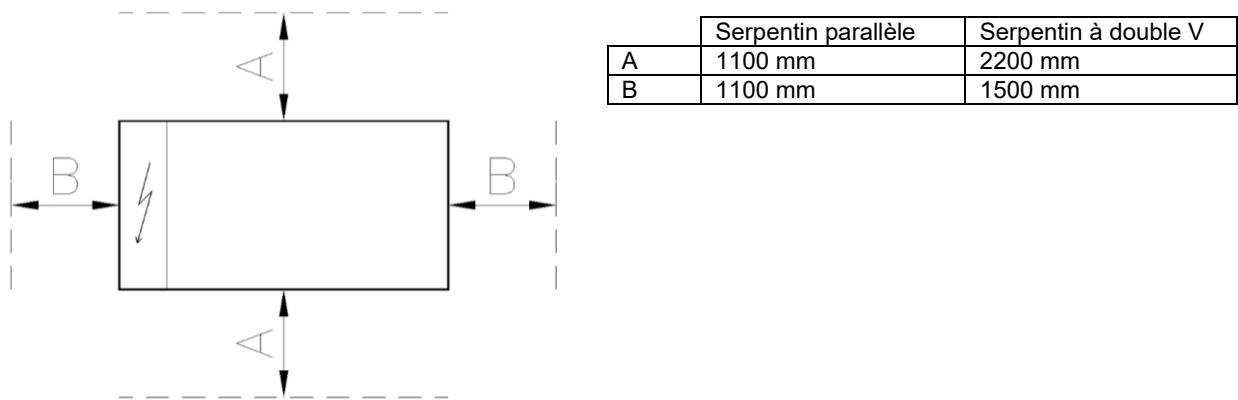
Fig. 16 - Encombrement minimal
