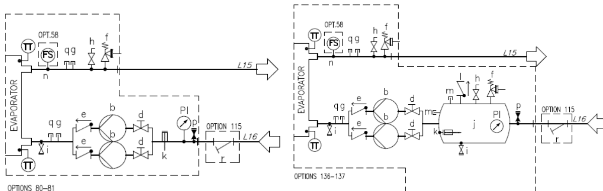
Fig. 24 - Schéma hydraulique pour pompe unique/pompes jumelles (opt. 78-79-80-81/134-135-136-137) (pression de service max. 6 bar)
