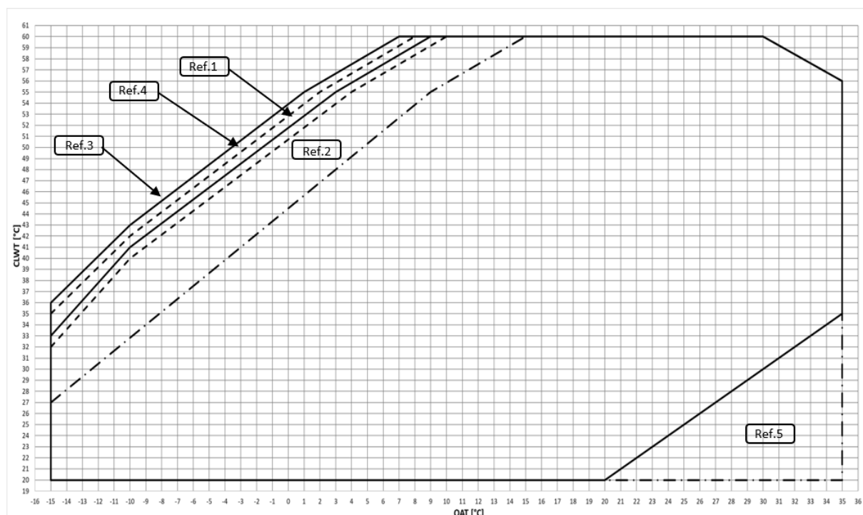
Fig. 11 - Limites opérationnelles du mode chauffage EWYT~B-X
