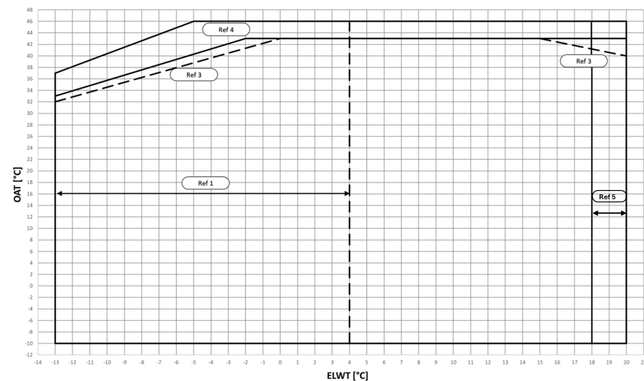
Fig. 6 - Limites opérationnelles du mode refroidissement EWYTx5B-S
