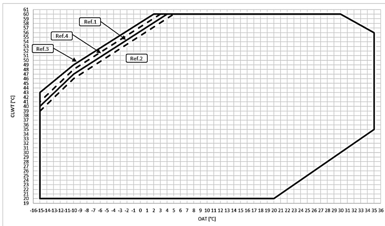
Fig. 13 - Limites opérationnelles du mode chauffage EWYT~B-X – OP.204
