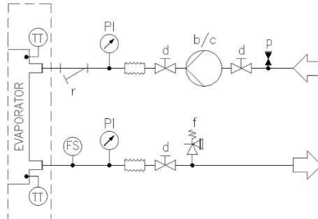
Fig. 21 - Schéma hydraulique pour pompe unique/pompes jumelles (EWYTx5B) (opt. 78-79) (pression de service max. 6 bar)
