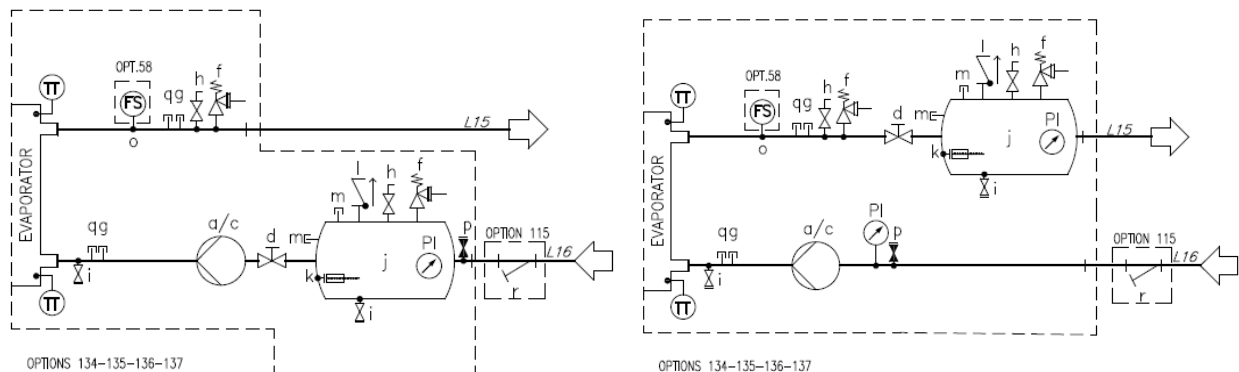
Fig. 22 - Schéma hydraulique pour pompe unique/pompes jumelles avec réservoir (EWYTx5B) (opt. 134-135) (pression de service max. 6 bar)
