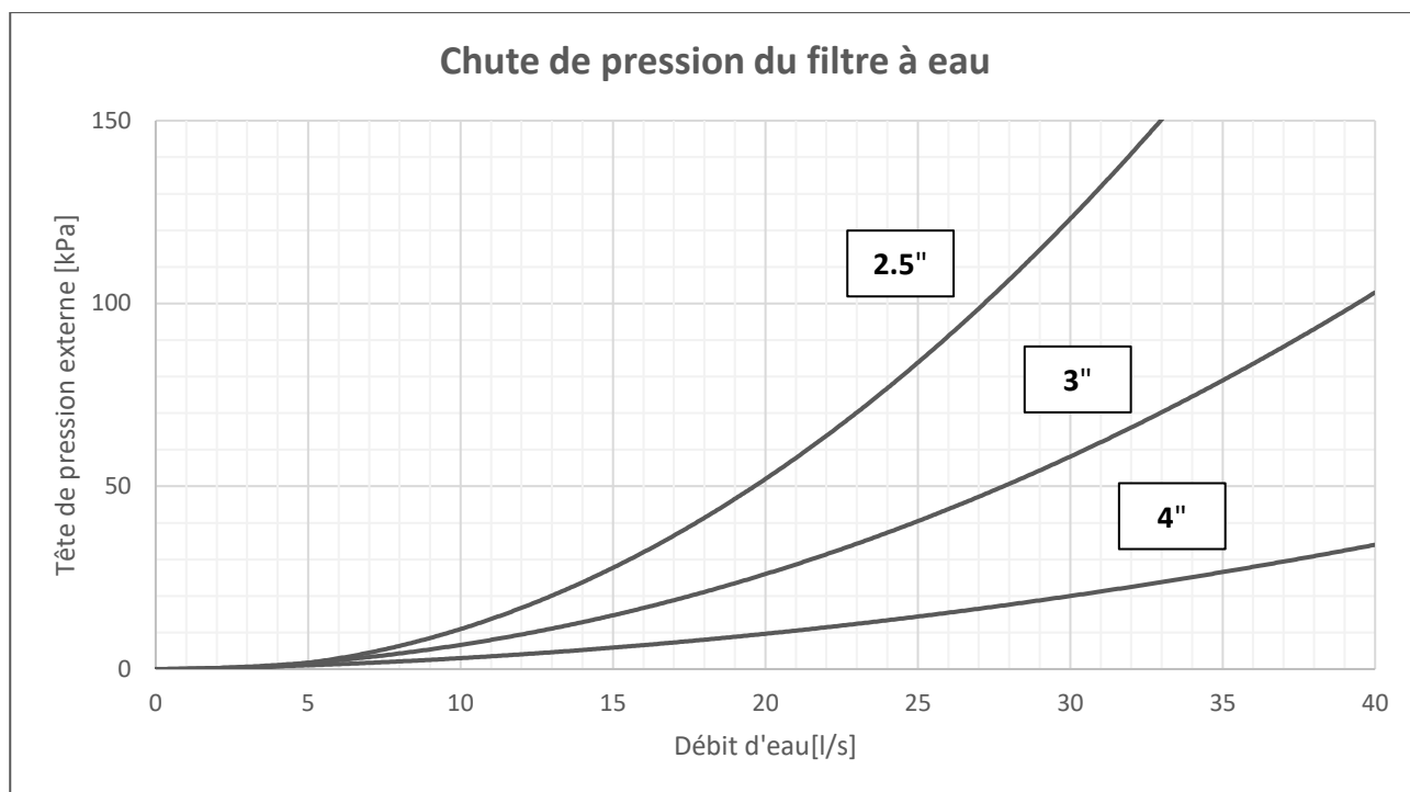
Fig. 18 - Perte de charge du filtre à eau
