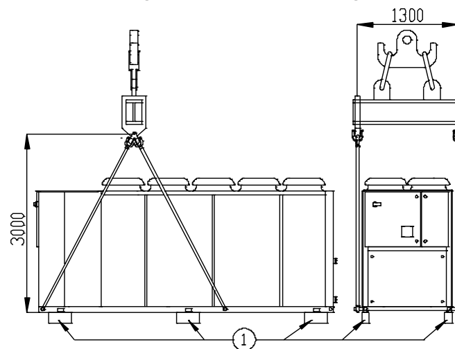
Fig. 14 - Instructions de levage
