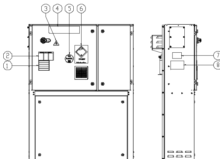
Fig. 4 - Description des étiquettes appliquées sur le tableau électrique EWYTxx5B
