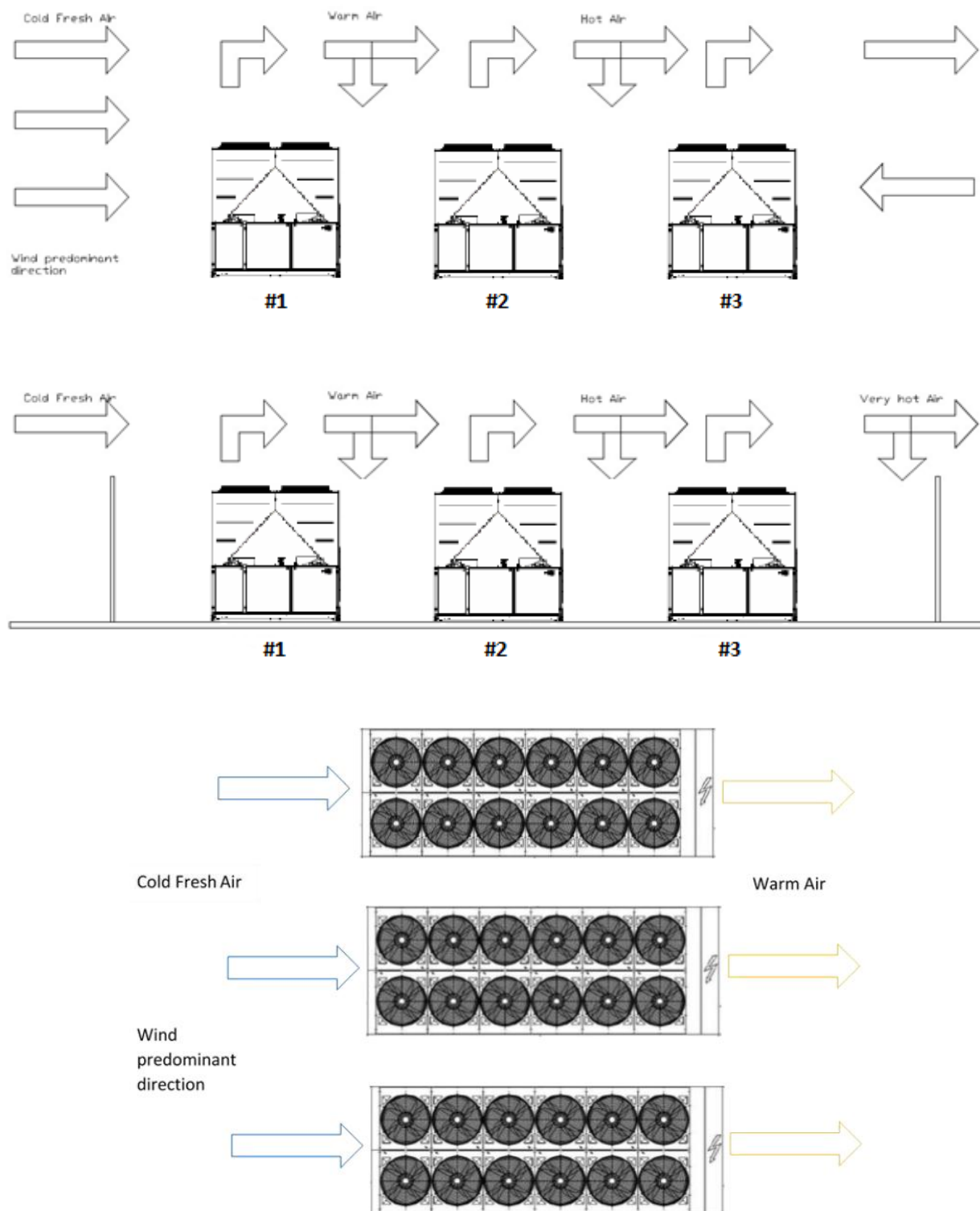
Sl. 17 – Instalacija višestruke jedinice (način hlađenja)
