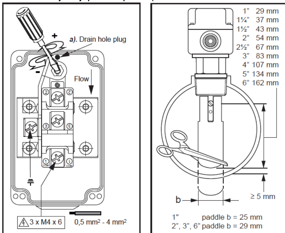
Sl. 19 – Namještanje prekidača protoka (model F61TB-9100 – Johnson Controls)
