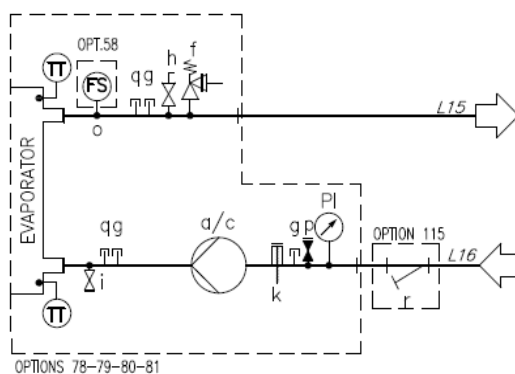
Sl. 22 – Hidraulički dijagram za jednu pumpu / dvostruku pumpu s spremnikom (EWYTx5B) (opt. 134-135) (maks. radni tlak 6 bara)
