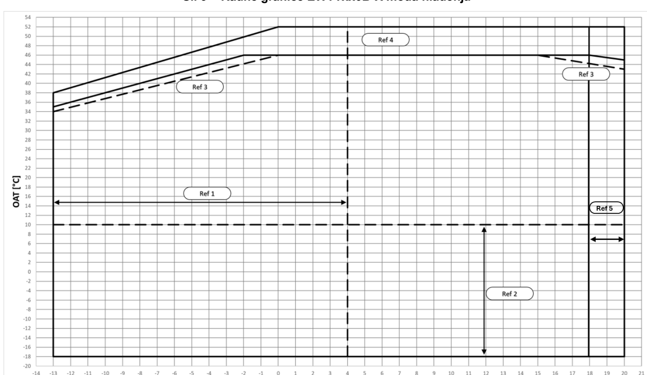
SI. 9 – Radne granice EWYTxx0B-X moda hlađenja
