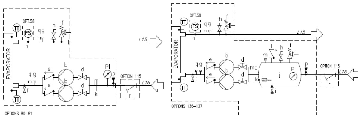
Sl. 23 – Hidraulički dijagram za dvostruku pumpu (EWYTx5B) (opcija 80-81/136-137) (maks. radni tlak 6 bara).
