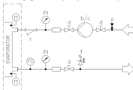
Sl. 21 – Hidraulički dijagram za jednu pumpu / dvostruku pumpu (EWYTx5B) (opt. 78-79) (maks. radni tlak 6 bara)
