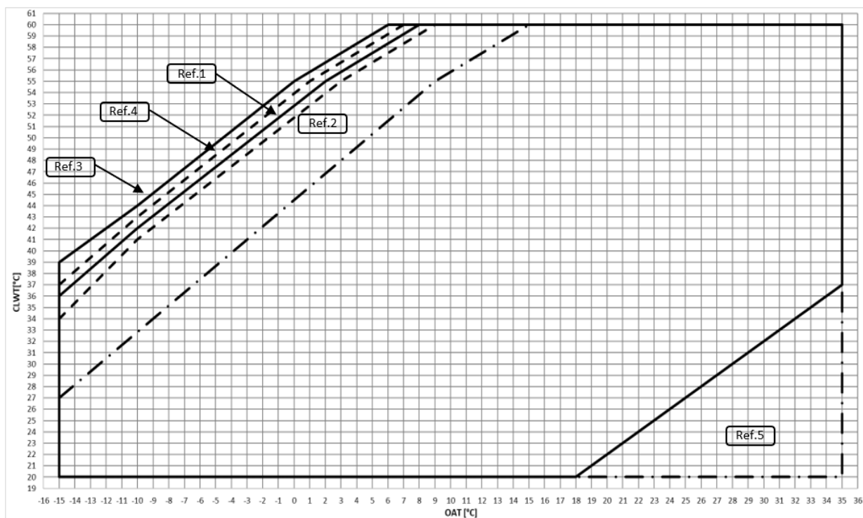
Sl. 11 – Radne granice EWYT ~ B-X načina grijanja
