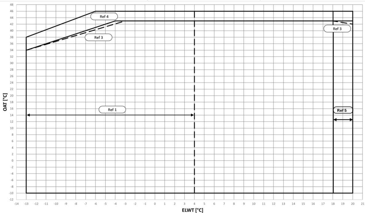
Sl. 7 – Radne granice EWYTx5B-X moda hlađenja
