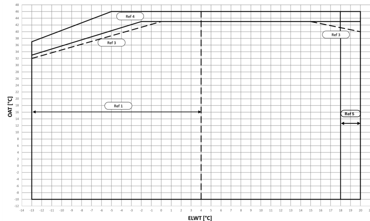
SI. 6 – Radne granice EWYTx5B-S načina hlađenja
