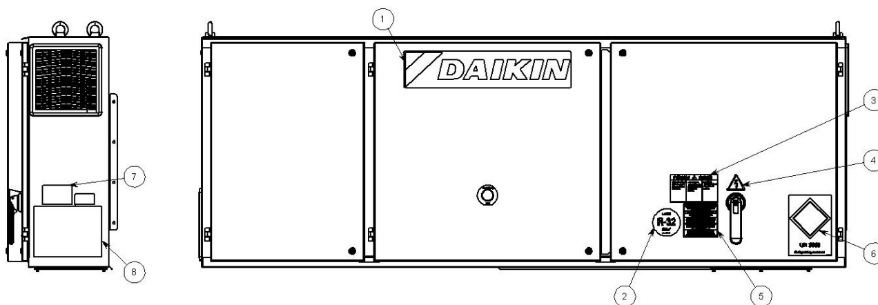
Sl. 5 – Opis naljepnica primijenjenih na električnu ploču EWYTxx0B
