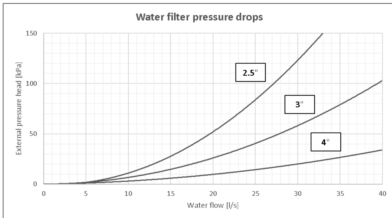
Sl. 18 – Pad tlaka filtra za vodu
