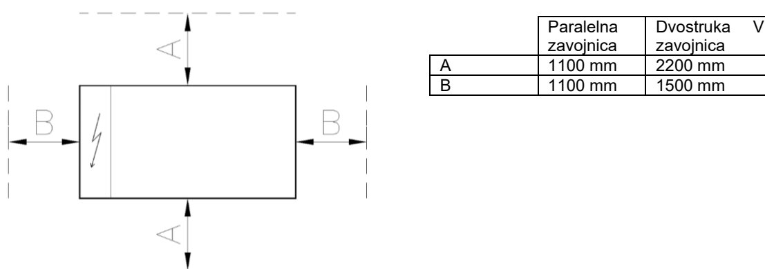
Sl. 16 – Minimalni zahtjevi za prostor
