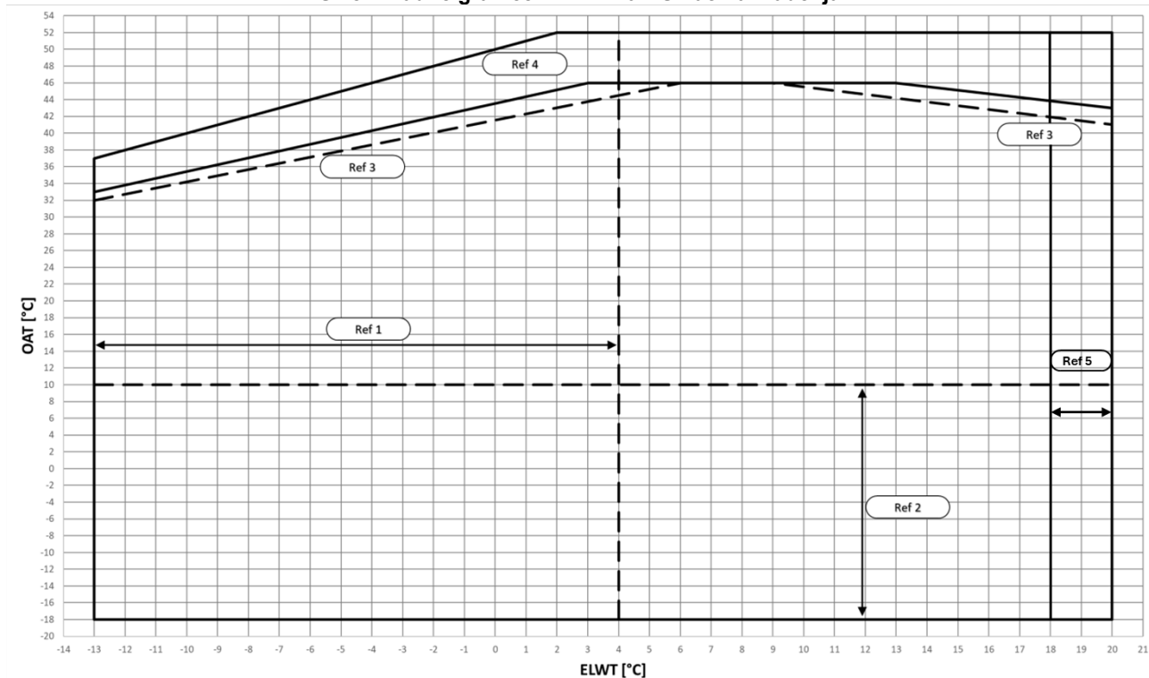
SI. 9 – Radne granice EWYTxx0B-X moda hlađenja
