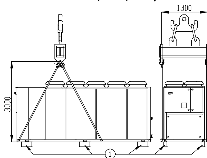
Sl. 14 – Upute za podizanje
