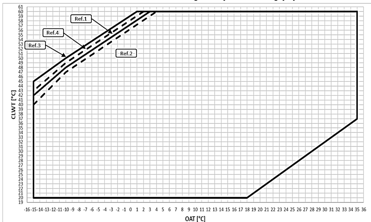
SI. 13 – EWYT ~B-X – OP.204 Ograničenja rada načina grijanja
