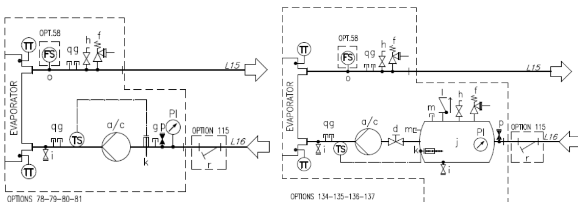
Sl. 24 – Hidraulički dijagram za jednu pumpu / dvostruku pumpu (opcija 78-79-80-81/134-135-136-137) (maks. radni tlak 6 bara)
