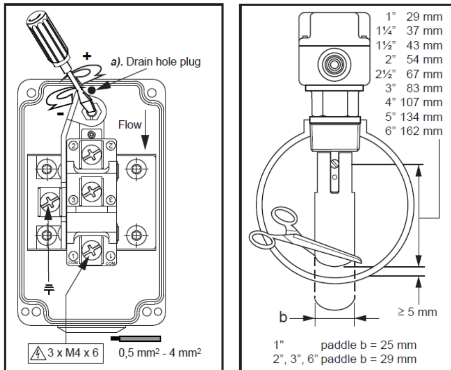
Fig. 19 – Regolazione del flussostato (modello F61TB-9100 – Johnson Controls)
