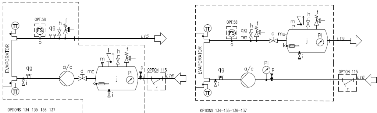
Fig. 22 - Schema idraulico per pompa singola/pompa doppia con serbatoio (EWYTx5B) (opz. 134-135) (pressione massima operativa 6 bar)
