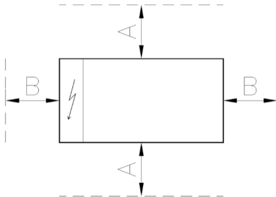
Fig. 16 - Requisiti di spazio minimi
