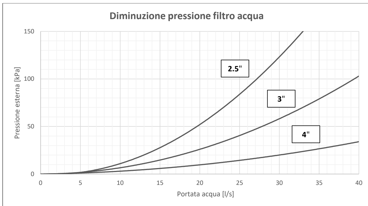
Fig. 18 - Calo di pressione del filtro dell'acqua
