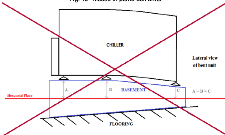
Fig. 15 - Messa in piano dell'unità
