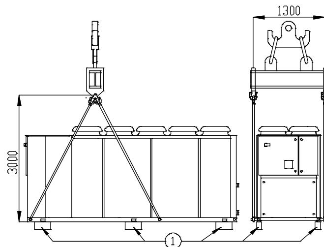
Fig. 14 - Istruzioni di sollevamento
