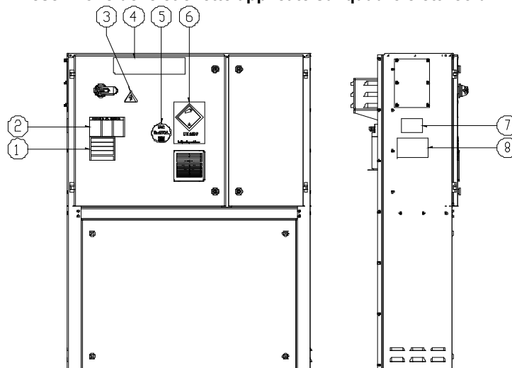
Fig. 4 - Descrizione delle etichette applicate sul quadro elettrico di EWYTxx5B
