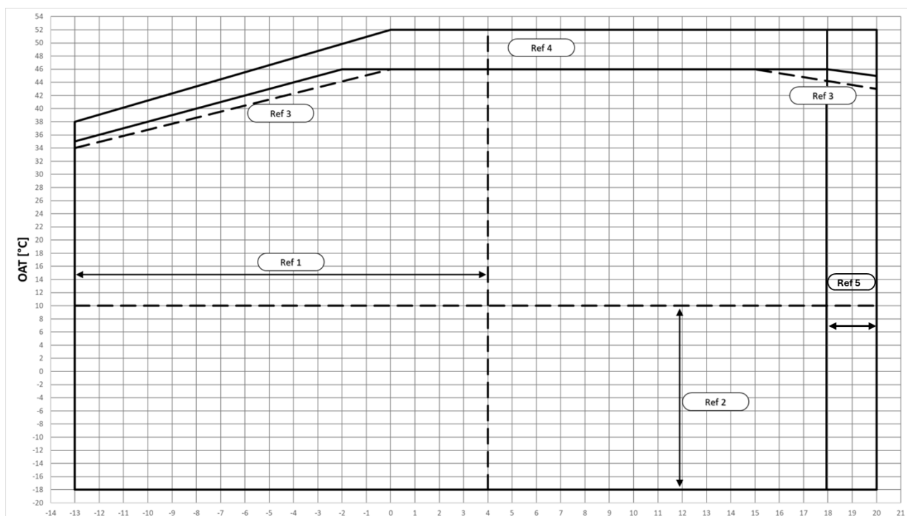
Fig. 9 - Limiti operativi della modalità di raffreddamento di EWYTx0B-X
