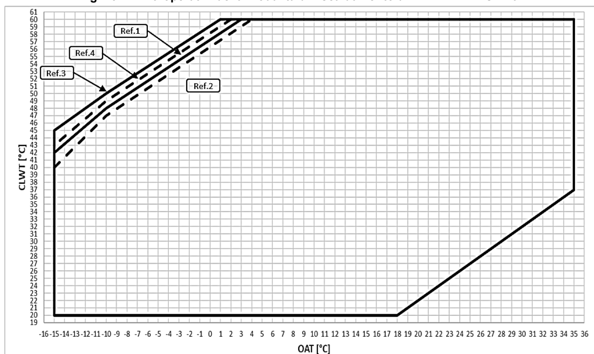
Fig. 13 - Limiti operativi della modalità di riscaldamento di EWYT~B-X - OP.204
