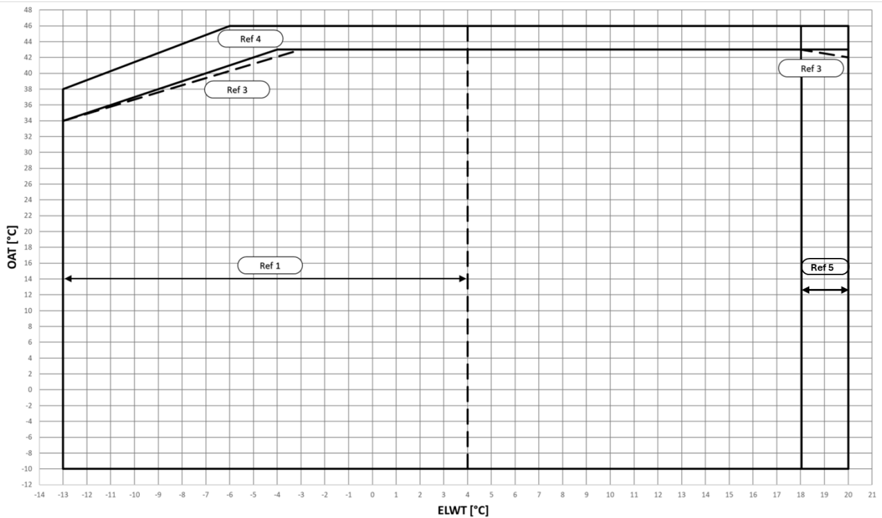
Fig. 7 - Limiti operativi della modalità di raffreddamento di EWYTxx5B-X
