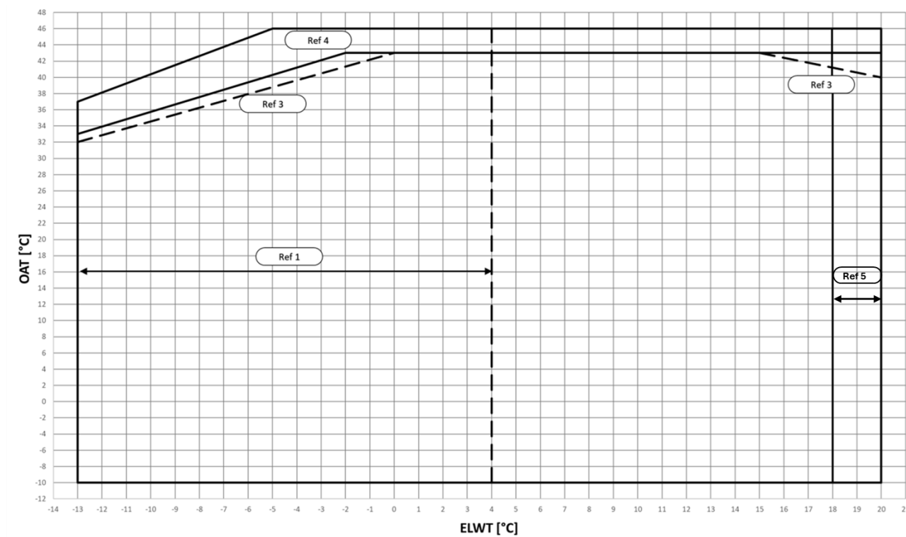
Fig. 6 - Limiti operativi della modalità di raffreddamento di EWYTxx5B-S
