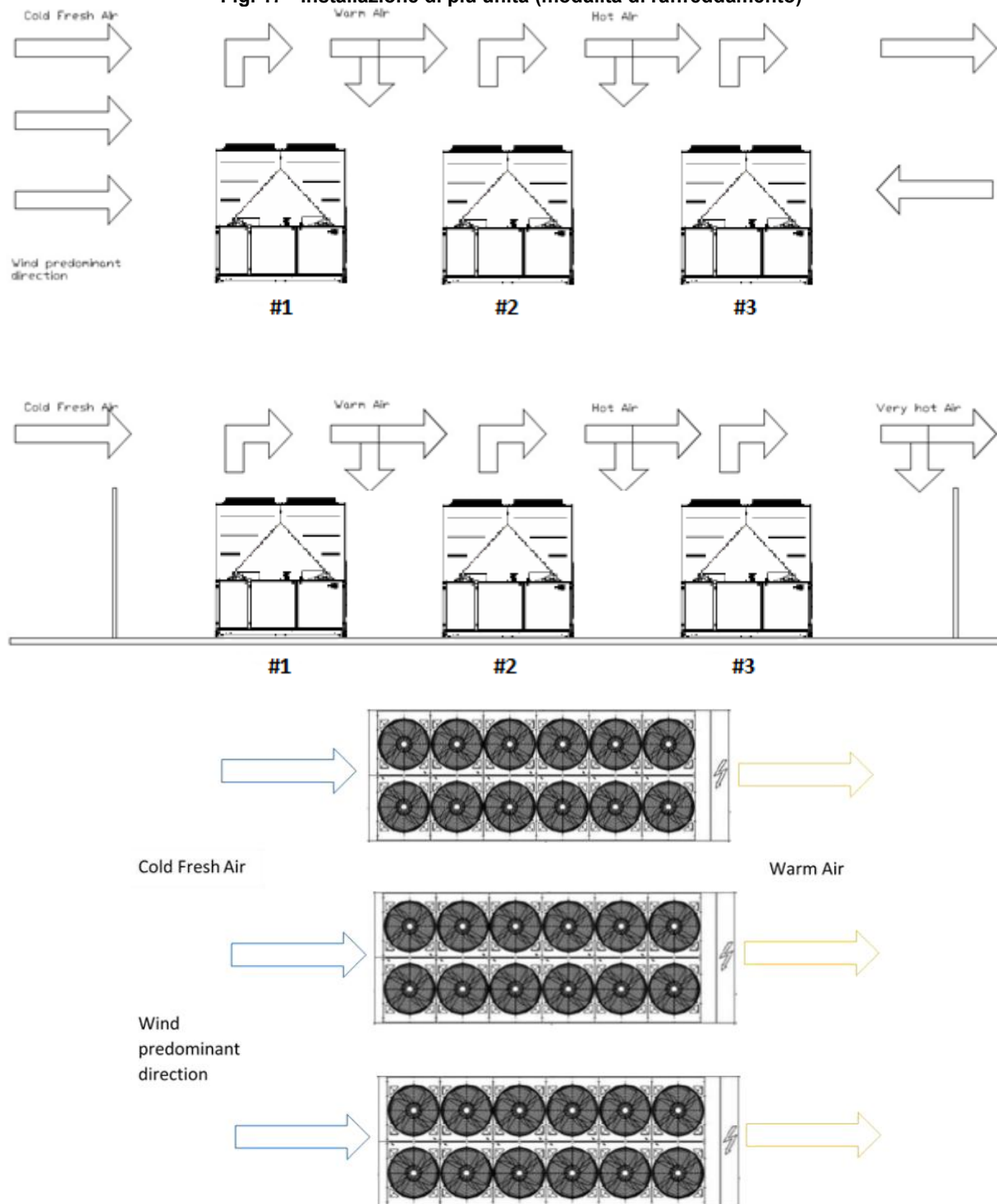
Fig. 17 - Installazione di più unità (modalità di raffreddamento)
