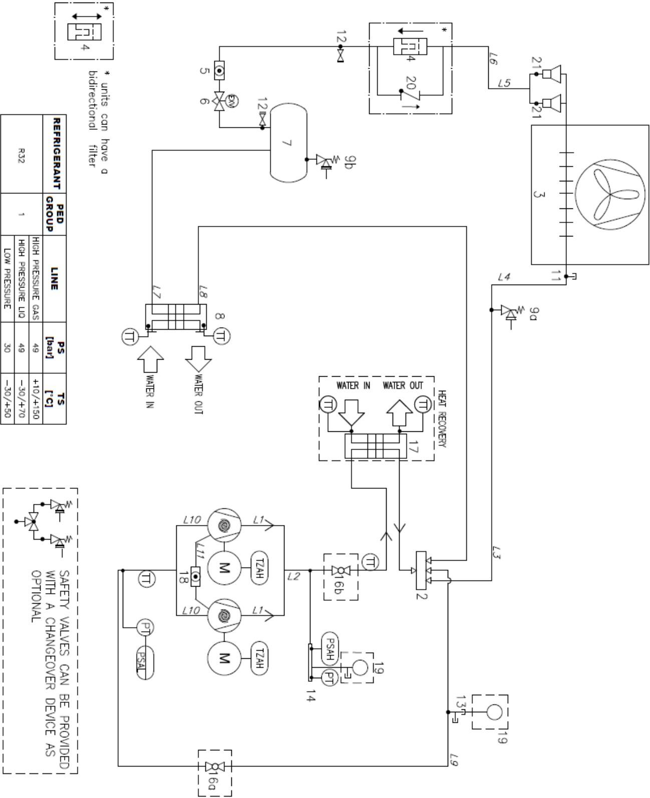
Fig. 1 - Schema delle tubazioni del refrigerante (P&ID) per unità a circuito singolo EWYTxx5B
