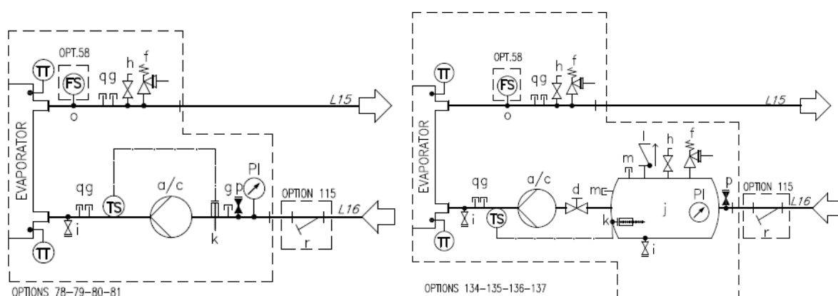
Fig. 24 - Schema idraulico per pompa singola/pompa doppia (EWATxx0B) (opz. 78-79-80-81/134-135-136-137) (pressione massima operativa 6 bar)
