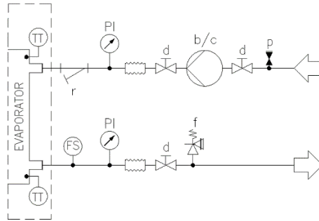
Fig. 21 - Schema idraulico per pompa singola/pompa doppia (EWYTx5B) (opz. 78-79) (pressione massima operativa 6 bar)
