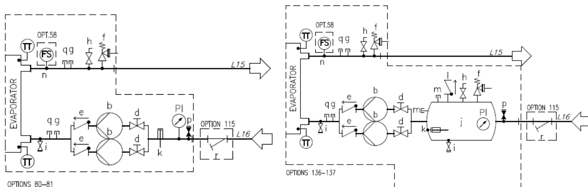
Fig. 24 - Schema idraulico per pompa singola/pompa doppia (EWATxx0B) (opz. 78-79-80-81/134-135-136-137) (pressione massima operativa 6 bar)
