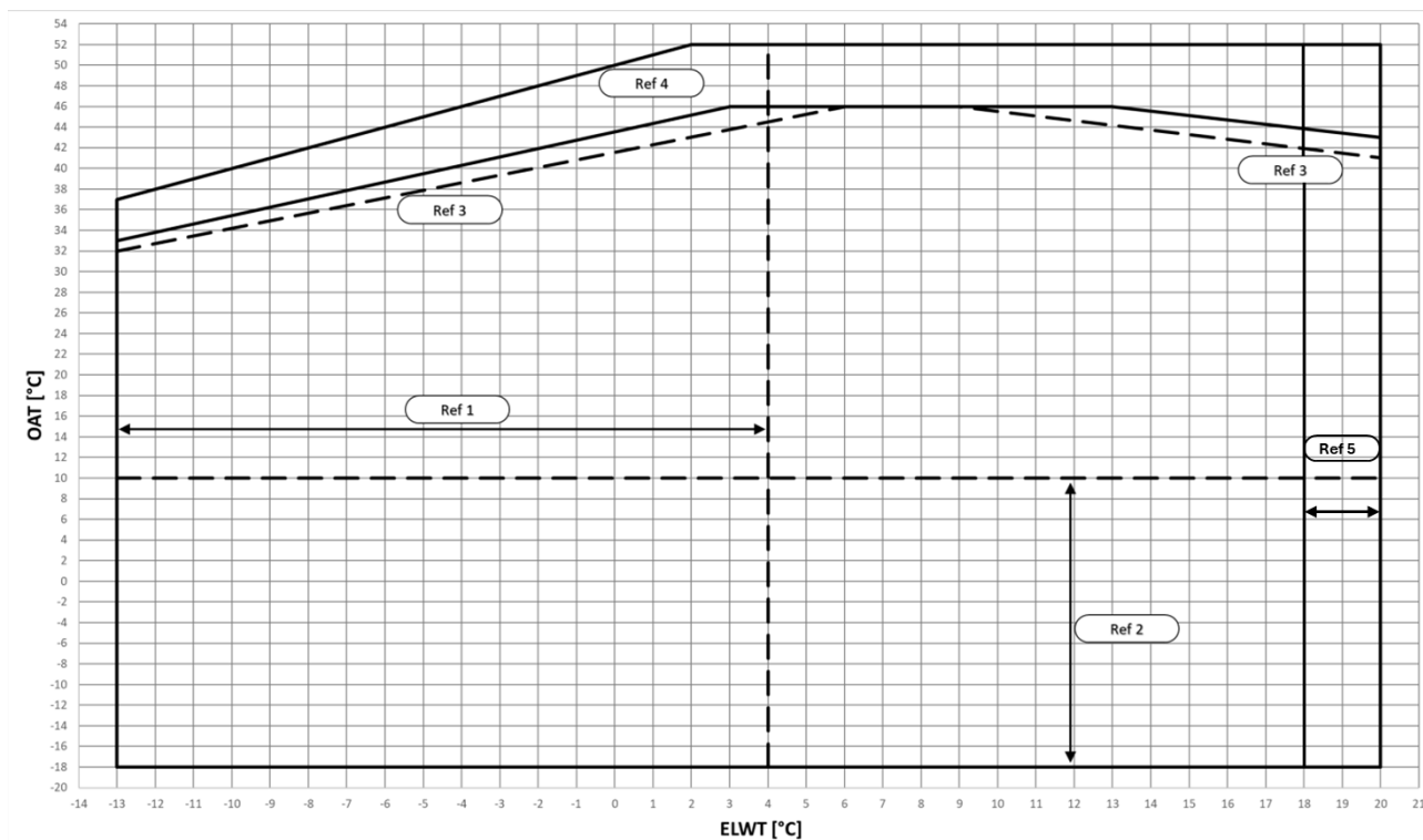
Afb. 9 – EWYTx0B-X Operationele limieten modus koeling
