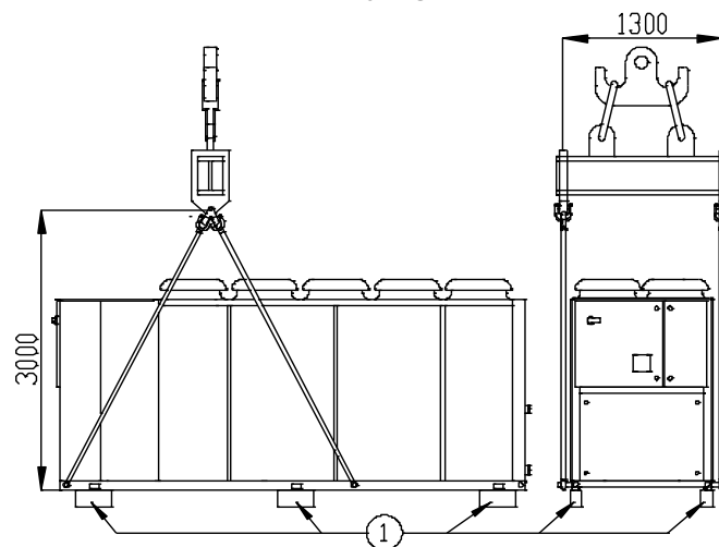
Afb. 14 – Aanwijzingen voor heffen
