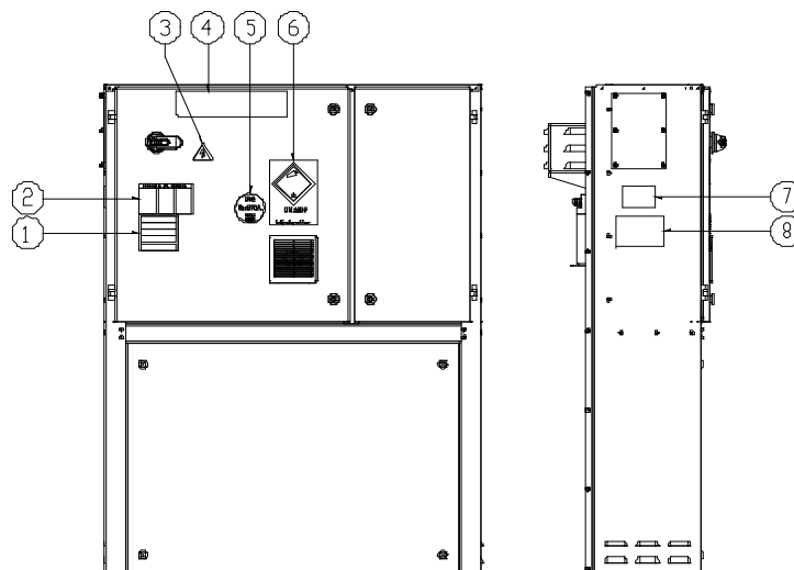
Afb. 4 – Beschrijving van de plaatjes op het schakelbord EWYTxx5B
