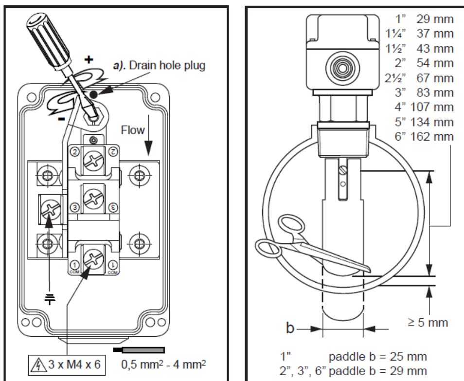
Afb. 19 – Afstelling stromingsschakelaar (model F61TB-9100 – Johnson Controls)
