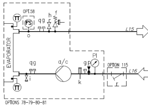
Afb. 22 – Hydraulisch schema voor enkele / dubbele pomp met tank (EWYTx5B) (optie 134-135) (max. bedrijfsdruk 6 bar)
