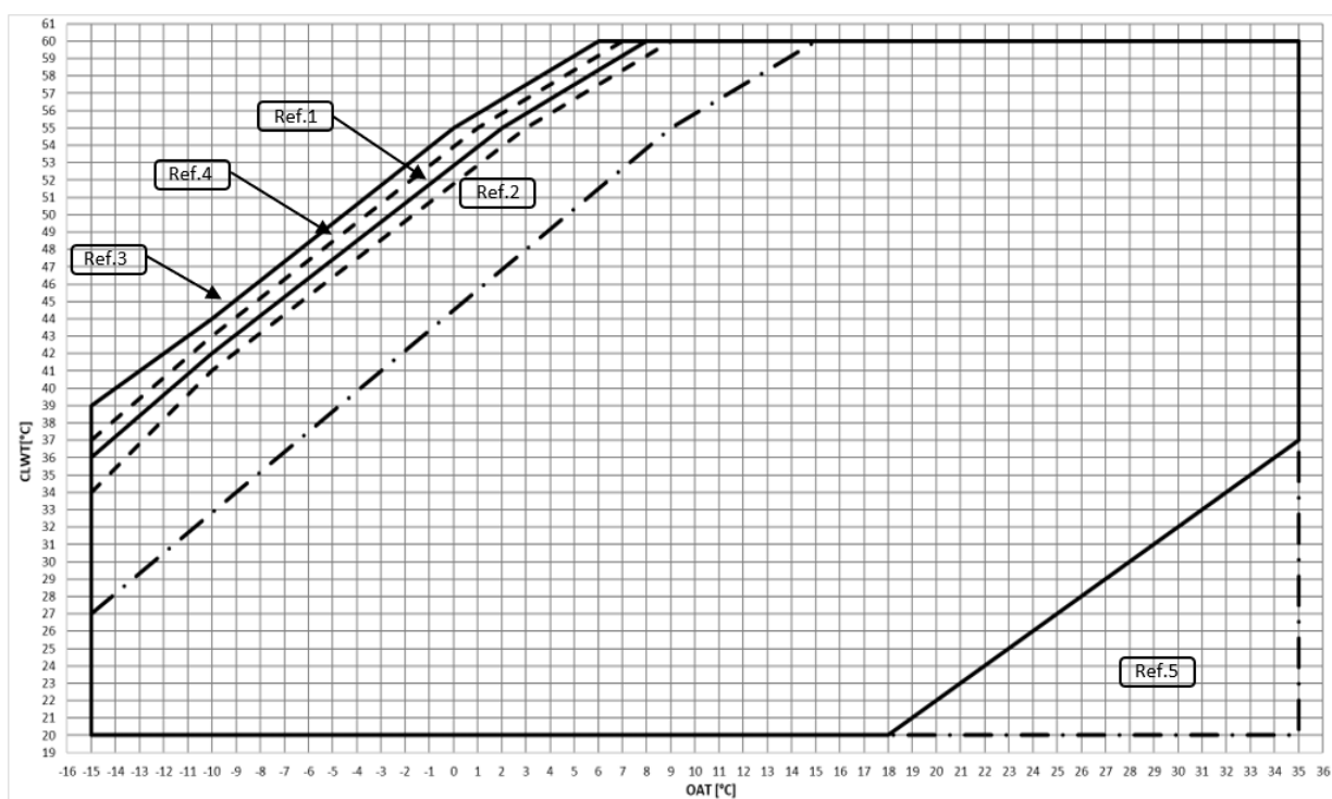
Afb. 11 – EWYT~B-X Operationele limieten modus verwarming
