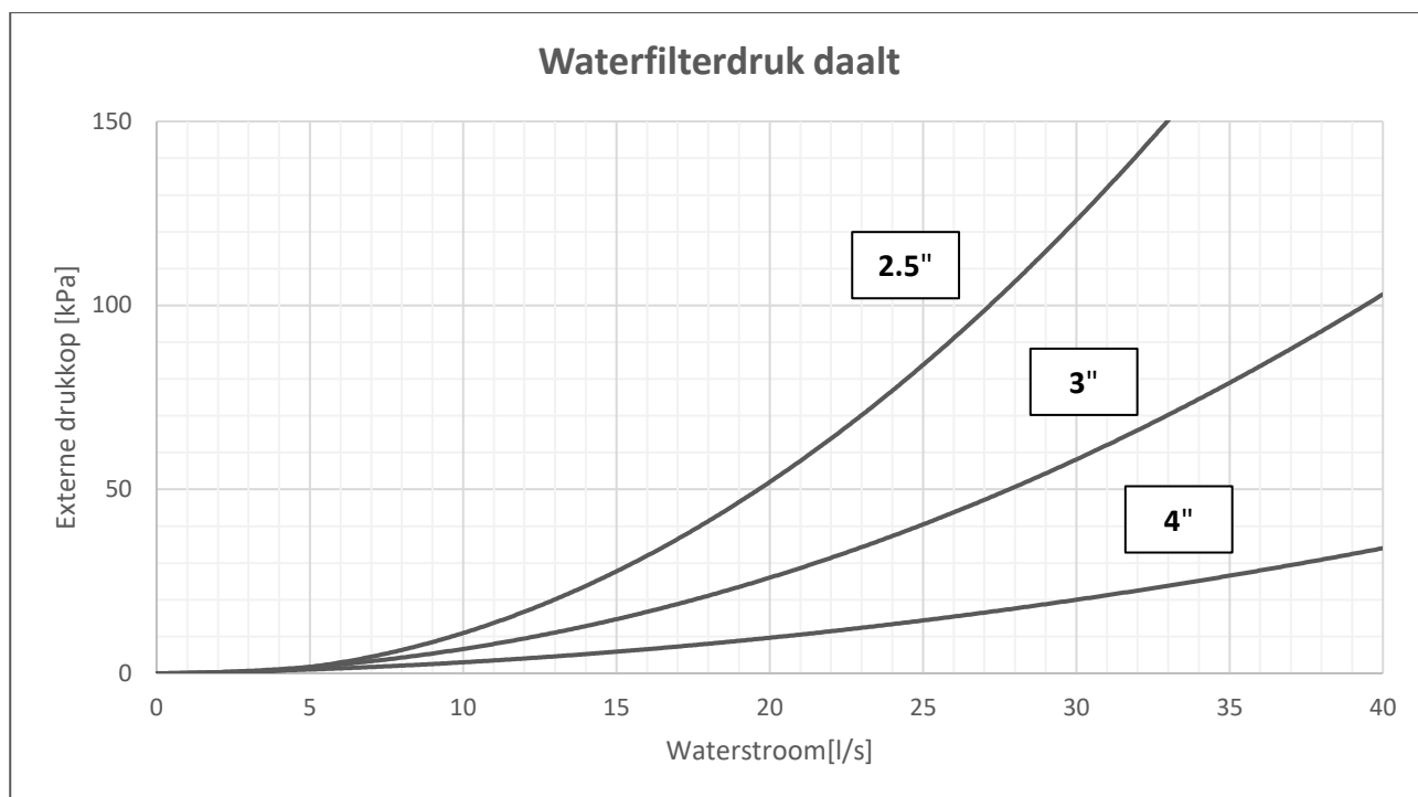
Afb. 18 – Drukvermindering waterfilter
