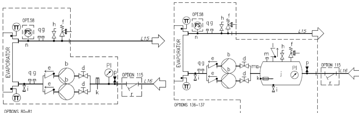
Afb. 23 – Hydraulisch schema voor dubbele pomp (optie 80-81/136-137) (max. bedrijfsdruk 6 bar)
