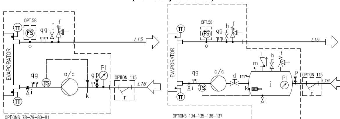
Afb. 24 - Hydraulisch schema voor enkele / dubbele pomp (EWATxx0B) (optie 78-79-80-81/134-135-136-137) (max. bedrijfsdruk 6 bar)
