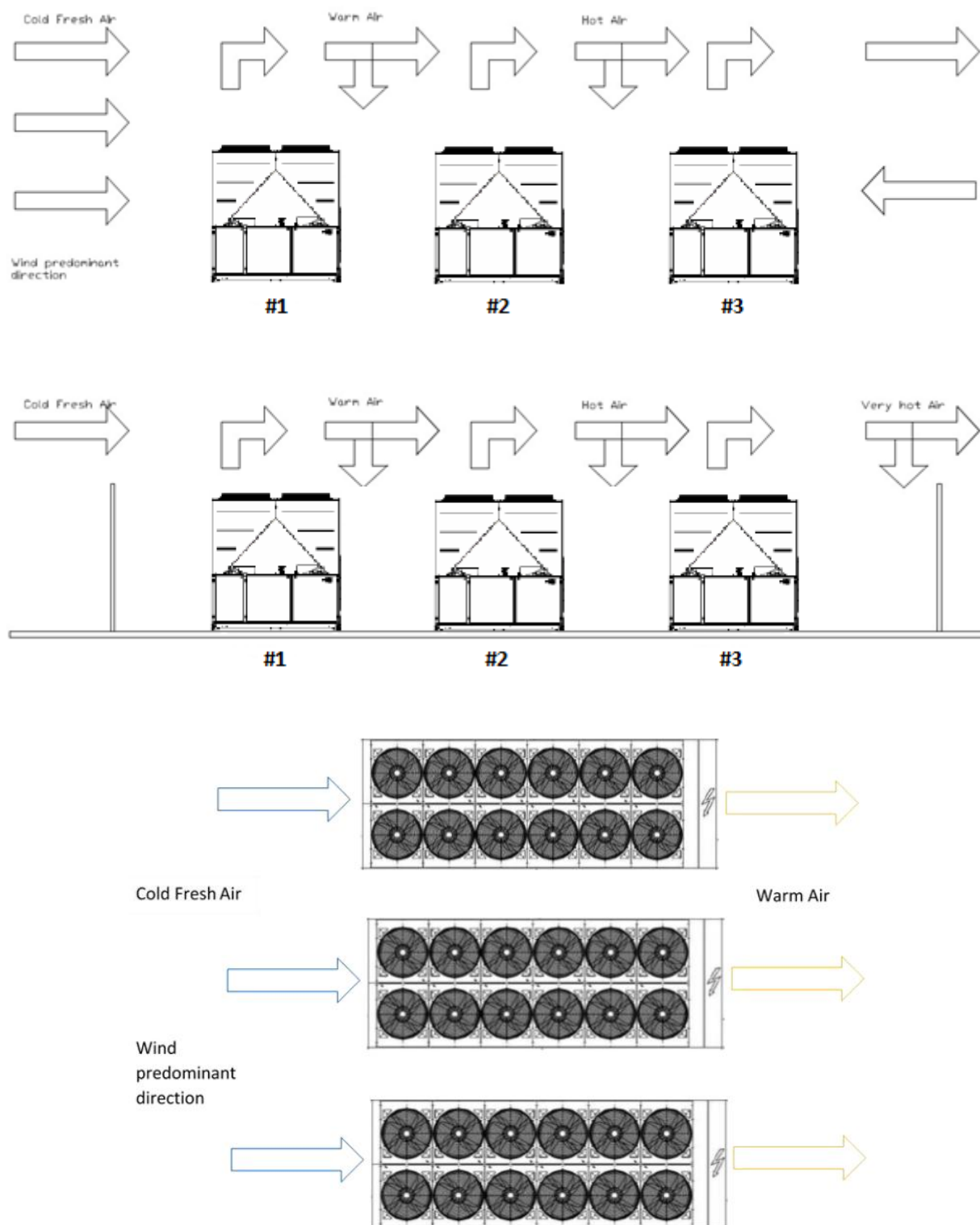
Afb. 17 – Installatie meerdere systemen (modus koeling)
