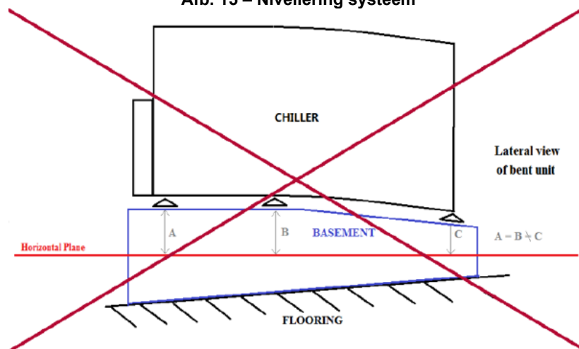
Afb. 15 – Nivellering systeem
