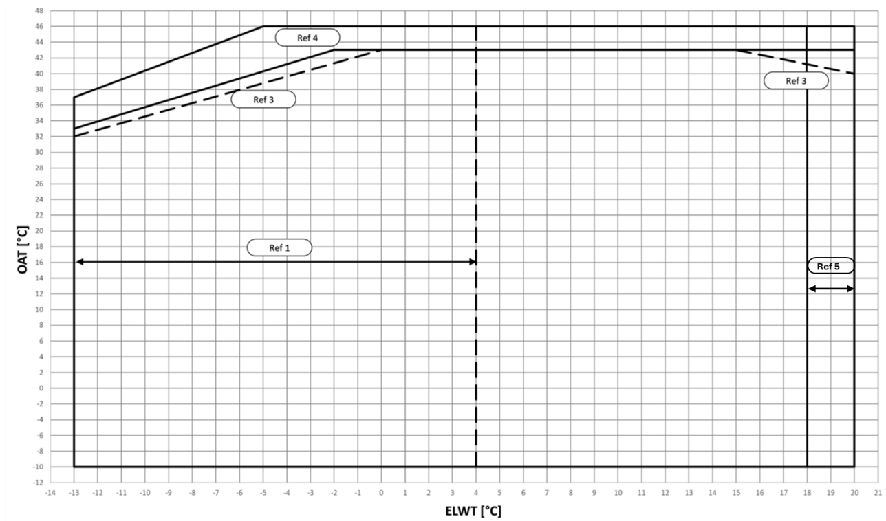
Afb. 6 – EWYTx5B-S Operationele limieten modus koeling
