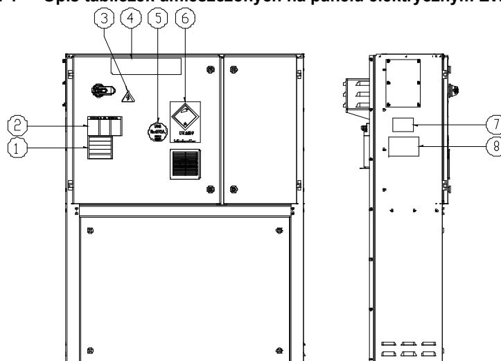
Rys. 4 — Opis tabliczek umieszczonych na panelu elektrycznym EWYTx5B
