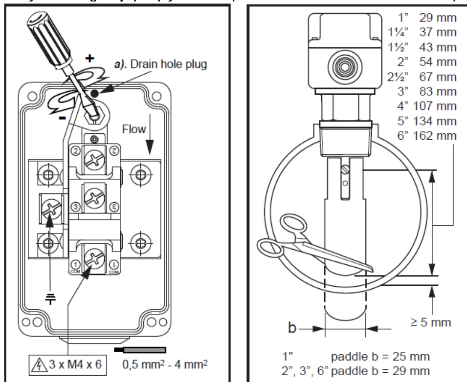
Rys. 19 – Regulacja przepływomierza (model F61TB-9100 – Johnson Controls)
