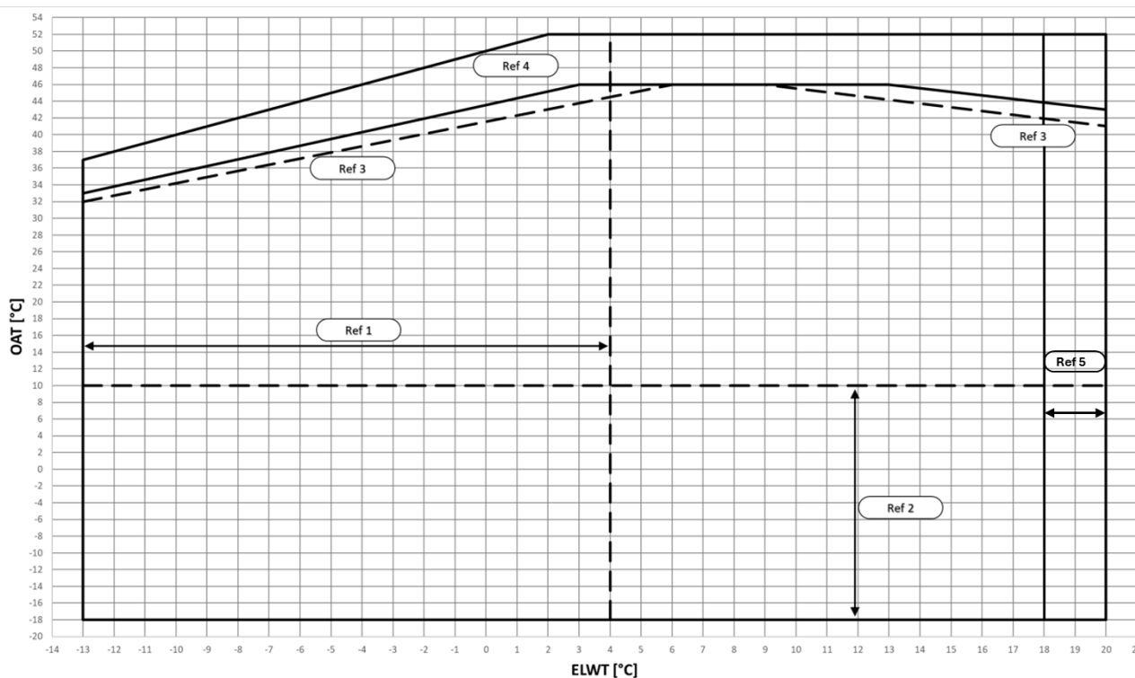
Rys. 8 — EWYTx0B-S — limity operacyjne trybu chłodzenia
