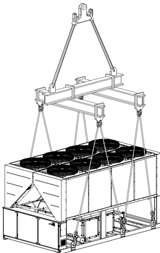
Jednostka z 6 punktami podnoszenia
