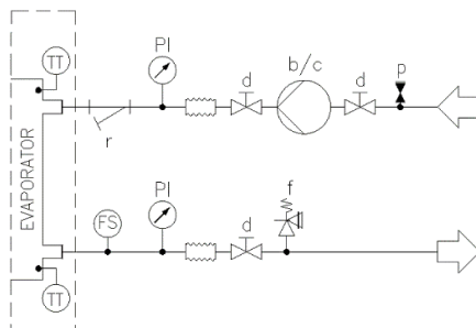
Rys. 21 — Schemat hydrauliczny pompy pojedynczej/pompy podwójnej (EWTxx5B) (opcja 78-79) (maks. ciśnienie robocze 6 bar)
