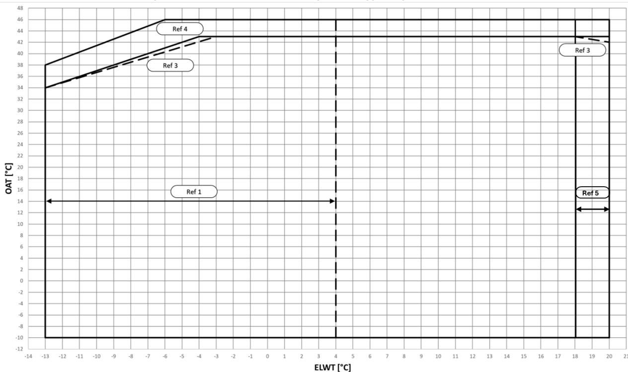
Rys. 7 — EWYTx5B-X — limity operacyjne trybu chłodzenia
