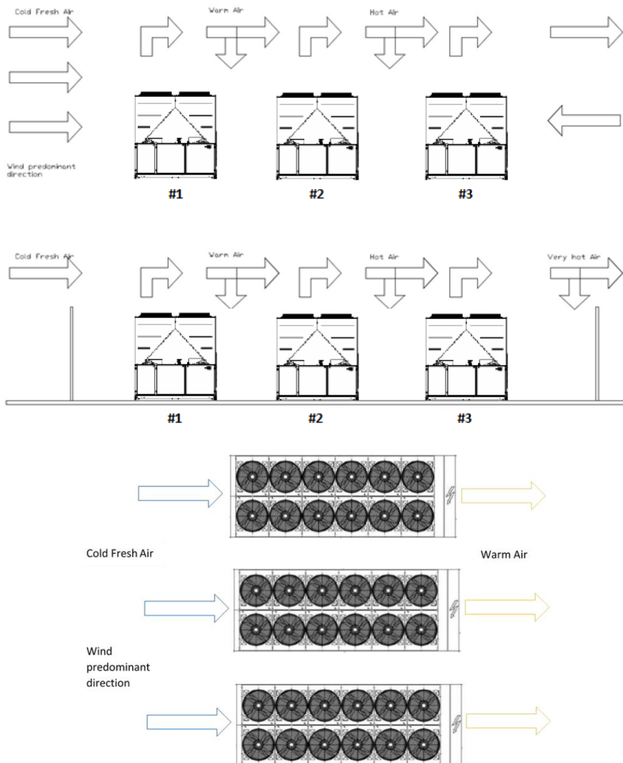
Rys. 17 — Instalacja wielu jednostek (tryb chłodzenia)
