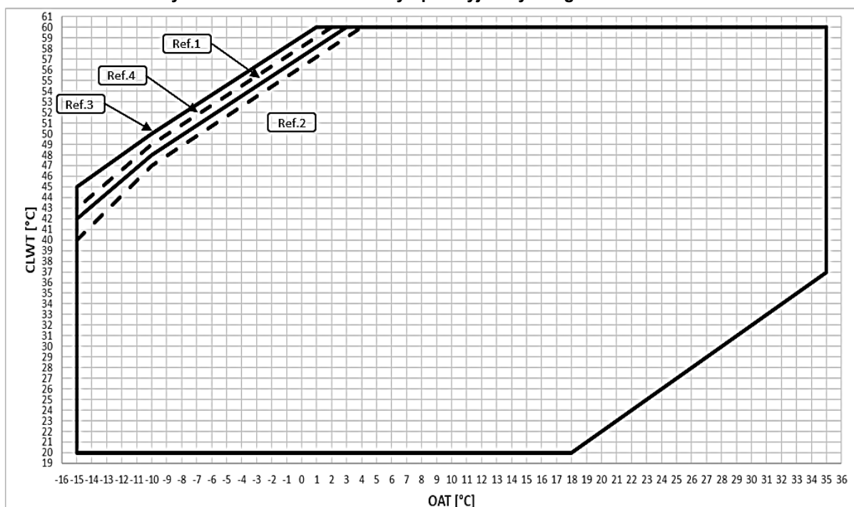
Rys. 13 — EWYT~B-X — limity operacyjne trybu ogrzewania OP.204
