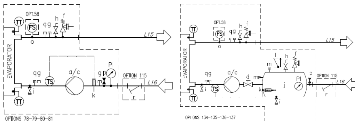
Rys. 24 — Schemat hydrauliczny pompy pojedynczej/pompy podwójnej (opcja 78-79-80-81/134-135-136-137) (maks. ciśnienie robocze 6 bar)
