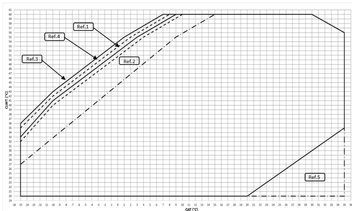
Rys. 10 — EWYT-B-S — limity operacyjne trybu ogrzewania
