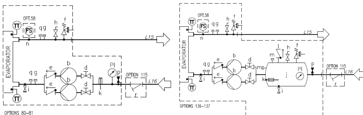
Rys. 23 — Schemat hydrauliczny pompy podwójnej (EWTxx5B) (opcja 80-81/136-137) (maks. ciśnienie robocze 6 bar)
