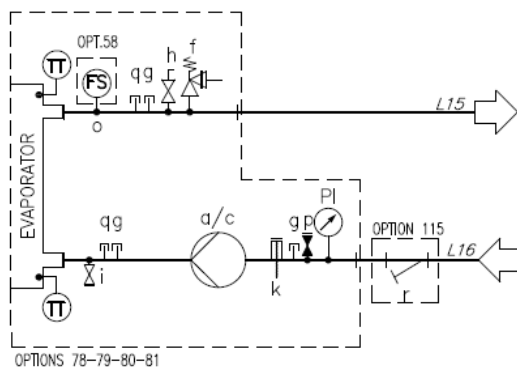
Rys. 22 — Schemat hydrauliczny pompy pojedynczej/pompy podwójnej ze zbiornikiem (EWTxx5B) (opcja 134-135) (maks. ciśnienie robocze 6 bar)
