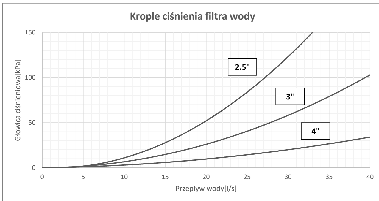
Rys. 18 — Spadek ciśnienia filtra wody
