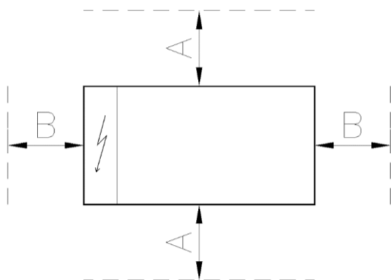
Rys. 16 — Wymagania dotyczące przestrzeni minimalnej
