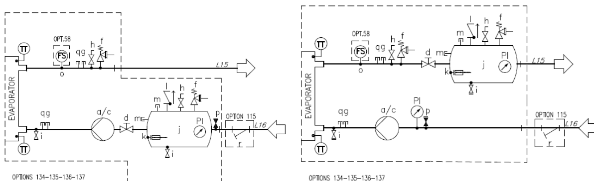
Rys. 23 — Schemat hydrauliczny pompy podwójnej (EWTxx5B) (opcja 80-81/136-137) (maks. ciśnienie robocze 6 bar)
