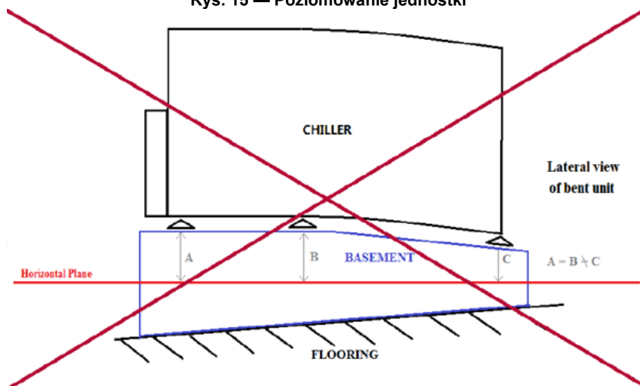
Rys. 15 — Wypoziomowanie jednostki
