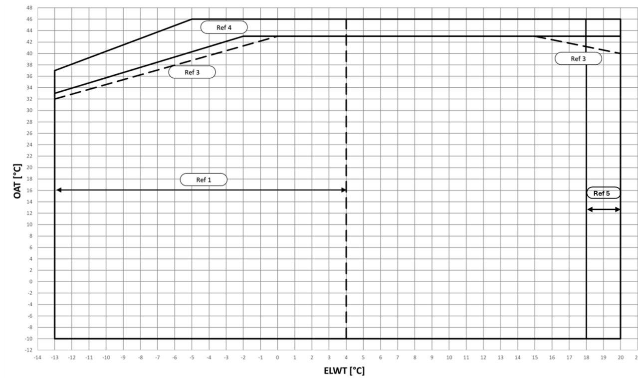
Rys. 6 — EWYTx5B-S — limity operacyjne trybu chłodzenia
