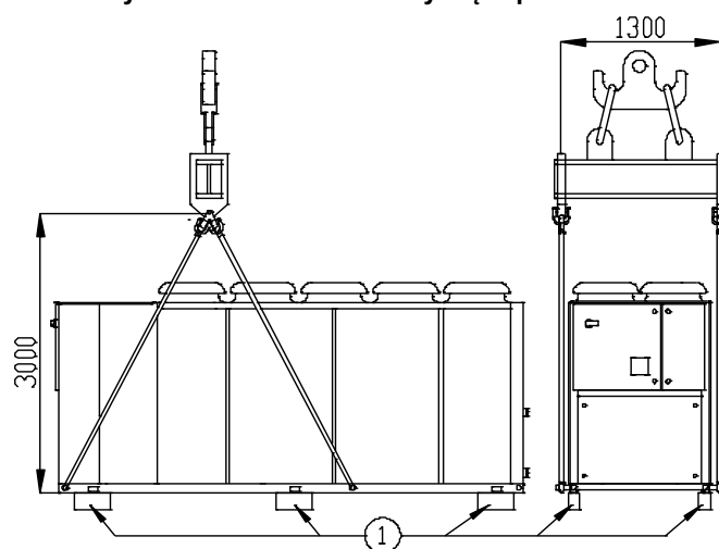
Rys. 14 — Wskazówki dotyczące podnoszenia
