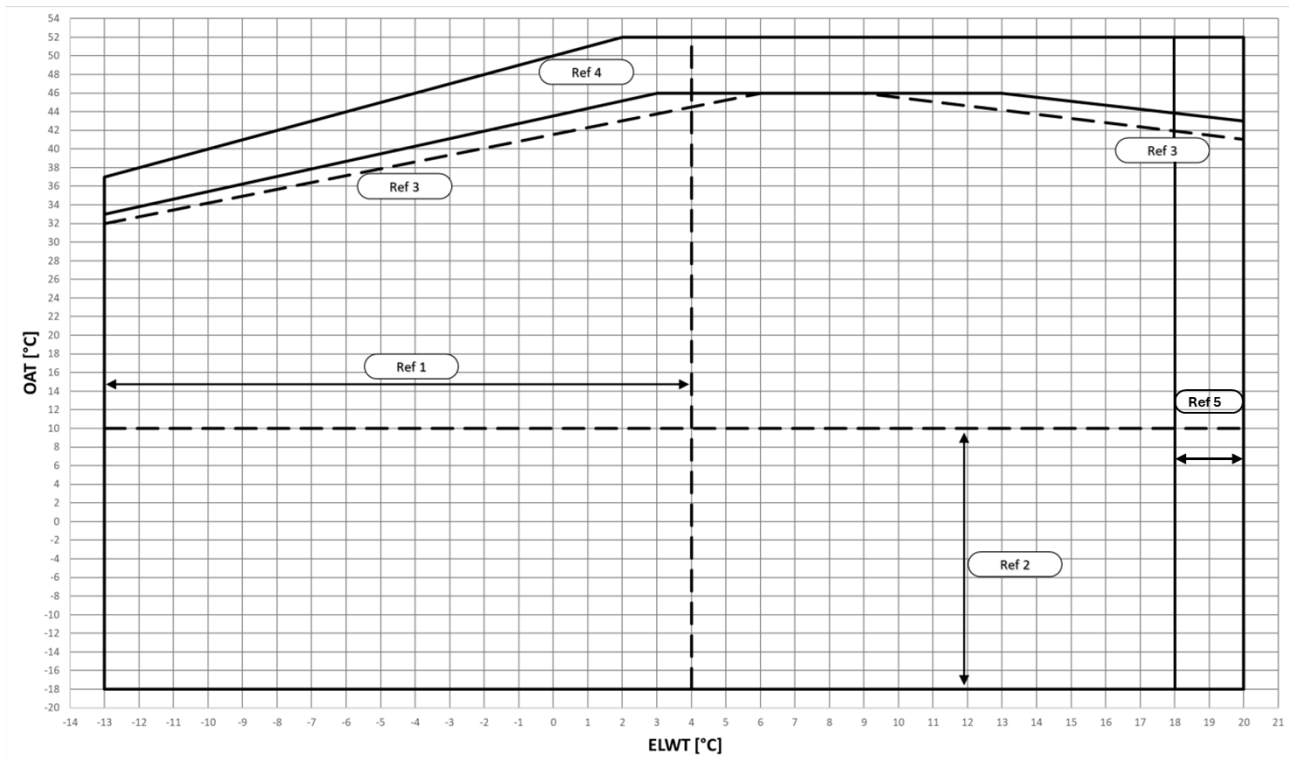
Fig. 8 – Limites operativos do modo de refrigeração EWYTxx0B-S
