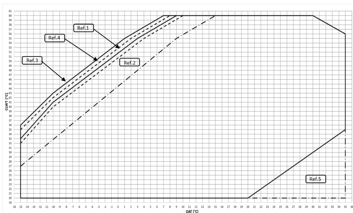
Fig. 10 – Limites operativos do modo de aquecimento EWYT~B-S
