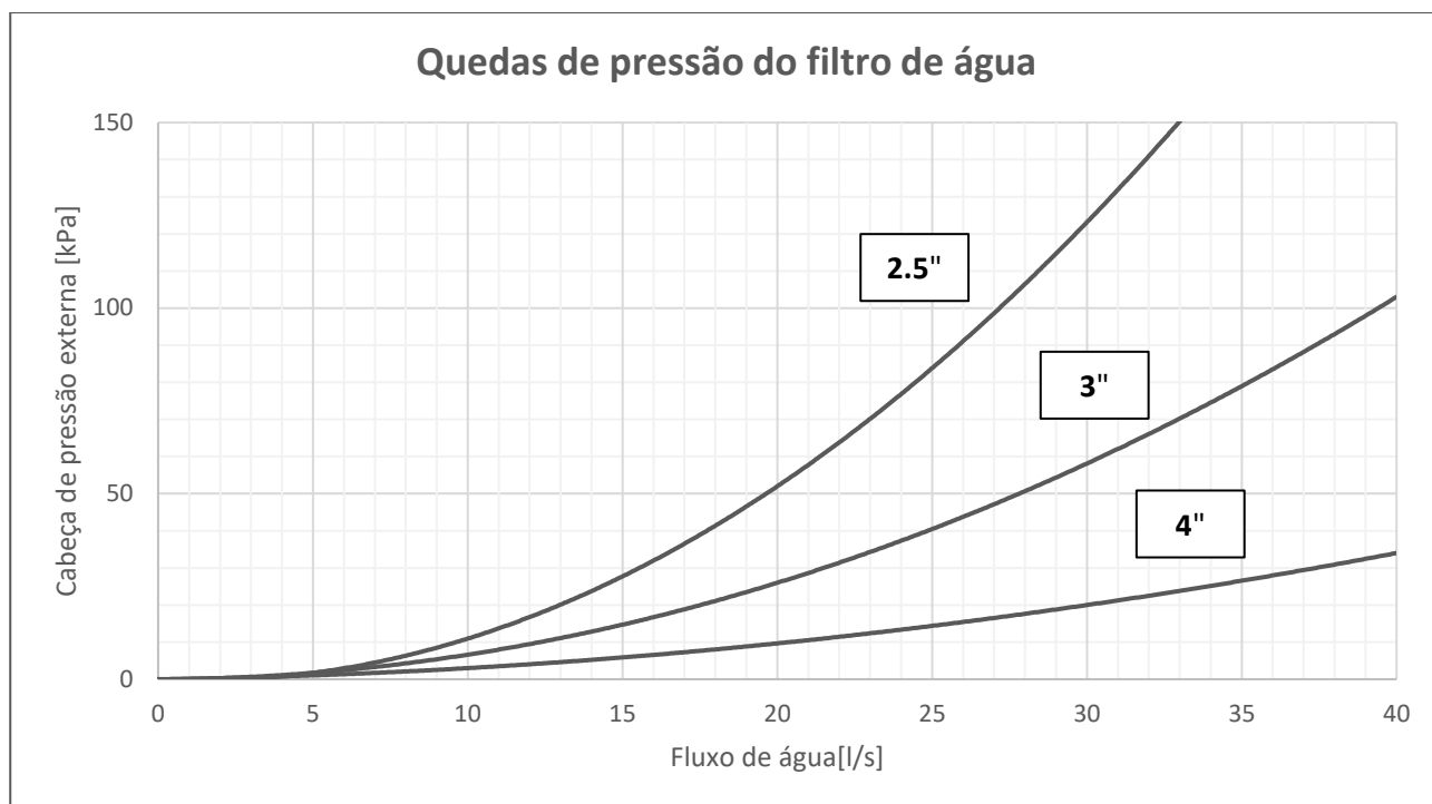
Fig. 18 – Queda de pressão no filtro de água
