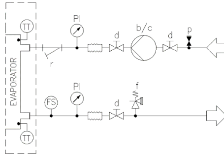
Fig. 21 – Diagrama hidráulico para bomba única / bomba dupla (EWYTx5B) (opc. 78-79) (pressão máxima de funcionamento 6 bar)
