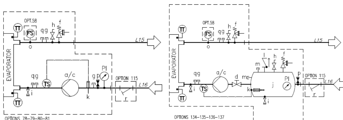
Fig. 24 – Diagrama hidráulico para bomba única / bomba dupla (opc. 78-79-80-81/134-135-136-137) (pressão máxima de funcionamento 6 bar)
