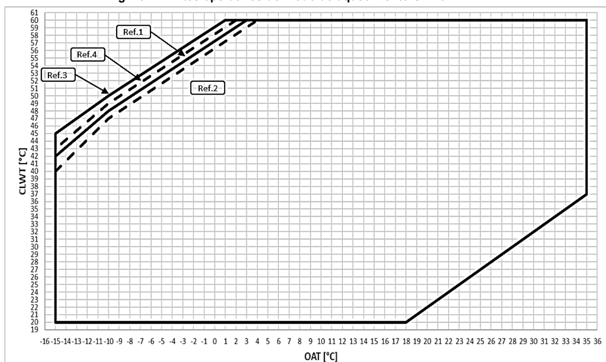
Fig. 13 – Limites operativos do modo de aquecimento OP.204 – EWYT~B-X
