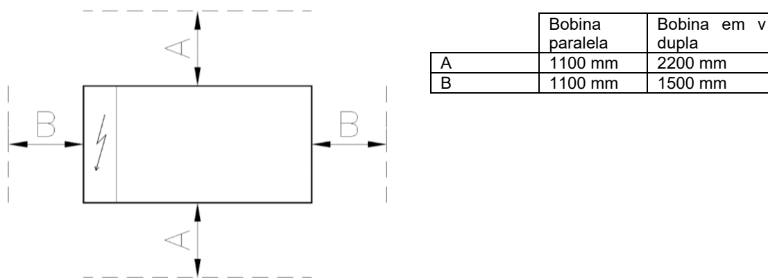
Fig. 16 – Requisitos mínimos de espaço
