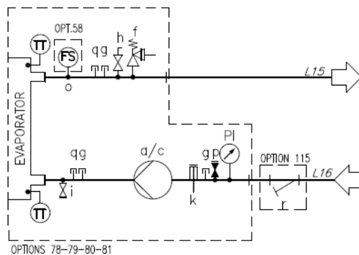
Fig. 22 – Diagrama hidráulico para bomba única / bomba dupla com tanque (EWYTx5B) (opc. 134-135) (pressão máxima de funcionamento 6 bar)
