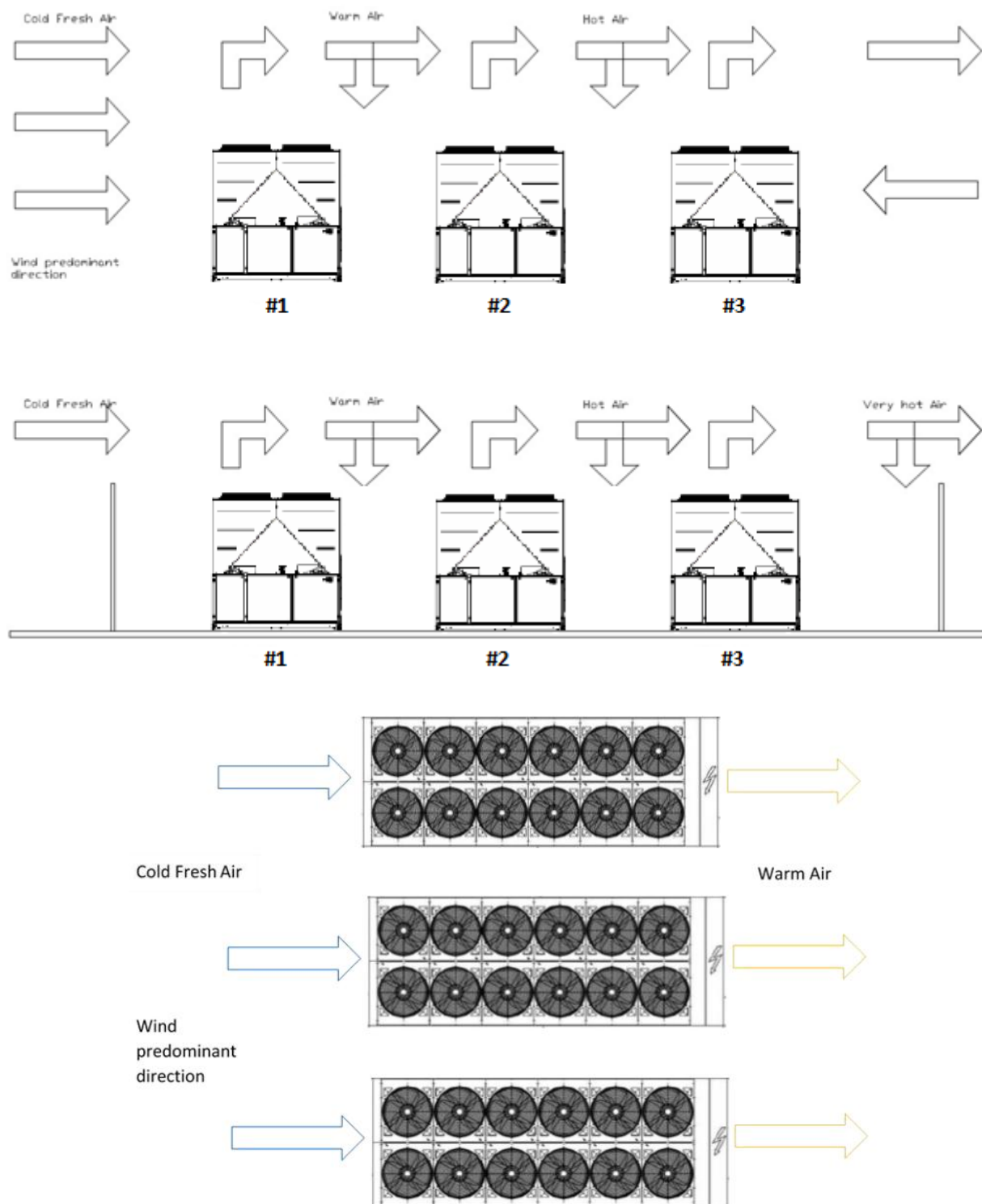
Fig. 17 – Instalação de várias unidades (modo de refrigeração)
