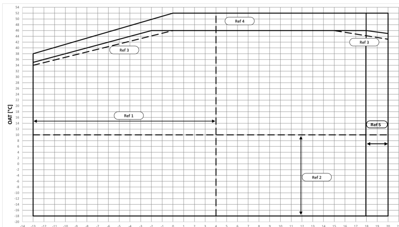
Fig. 9 – Limites operativos do modo de refrigeração EWYTx0B-X
