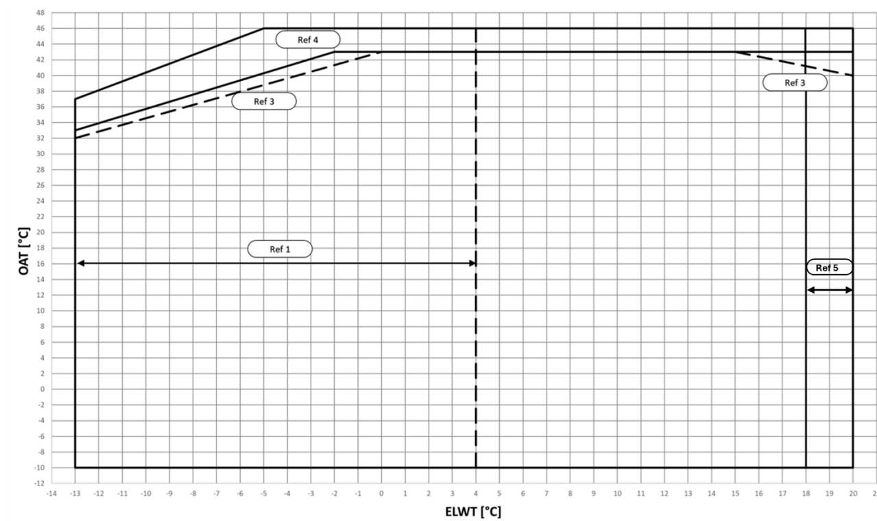
Fig. 6 – Limites operativos do modo de refrigeração EWYTxx5B-S
