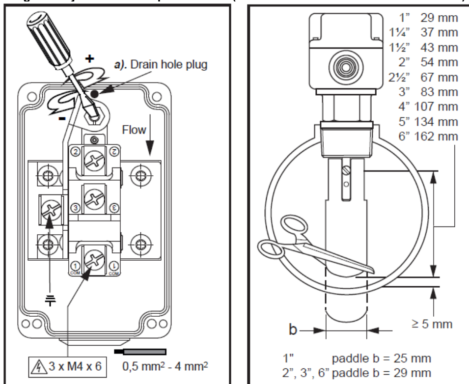
Fig. 19 – Ajuste do interruptor de fluxo (modelo F61TB-9100 – Johnson Controls)
