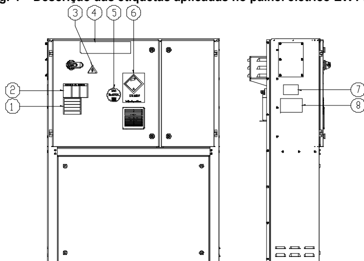
Fig. 4 – Descrição das etiquetas aplicadas no painel elétrico EWYTx5B
