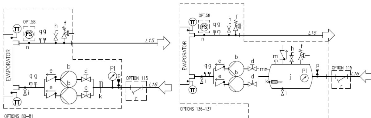
Fig. 23 – Diagrama hidráulico para bomba dupla (EWYTx5B) (opc. 80-81/136-137) (pressão máxima de funcionamento 6 bar)
