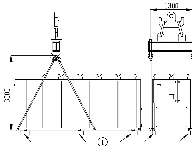
Fig. 14 – Instruções de levantamento
