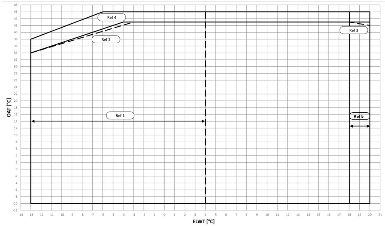
Fig. 7 – Limites operativos do modo de refrigeração EWYTxx5B-X
