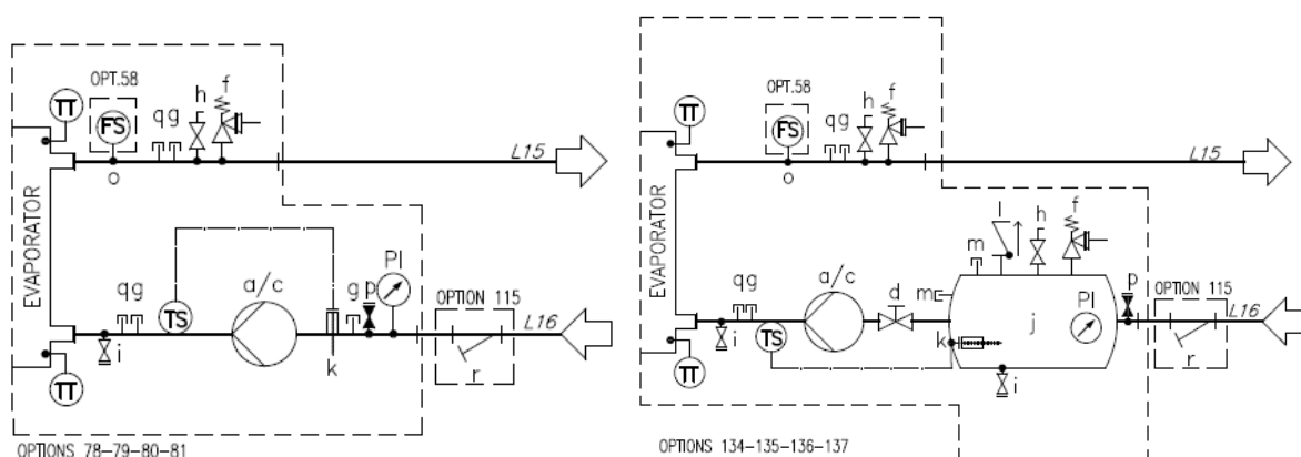
Fig. 24 – Diagrama hidraulică pentru o singură pompă /pompă dublă (opt. 78-79-80-81/134-135-136-137) (presiune max. de operare 6 bari)
