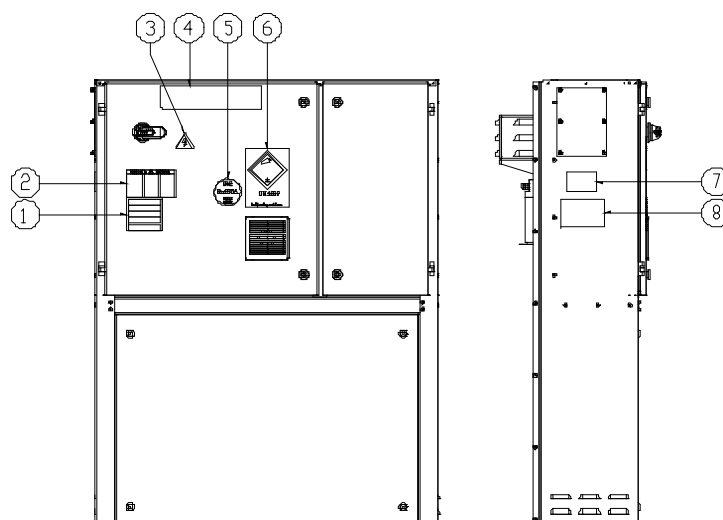
Fig. 4 – Descrierea etichetelor aplicate pe tabloul electric EWYTxx5B
