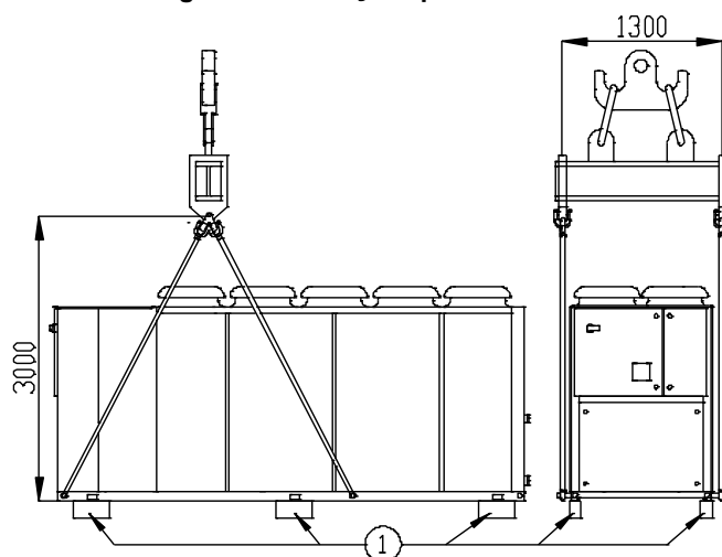
Fig. 14 – Instrucțiuni privind ridicarea
