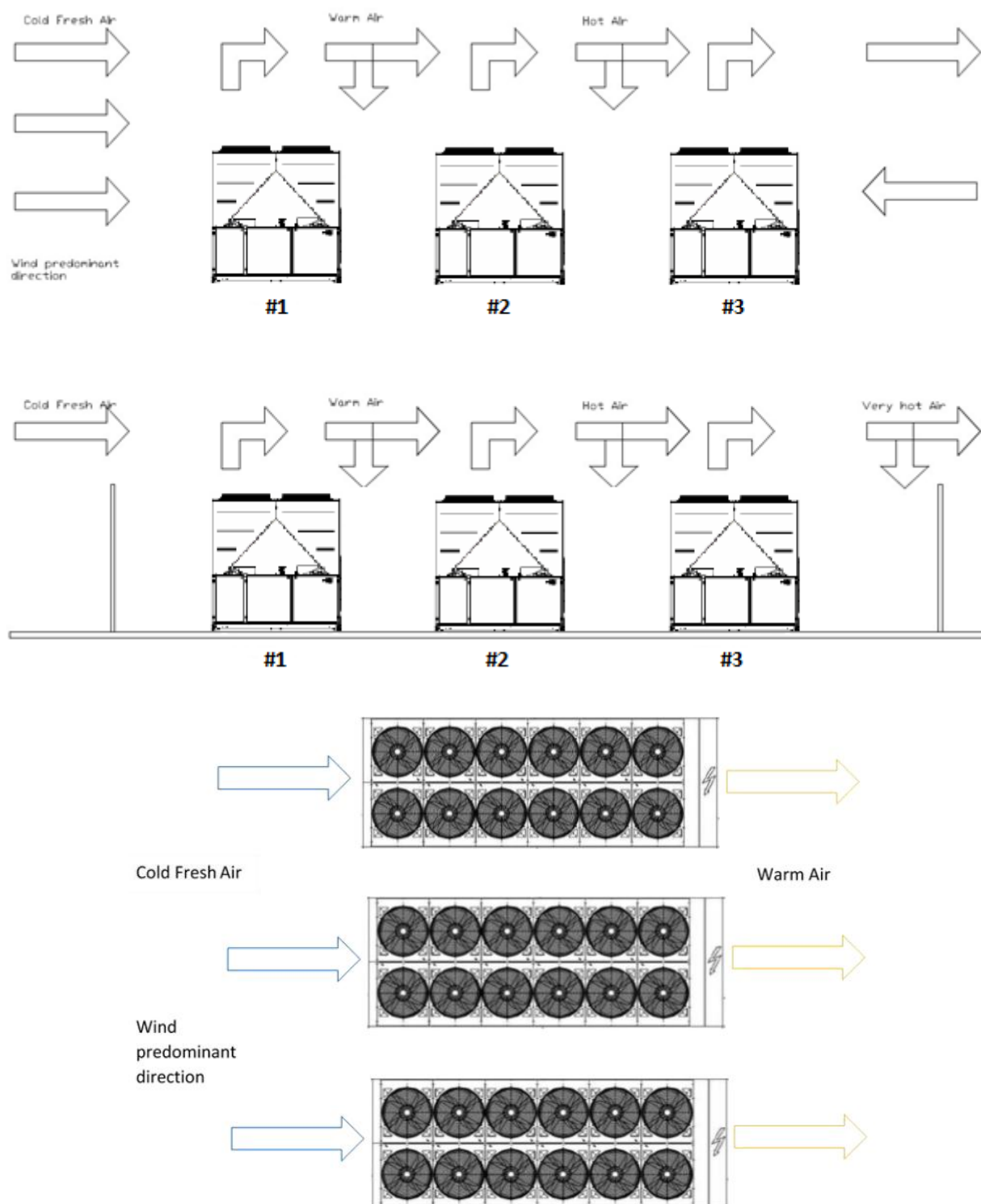
Fig. 17 – Instalarea mai multor răcitoare
