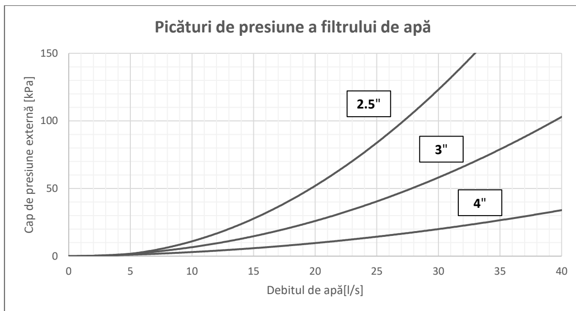
Fig. 18 –Cădere de presiune a filtrului de apă
