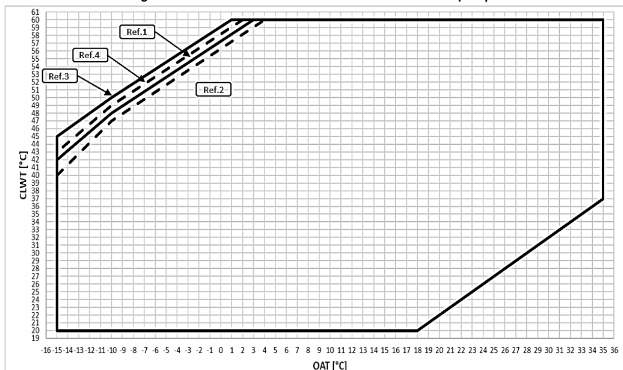
Fig. 13 – EWYT~B-X – OP.204 Modul de încălzire Limite operaționale
