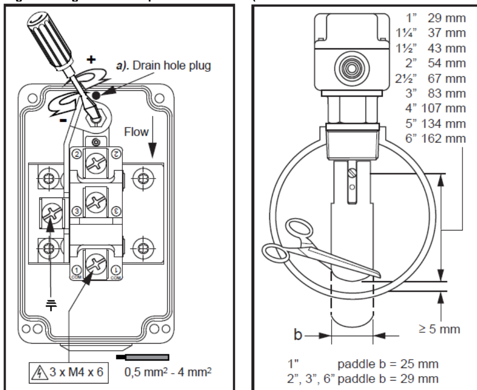
Fig. 19 – Reglarea întrerupătorului de debit (model F61TB-9100 – Johnson Controls)
