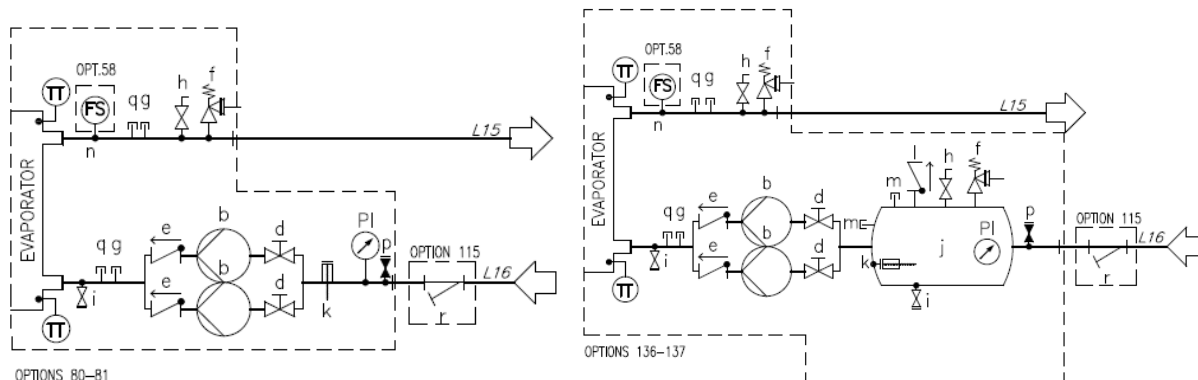
Fig. 23 – Diagrama hidraulica pentru pompa dubla (EWYTx5B) (opt. 80-81/136-137) (presiune max. de operare 6 bari)
