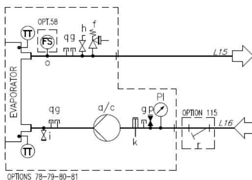
Fig. 22 – Diagrama hidraulică pentru o singură pompă /pompă dublă cu rezervor (EWYTx5B) (opt. 134-135) (presiune max. de operare 6 bari)
