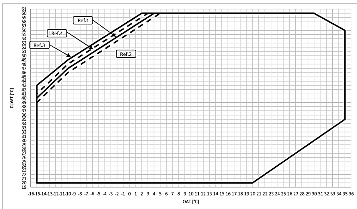
Fig. 12 – EWYT~B-S – OP.204 Modul de încălzire Limite operaționale
