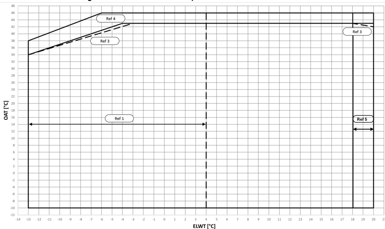
Fig. 7 – EWYTxx5B-X Limitele Operationale ale Modulului de Racire
