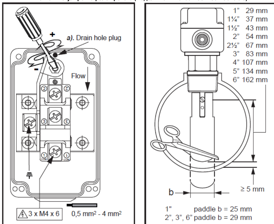
Рис. 19 – Регулировка реле потока (модель F61TB-9100 – Johnson Controls)
