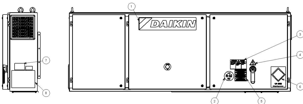
Рис. 5. Описание табличек, нанесенных на электрический щит EWYTxx0B
