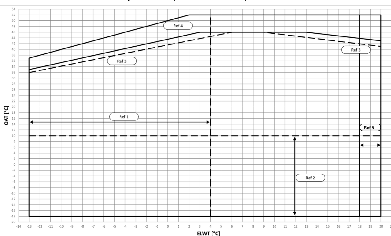
Рис. 8. Эксплуатационные пределы EWYTxh0B-S в режиме охлаждения
