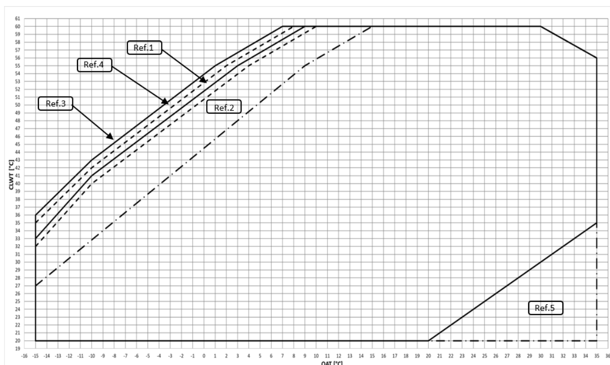
Рис. 10. Эксплуатационные пределы EWYT-B-S в режиме нагрева
