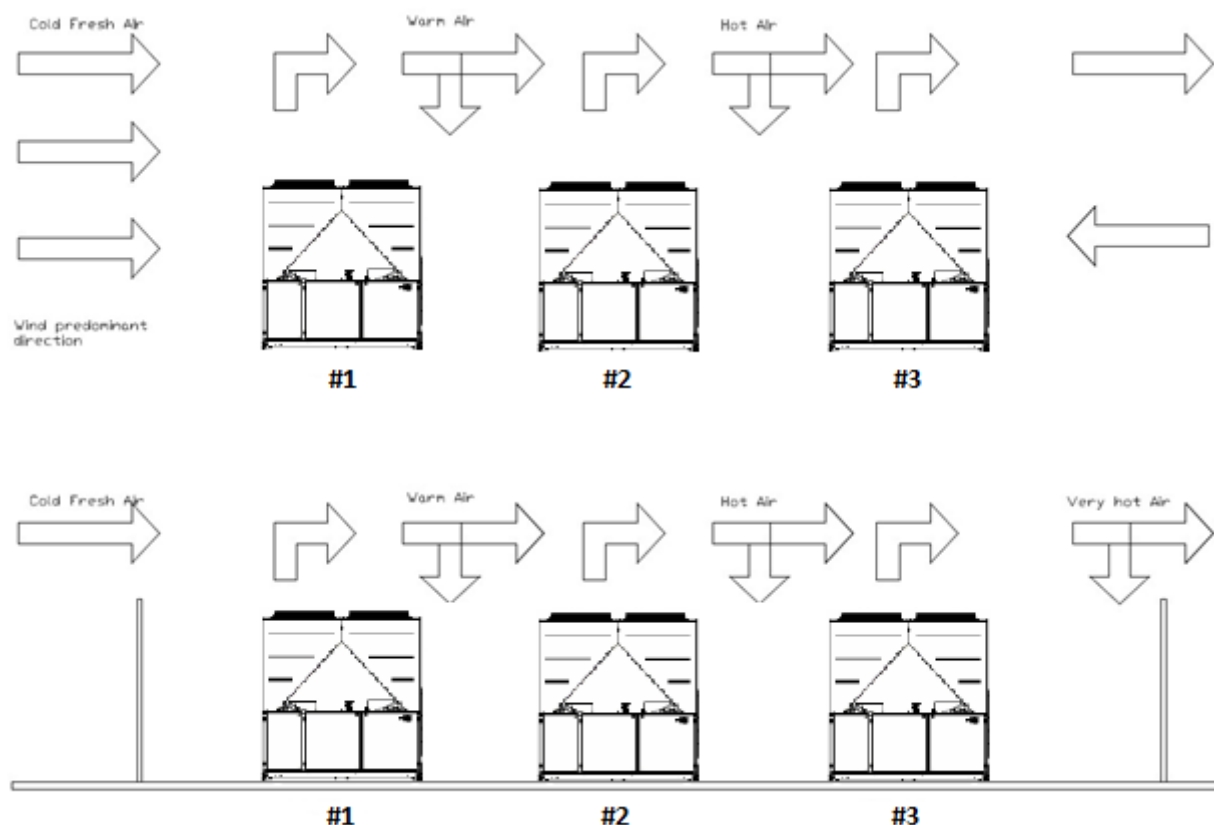
Рис. 17. Монтаж нескольких агрегатов (режим охлаждения)
