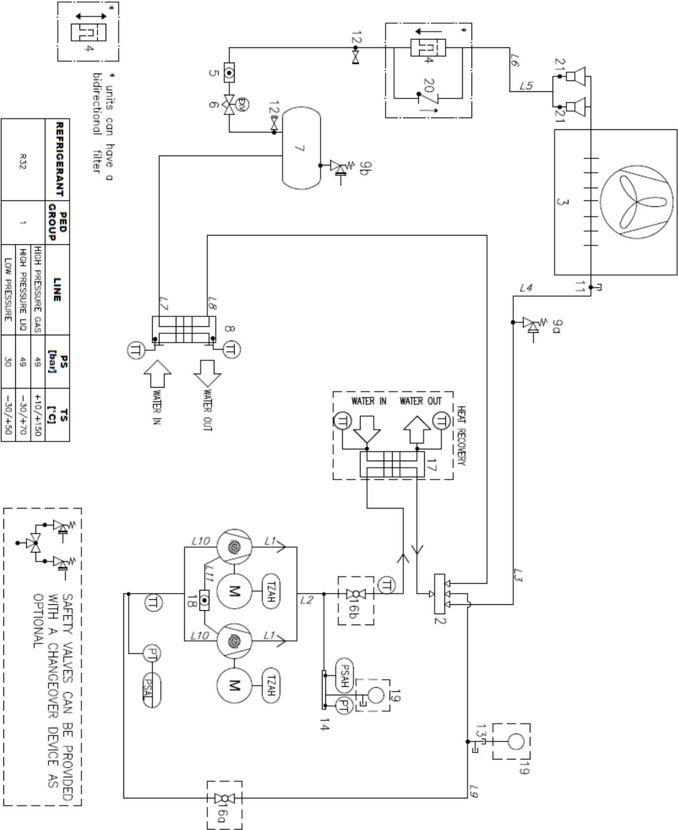
Рис. 1. Схема трубопровода хладагента (схема трубопроводов и КИП) для одноконтурного агрегата EWYTx5B
