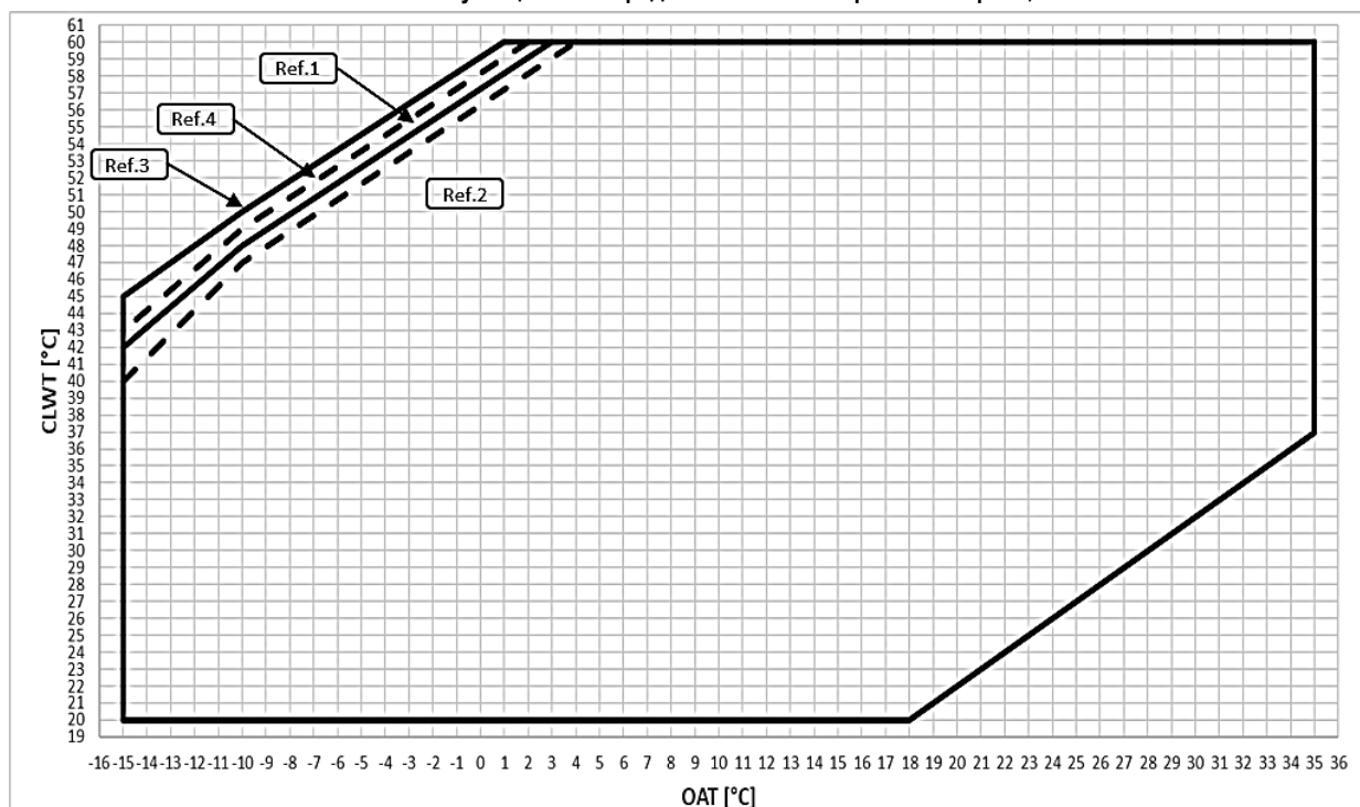
Рис. 13. Эксплуатационные пределы EWYT-B-X в режиме нагрева, OP.204
