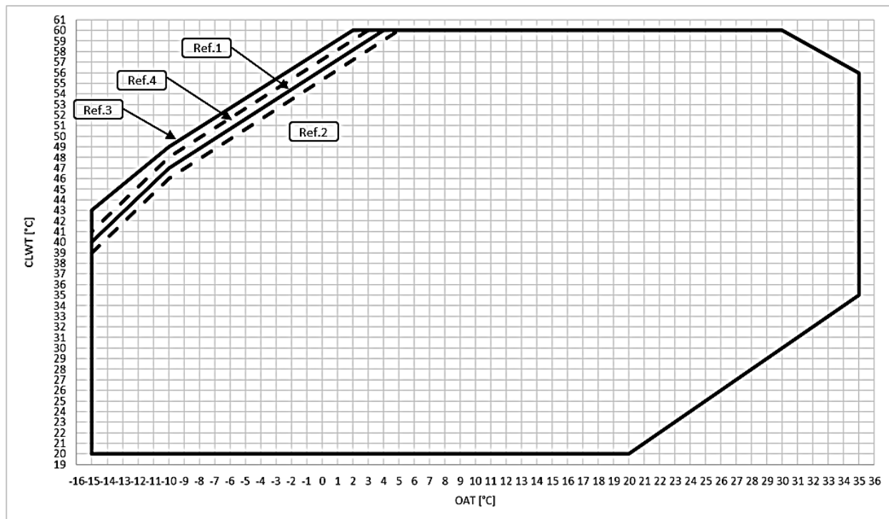
Рис. 12. Эксплуатационные пределы EWYT~В-S в режиме нагрева, ОР.204
