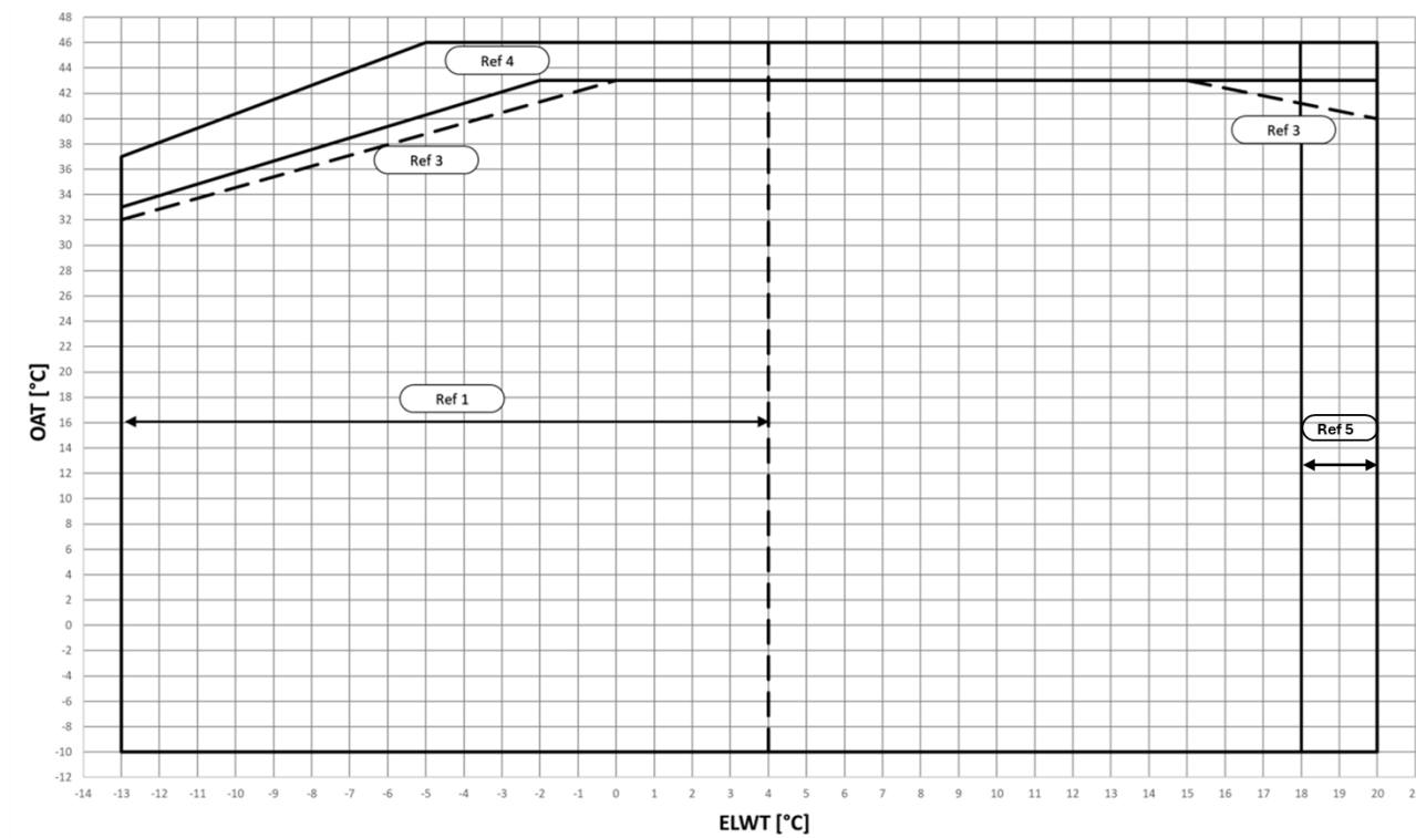
Рис. 6. Эксплуатационные пределы EWYTxh5B-S в режиме охлаждения
