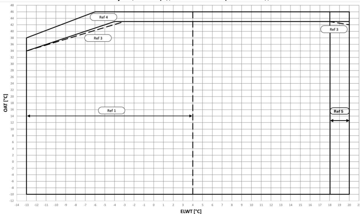
Рис. 7. Эксплуатационные пределы EWYTxh5B-X в режиме охлаждения
