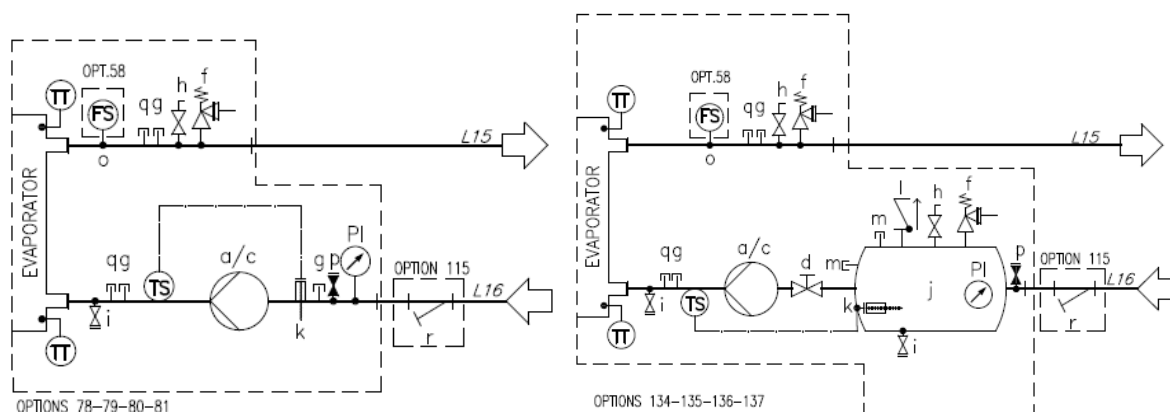
Рис. 24. Гидравлическая схема для одного насоса / двух насосов (компл. 78-79-80-81/134-135-136-137) (макс. рабочее давление 6 бар)
