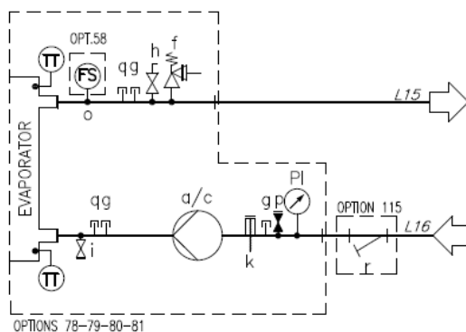
Рис. 22. Гидравлическая схема для одного насоса / двух насосов с баком (EWYTxh5B) (компл. 134-135) (макс. рабочее давление 6 бар)
