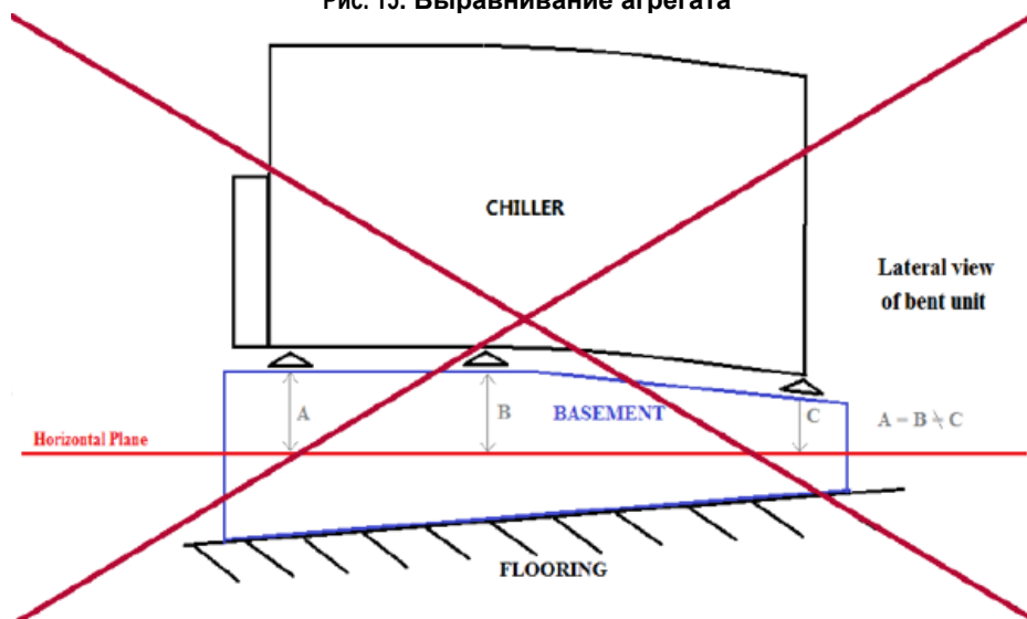
Рис. 15. Выравнивание агрегата
