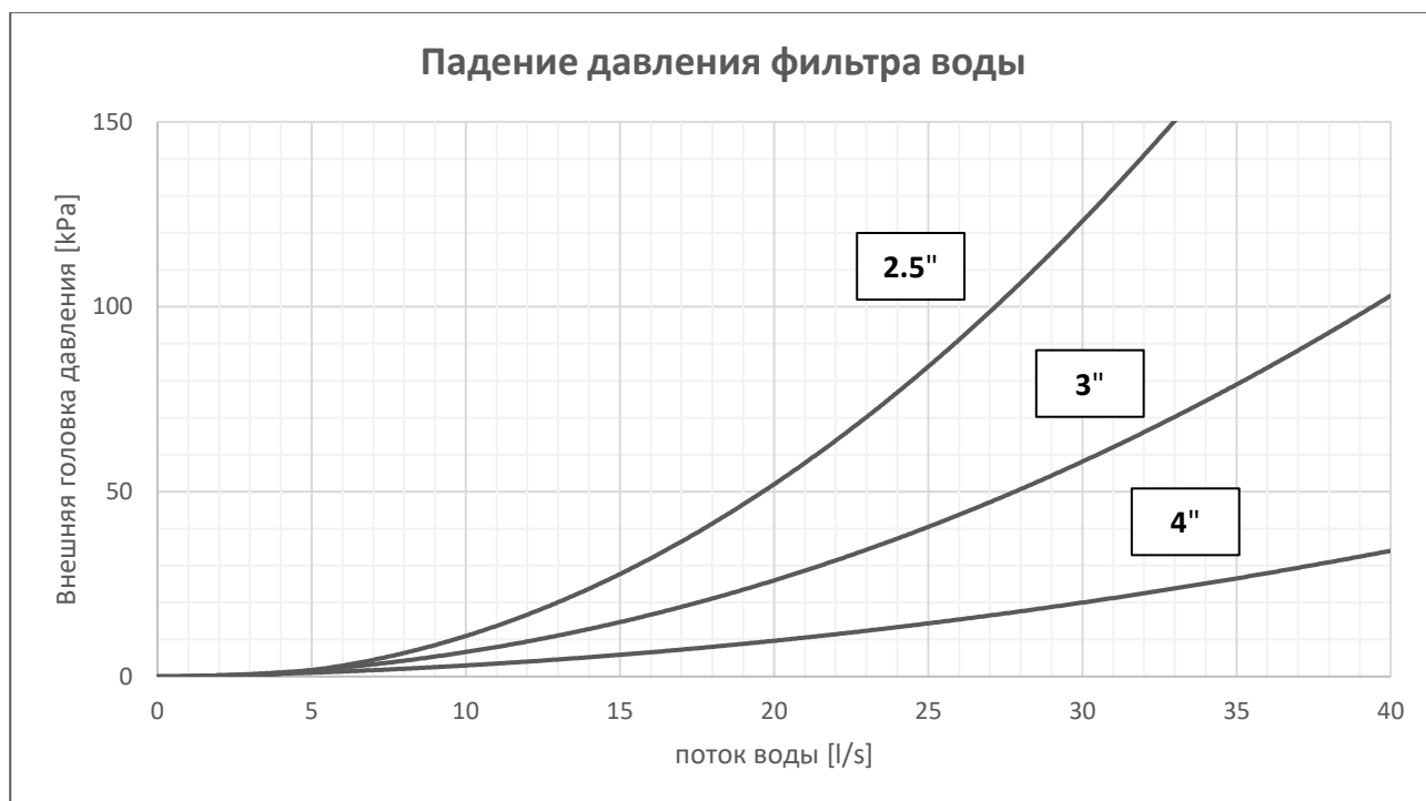
Рис. 18. Перепад давления на фильтре для воды
