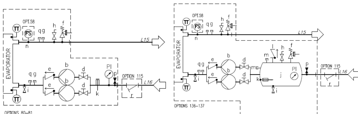
Рис. 23. Гидравлическая схема для сдвоенного насоса (EWYTxh5B) (компл. 80-81/136-137) (макс. рабочее давление 6 бар)
