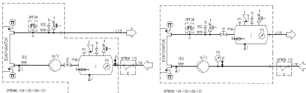
Obr. 22 – Hydraulická schéma samostatného čerpadla/dvojitého čerpadla s nádržou (EWYTx5B) (možnosť 134 – 135) (max. prevádzkový tlak 6 barov)
