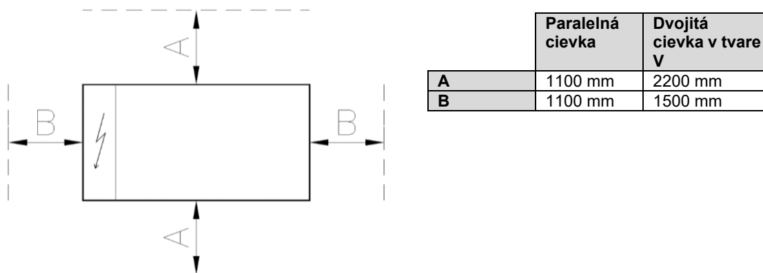
Obr. 16 – Minimálne požiadavky na priestor
