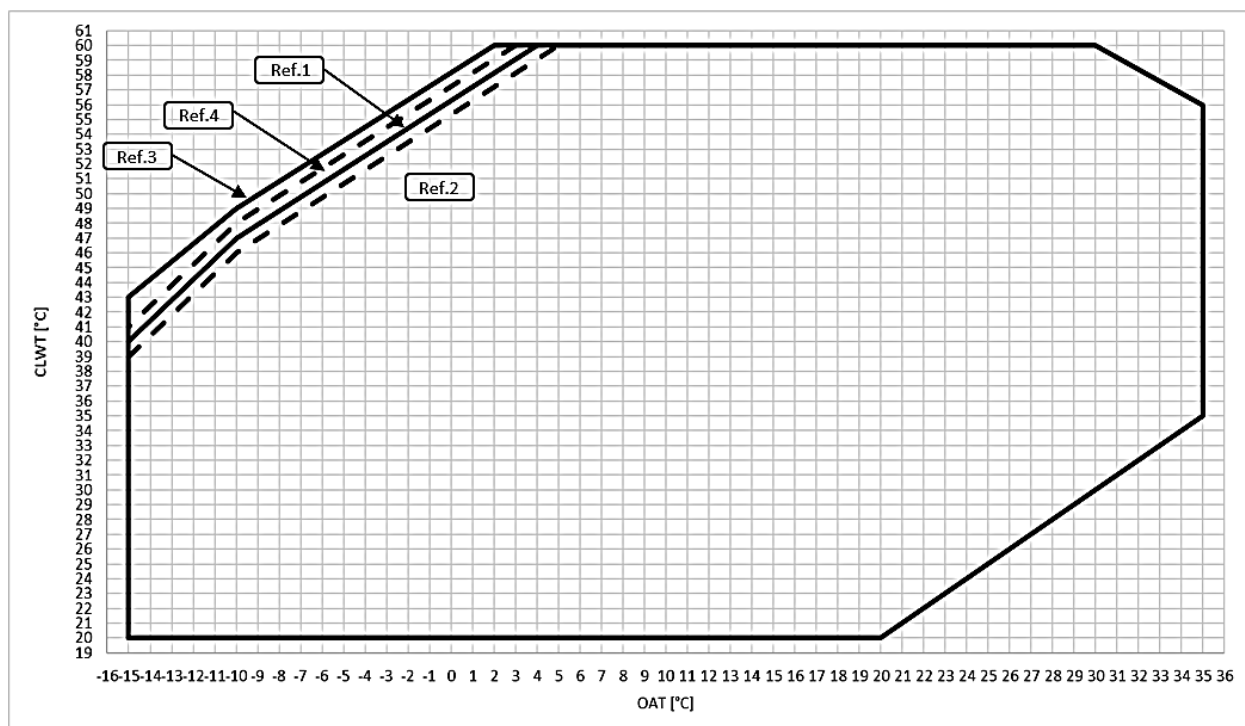
Obr. 13 – Prevádzkové limity režimu ohrevu EWYT~B-X – OP.204
