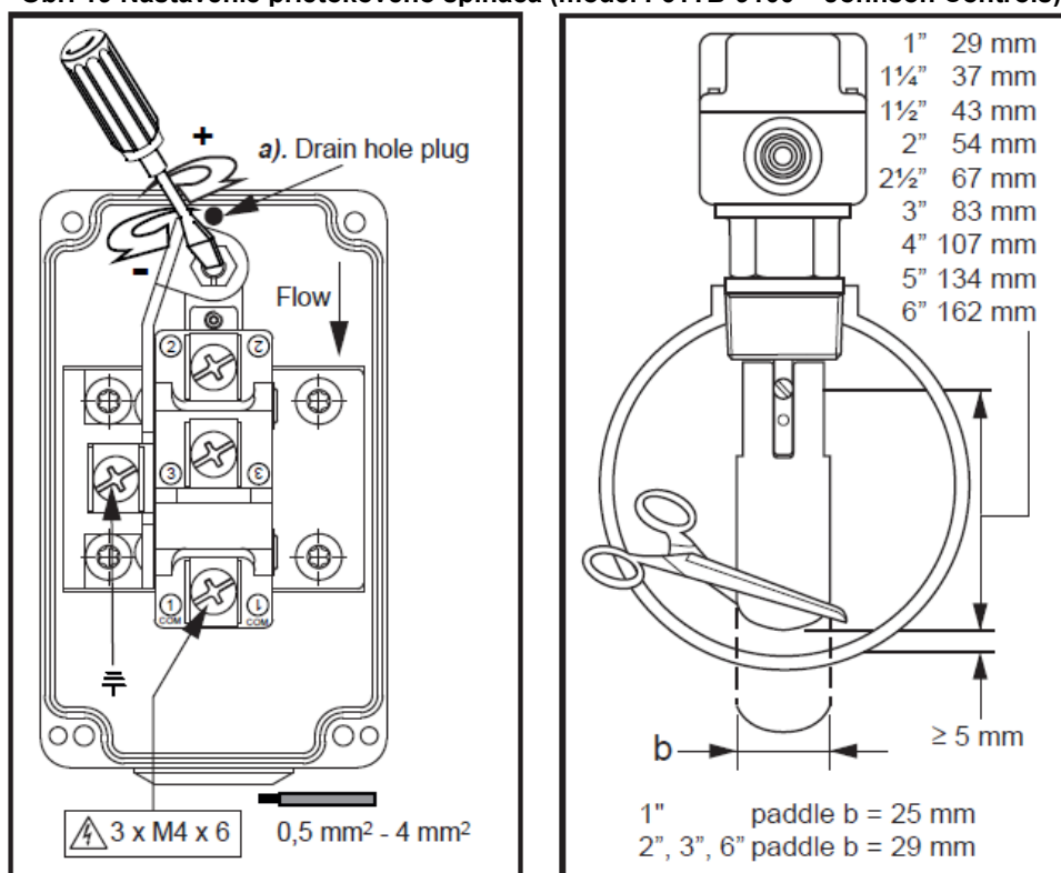
Obr. 19 Nastavenie prietokového spínača (model F61TB-9100 – Johnson Controls)
