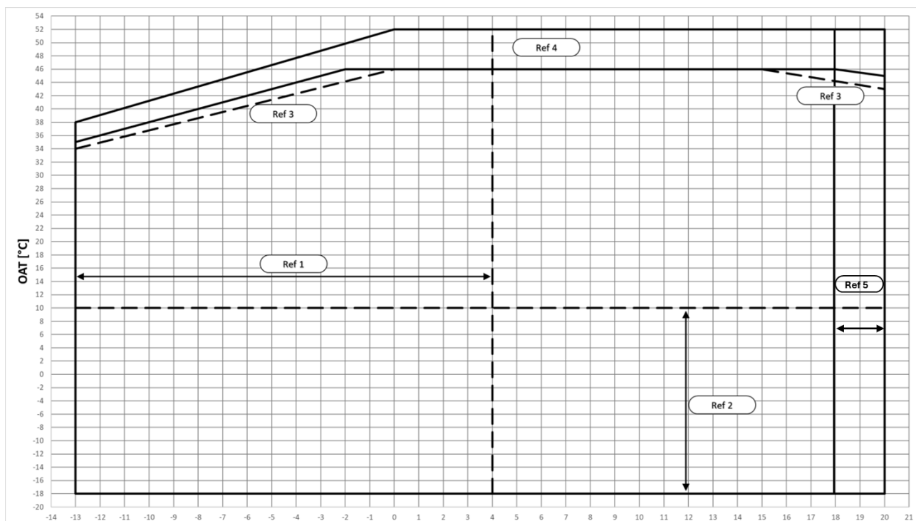
Obr. 9 – Prevádzkové limity režimu chladenia EWYTx0B-X
