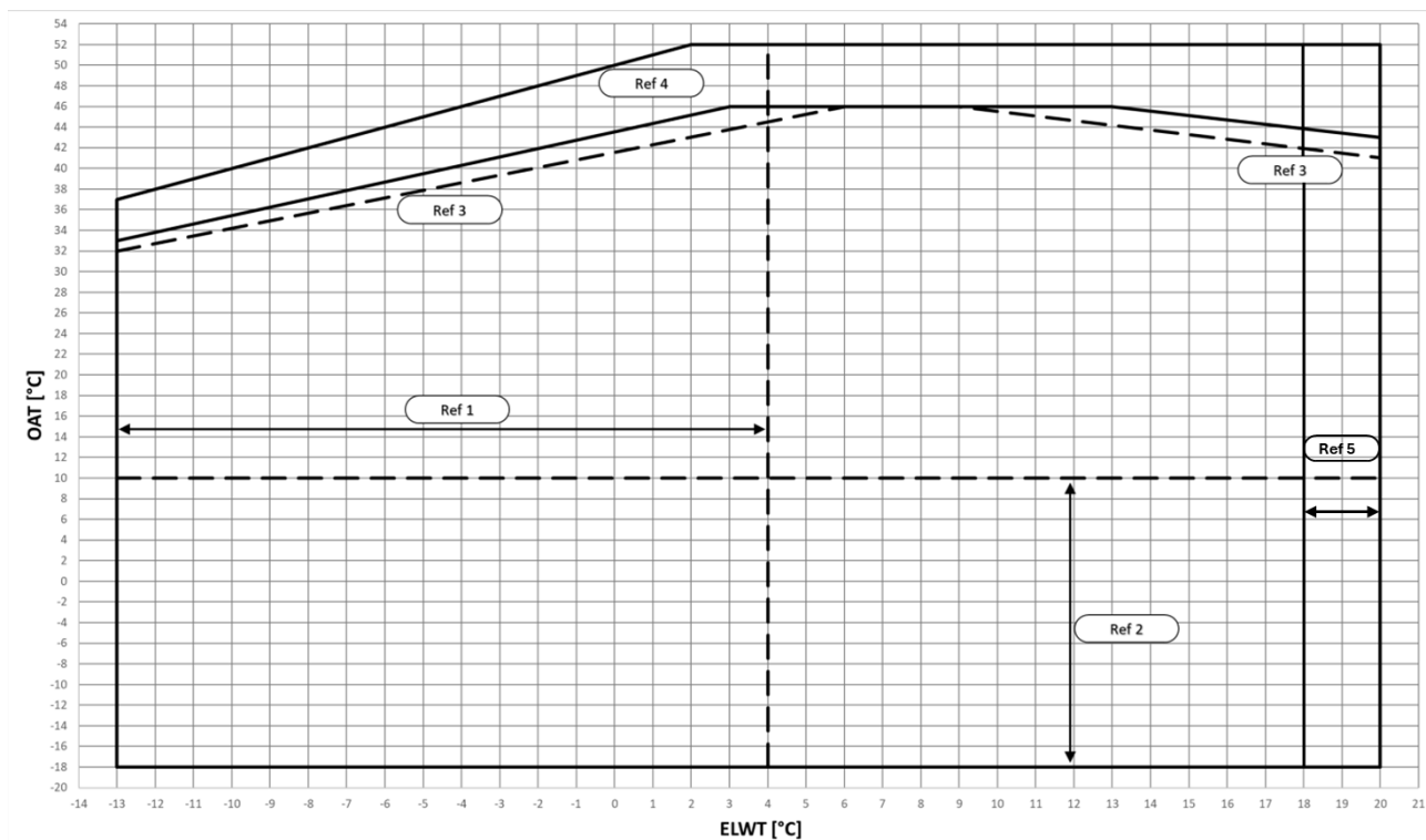
Obr. 9 – Prevádzkové limity režimu chladenia EWYTx0B-X
