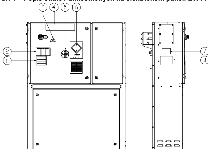
Obr. 4 – Popis štítkov umiestnených na elektrickom paneli EWYTx5B
