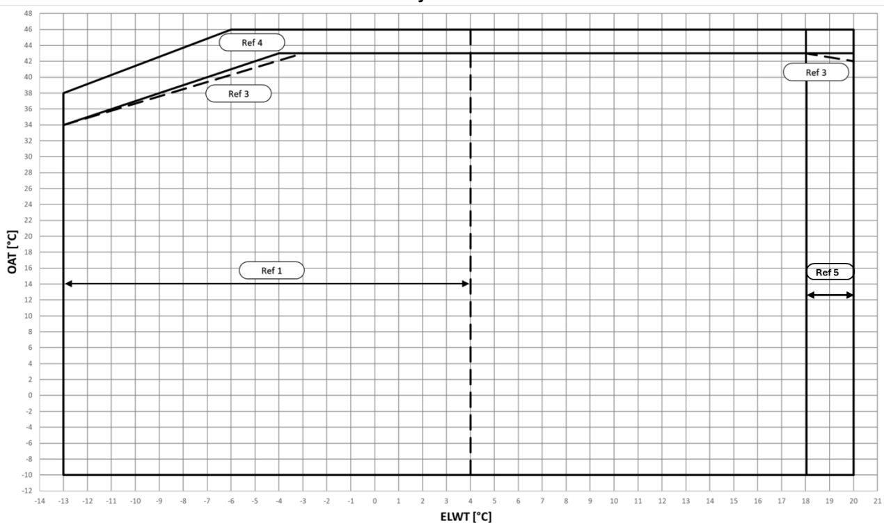
Obr. 7 – Prevádzkové limity režimu chladenia EWYTxx5B-X
