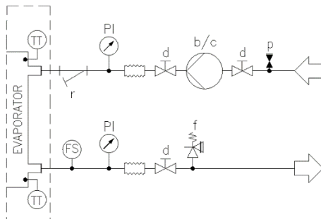
Obr. 21 – Hydraulická schéma samostatného čerpadla/dvojitého čerpadla (EWYTx5B) (možnosť 78 – 79) (max. prevádzkový tlak 6 barov)
