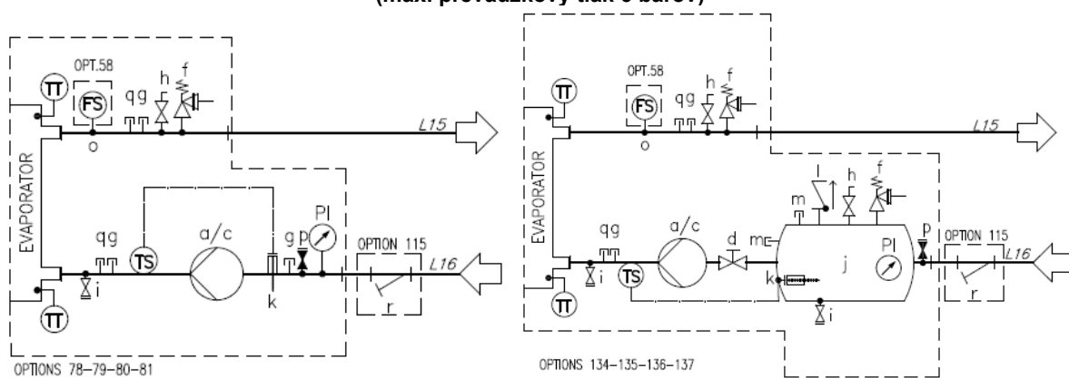
Obr. 24 – Hydraulická schéma samostatného čerpadla/dvojitého čerpadla (opt. 78-79-80-81/134-135-136-137) (max. prevádzkový tlak 6 barov)
