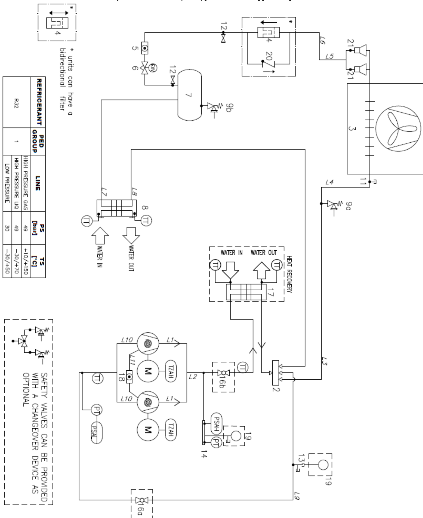
Obr. 1 – Schéma potrubia chladiva (P&ID) jednookruhovej jednotky EWYTxx5B
