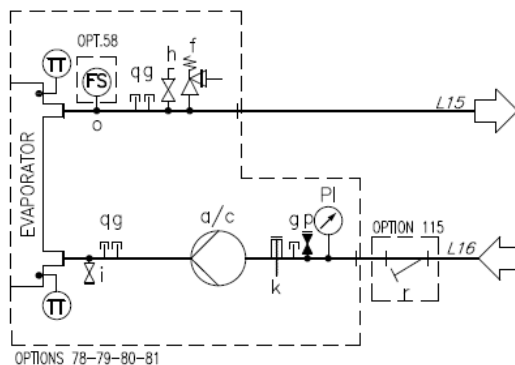
Obr. 21 – Hydraulická schéma samostatného čerpadla/dvojitého čerpadla (EWYTx5B) (možnosť 78 – 79) (max. prevádzkový tlak 6 barov)
