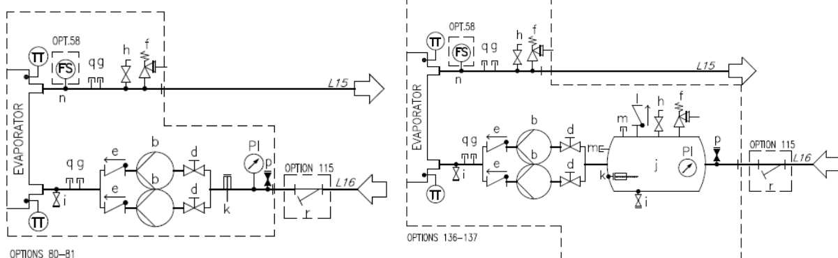
Obr. 23 – Hydraulická schéma dvojitého čerpadla (EWYTxx5B) (možnosť 80 – 81/136 – 137) (max. prevádzkový tlak 6 barov)
