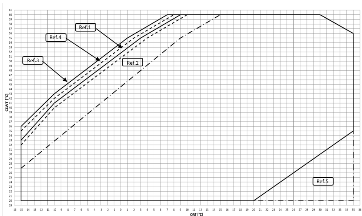
Obr. 11 – Prevádzkové limity režimu ohrevu EWYT~B-X
