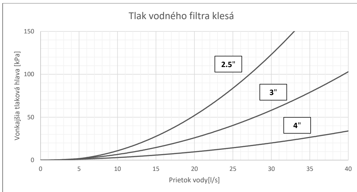
Obr. 18 – Pokles tlaku vodného filtra
