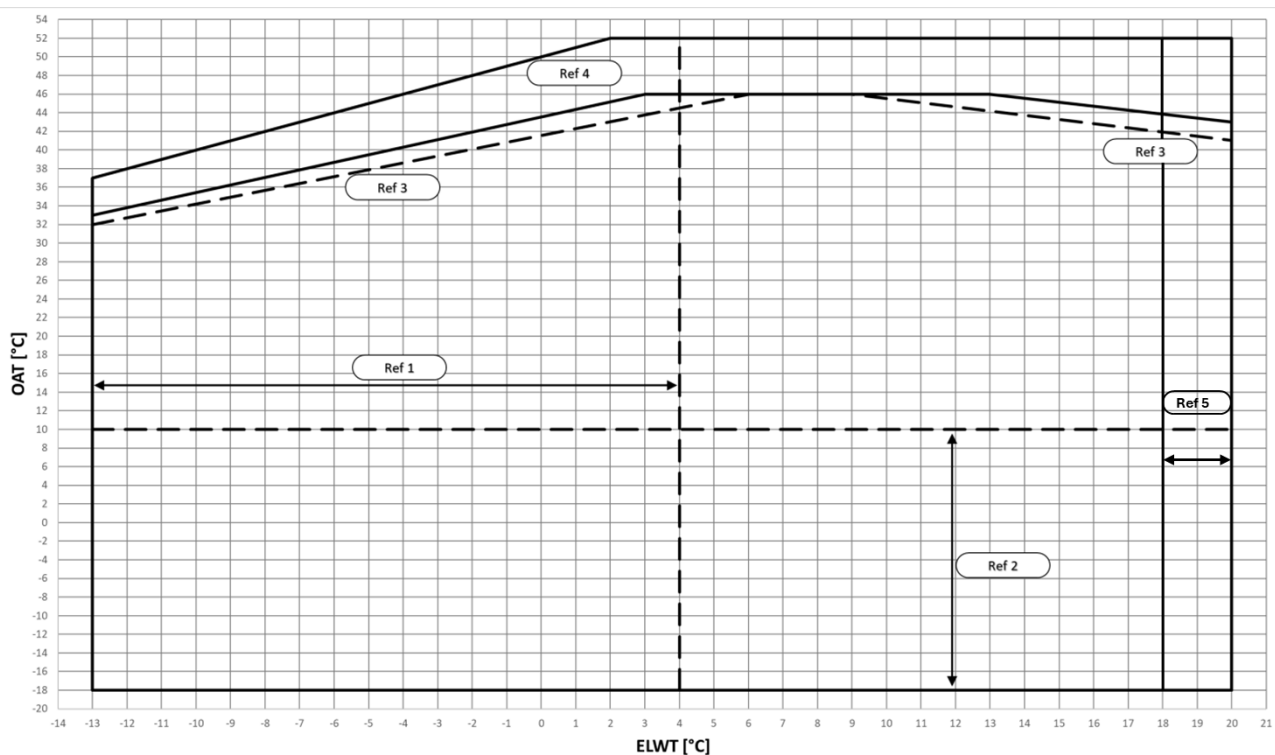
Slika 8 – EWYTx0B-S Delovne omejitve načina hlajenja
