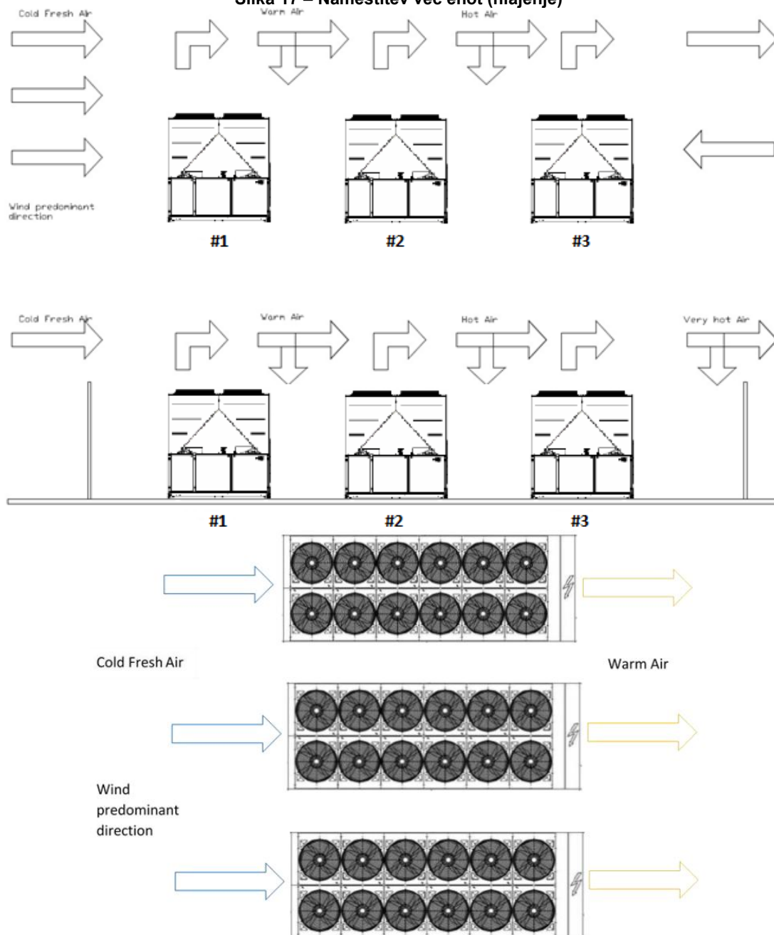
Slika 17 – Namestitev več enot (hlajenje)
