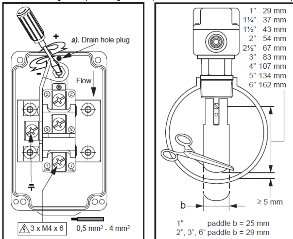
Slika 19 – Prilagoditev pretočnega stikala (model F61TB-9100 – Johnson Controls)
