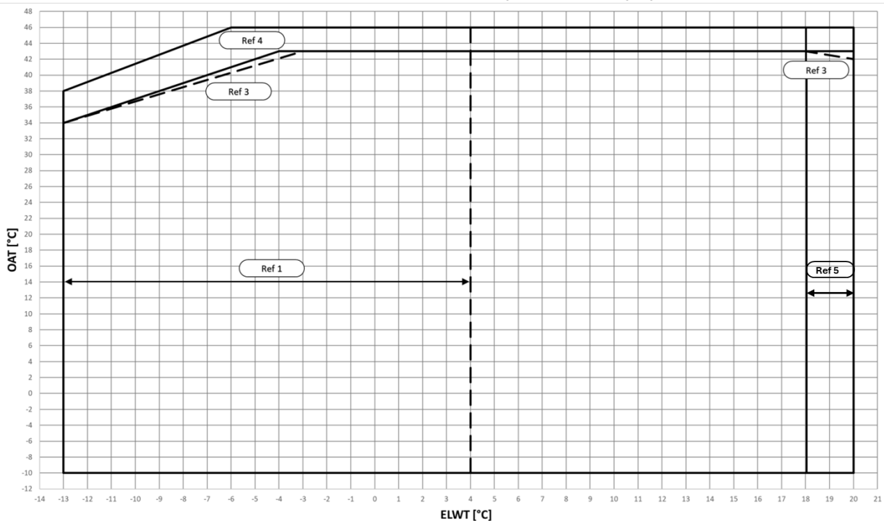
Slika 7 – EWYTx5B-X Delovne omejitve načina hlajenja
