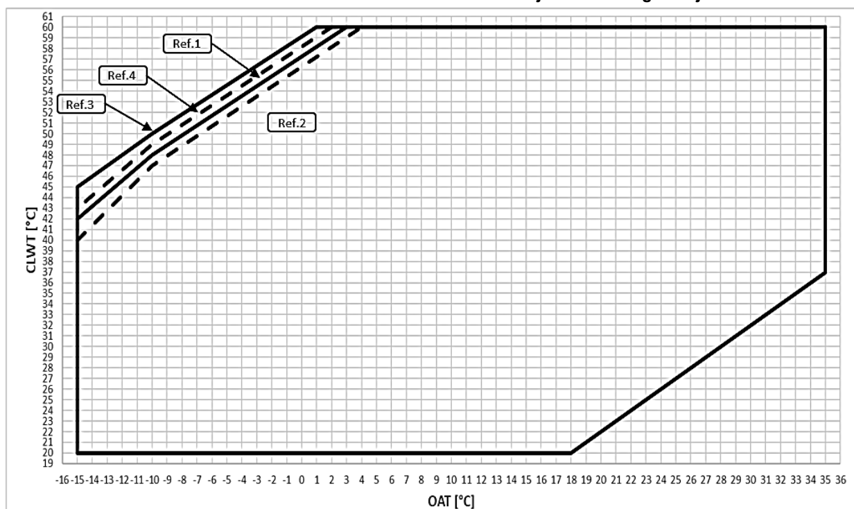
Slika 13 – EWYT ~B-X – OP.204 Delovne omejitve načina ogrevanja
