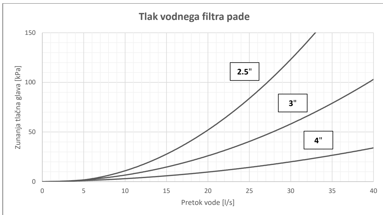
Slika 18 – Padec tlaka vodnega filtra
