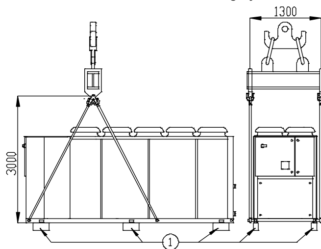
Enota s 4 dvignimi točkami
