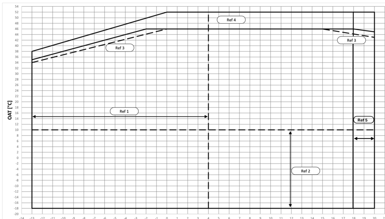
Slika 9 – EWYTxx0B-X Delovne omejitve načina hlajenja
