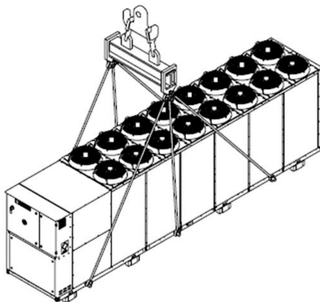
Enota s 6 dvignimi točkami
