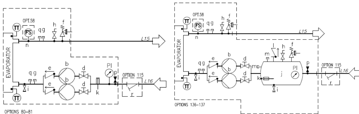
Slika 23 – Hidravlična shema za dvojno črpalko (EWYTx5B) (opc. 80-81/136-137) (maks. delovni tlak 6 barov)
