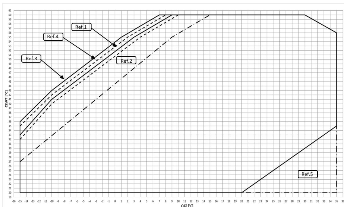
Slika 10 – EWYT ~B-S Delovne omejitve načina ogrevanja
