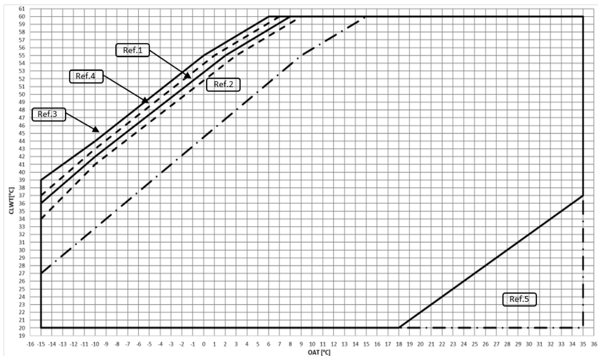
Slika 11 – EWYT ~ B-X Delovne omejitve načina ogrevanja
