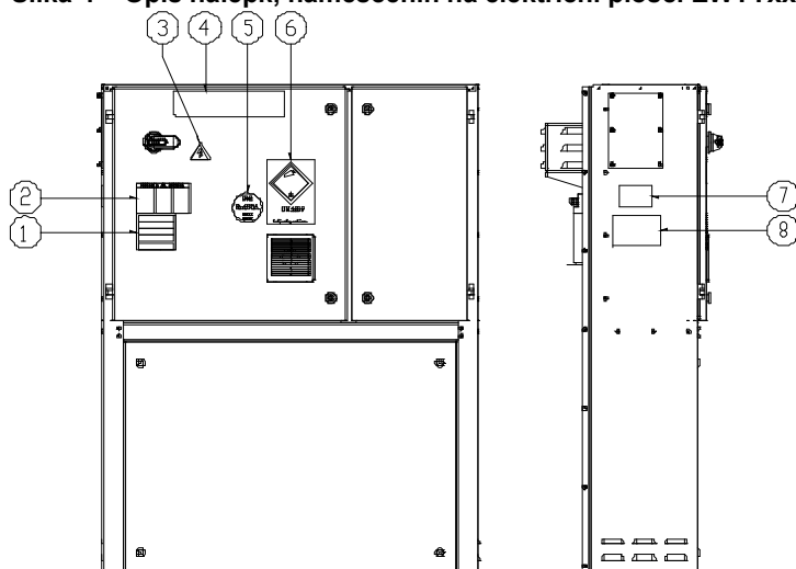
Slika 4 – Opis nalepk, nameščenih na električni plošči EWYTxx5B
