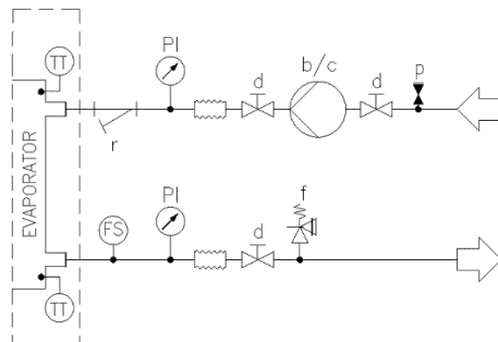
Slika 21 – Hidravlični diagram za eno črpalko / dvojno črpalko (EWYTx5B) (opc. 78-79) (maks. delovni tlak 6 barov)
