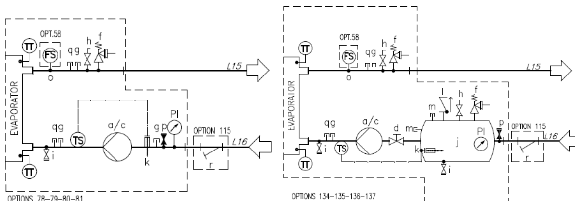
Slika 24 – Hidravlični diagram za eno črpalko / dvojno črpalko (opc. 78-79-80-81/134-135-136-137) (maks. delovni tlak 6 barov)
