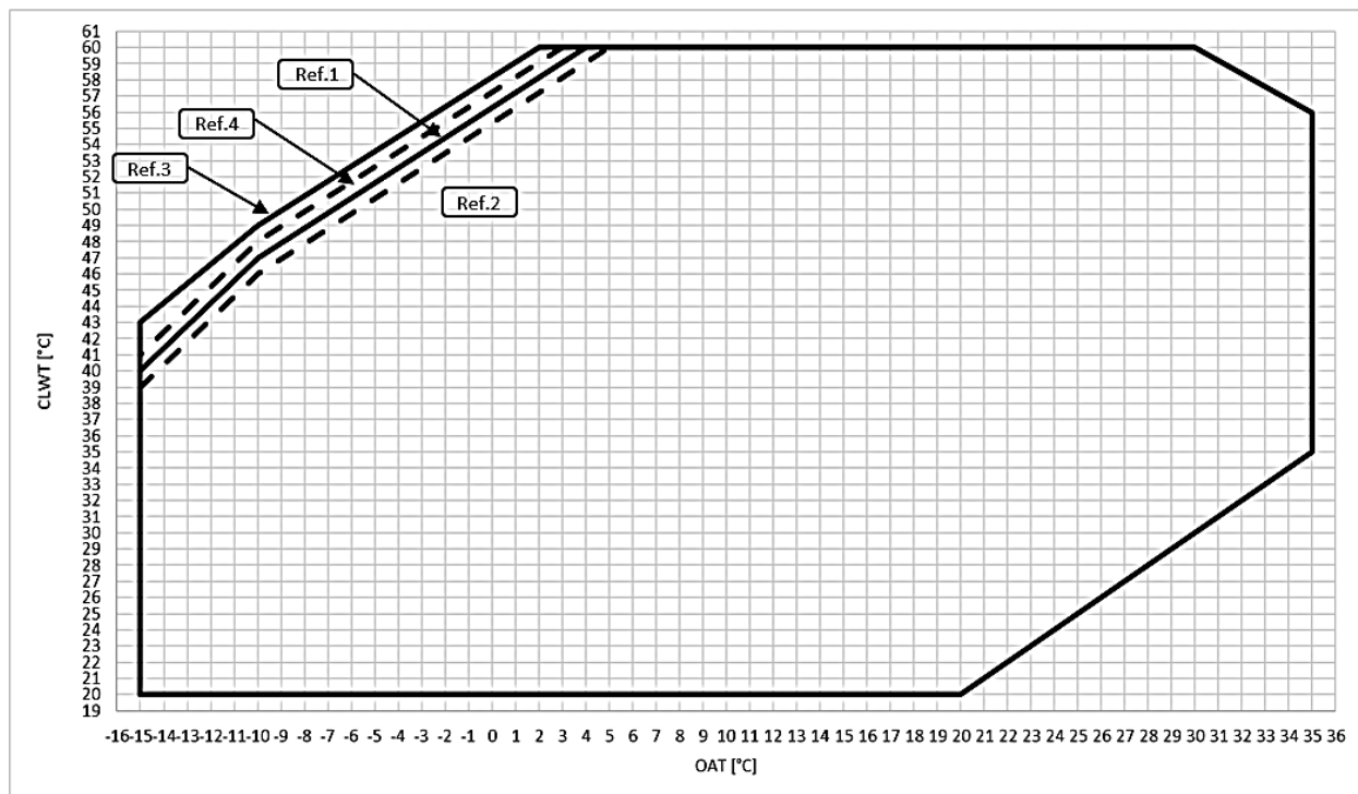
Slika 12 – EWYT ~B-S – OP.204 Delovne omejitve načina ogrevanja
