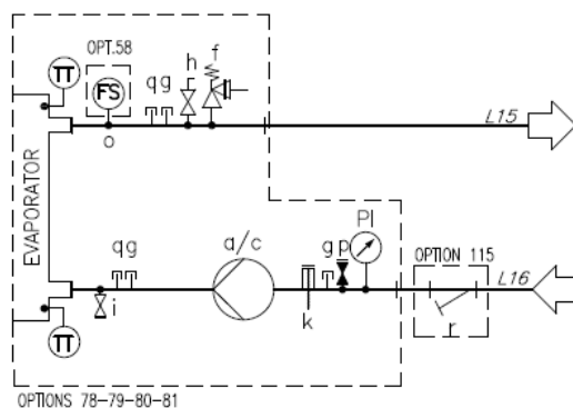
Slika 22 – Hidravlična shema za eno črpalko / dvojno črpalko z rezervoarjem (EWYTx5B) (opc. 134-135) (maks. delovni tlak 6 barov)
