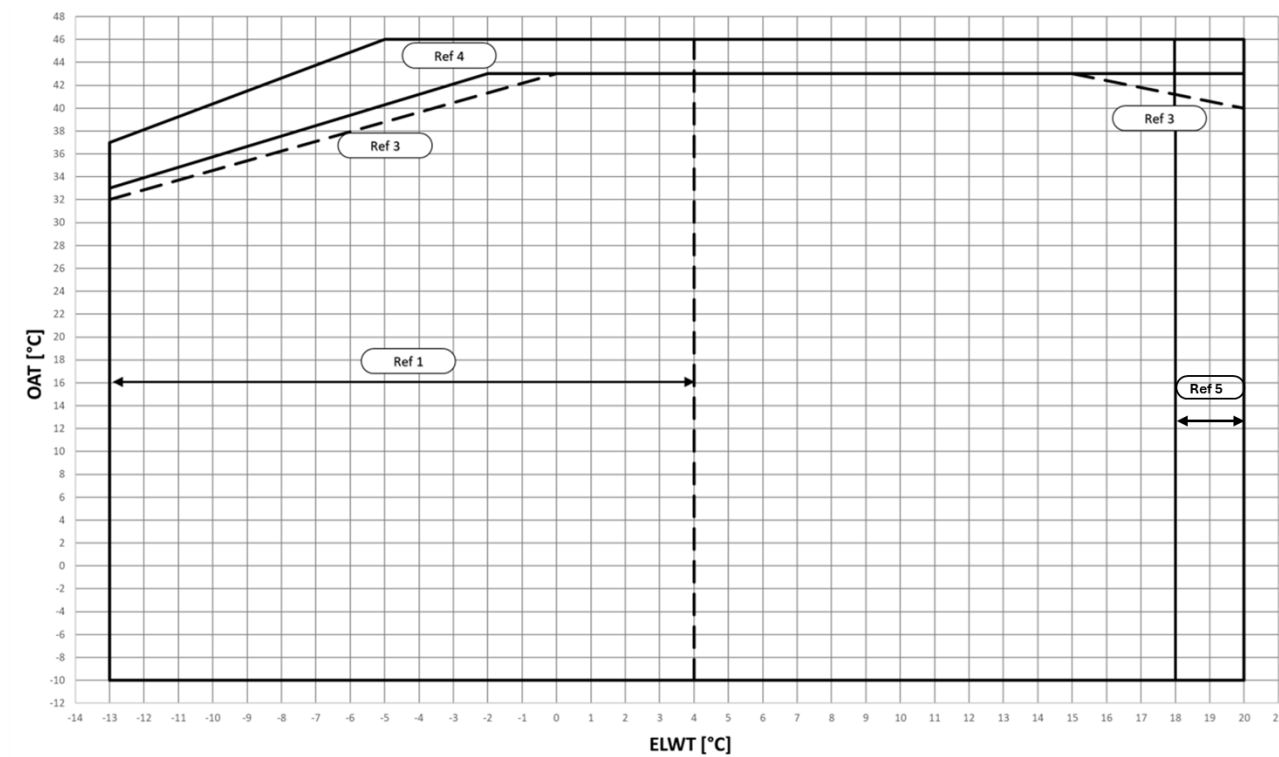
Slika 6 – EWYTx5B-S Delovne omejitve hladilnega načina
