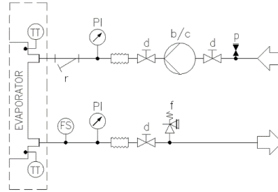
Fig.20– Diagrama hidraulike pa pompa në bord (presioni maksimal i funksionimit 20 bar)
