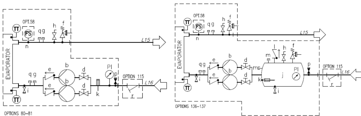
Fig.23– Diagrami hidraulik për pompën e dyfishtë (EWYTx5B) (opt. 80-81/136-137) (presioni maksimal i funksionimit 6 bar)
