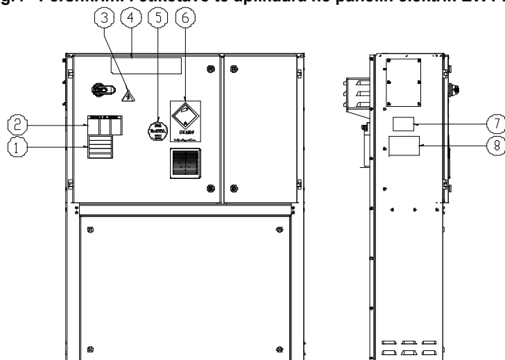
Fig.4– Përshkrimi i etiketave të aplikuara në panelin elektrik EWYTxx5B
