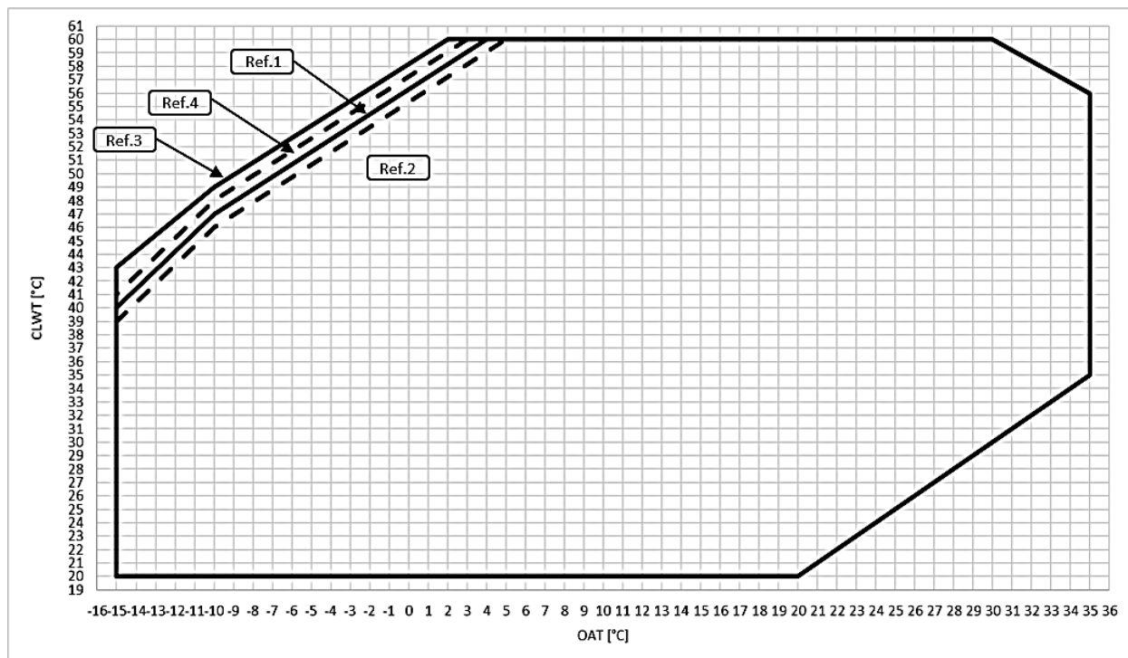
Fig.12– EWT~BS – OP.204 Kufijtë e funksionimit të modalitetit të ngrohjes
