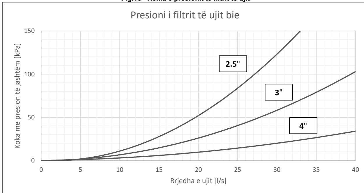
Fig.18– Rënia e presionit të filtrit të ujit
