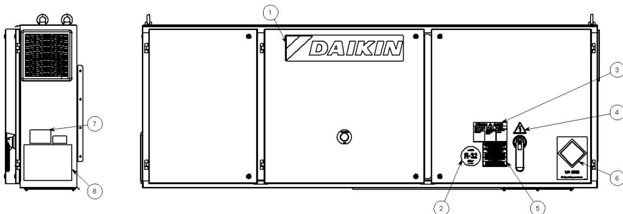
Fig.5– Përshkrimi i etiketave të aplikuara në panelin elektrik EWYTxx0B
