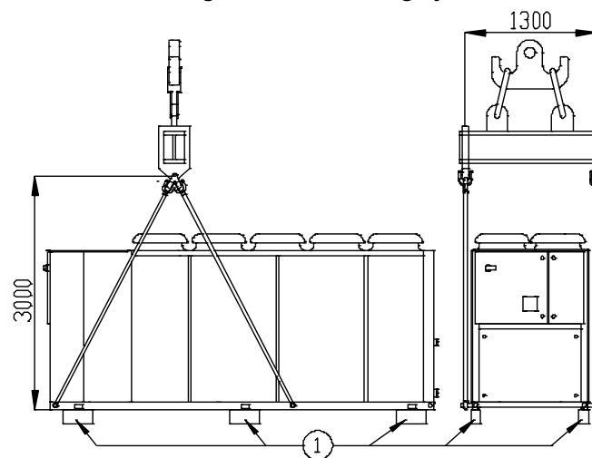
Fig.14-Udhëzimet e ngritjes
