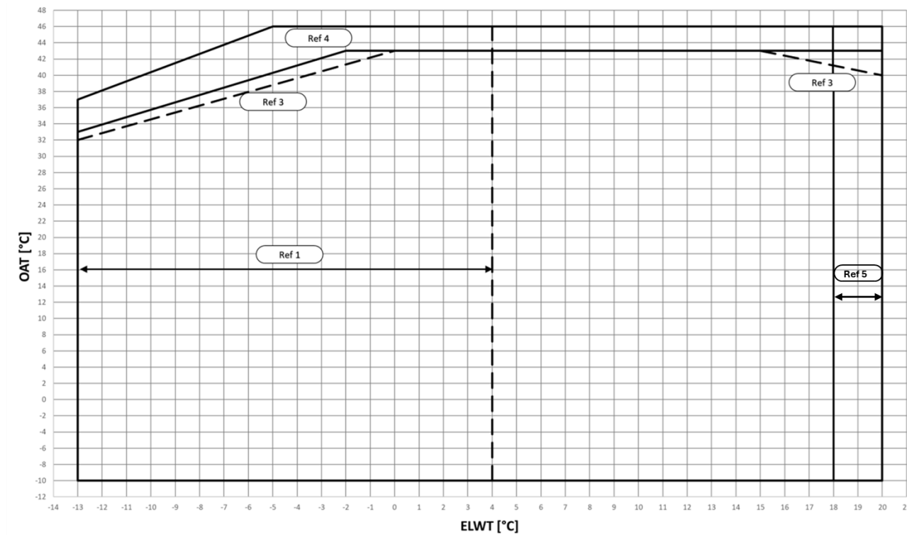
Fig.6– Kufijtë e funksionimit të modalitetit të ftohjes EWYTxx5B-S
