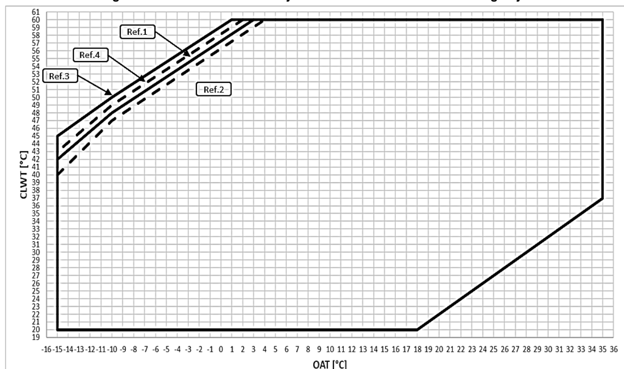
Fig.13– EWYT~BX – OP.204 Kufijtë e funksionimit të modalitetit të ngrohjes
