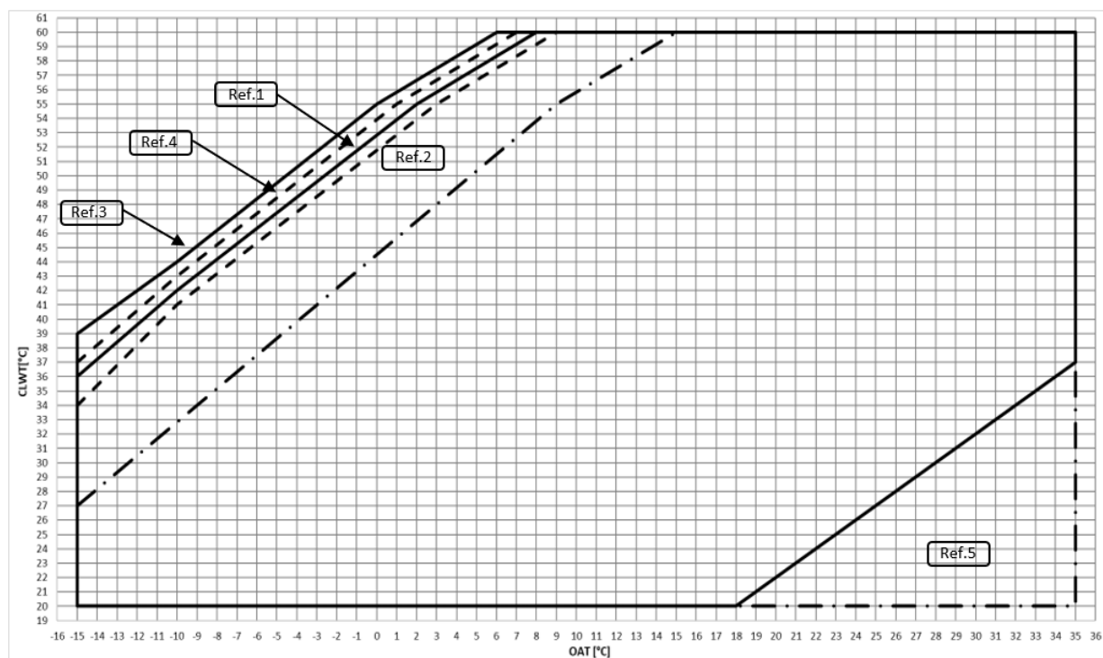
Fig.11– Kufijtë e funksionimit të modalitetit të ngrohjes EWT~BX
