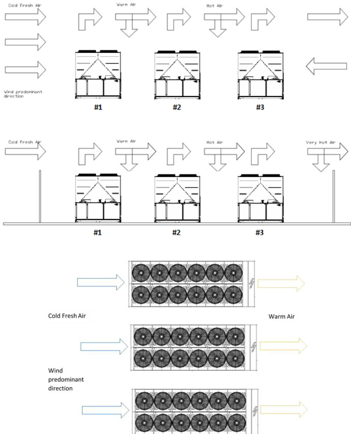
Fig.17– Instalimi i shumë njësive (modaliteti i ftohjes)
