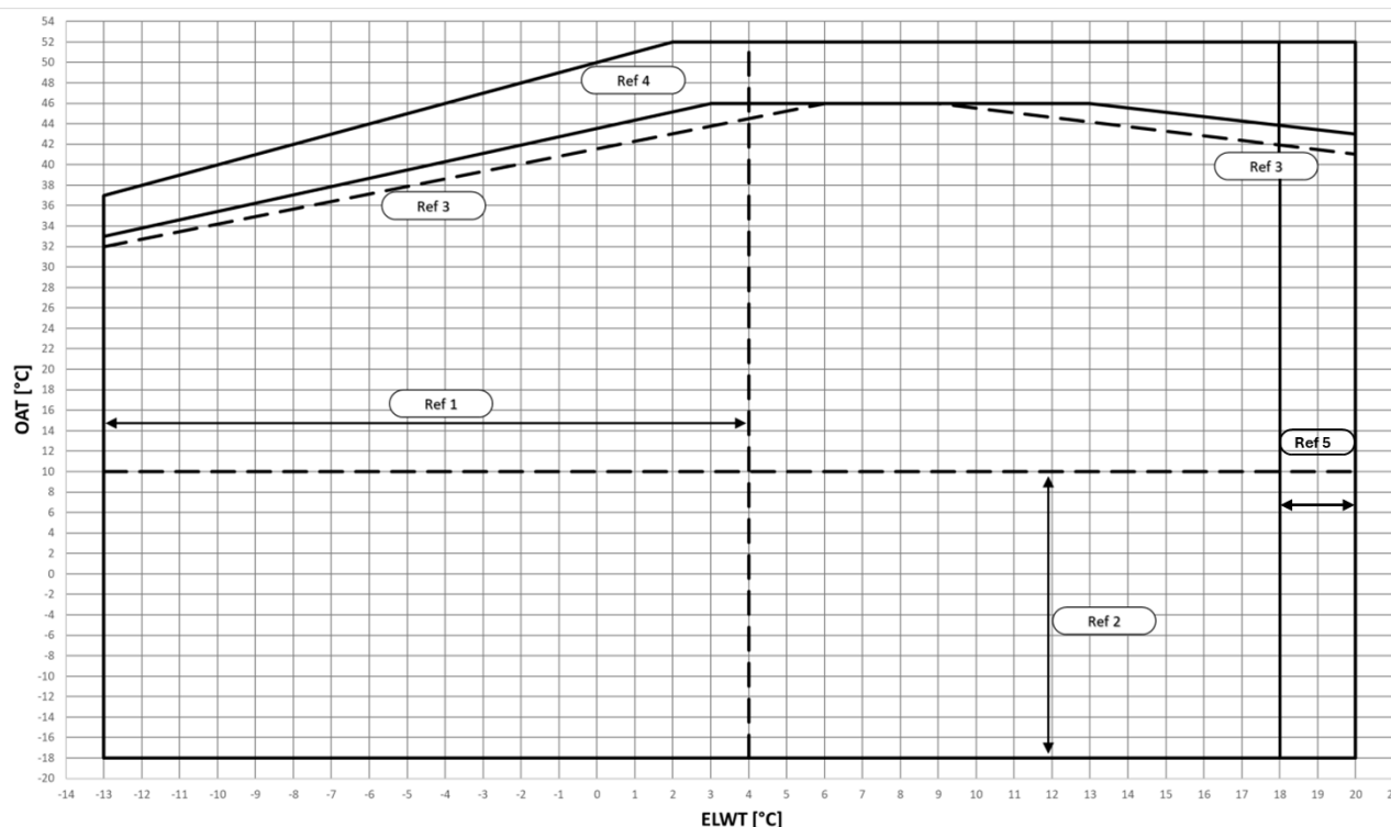
Fig.8– Kufijtë e funksionimit të modalitetit të ftohjes EWYTx0B-S
