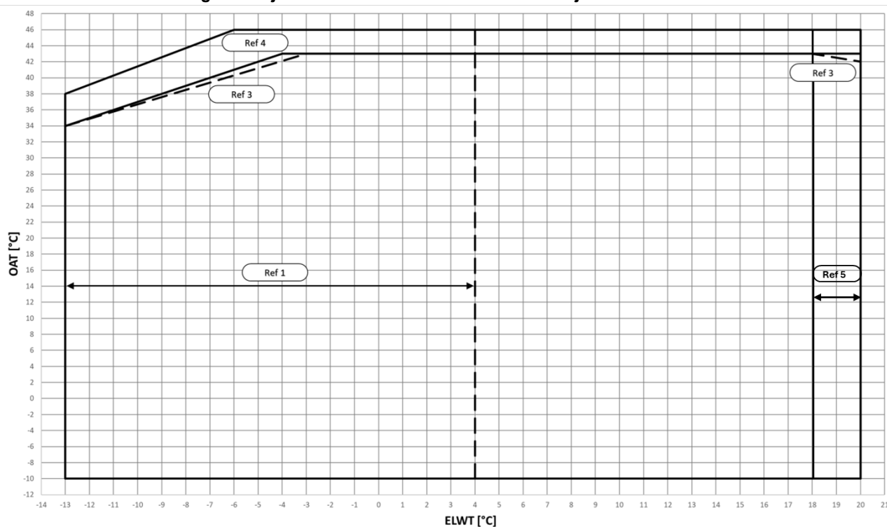
Fig.7– Kufijtë e funksionimit të modalitetit të ftohjes EWYTx5B-X
