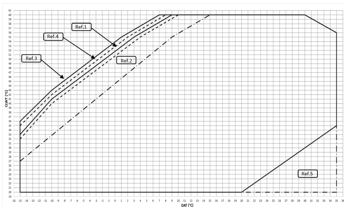
Fig.10– Kufijtë e funksionimit të modalitetit të ngrohjes EWYT~BS
