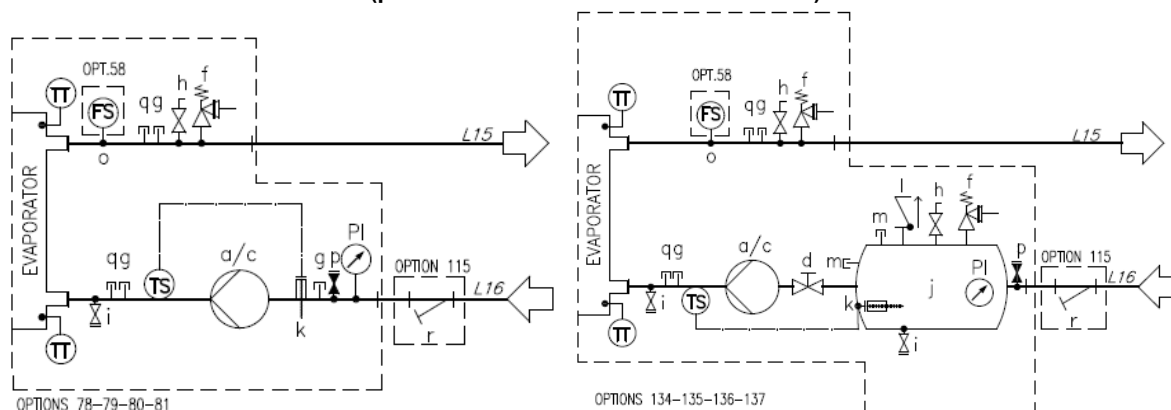
Fig.24– Diagrami hidraulik për një pompë të vetme / pompë dyshe (opt. 78-79-80-81/134-135-136-137) (presioni maksimal i funksionimit 6 bar)
