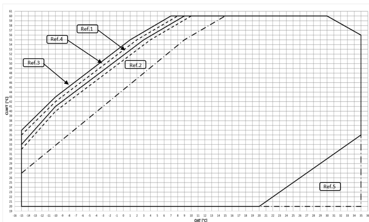
Fig. 10 – EWYT~B-S Operativa gränser för uppvärmningsläge
