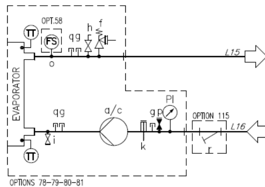
Fig. 22 – Hydrauliska schema för enkelpump / dubbelpump med tank (EWYTx5B) (alt. 134-135) (max arbetstryck 6 bar)
