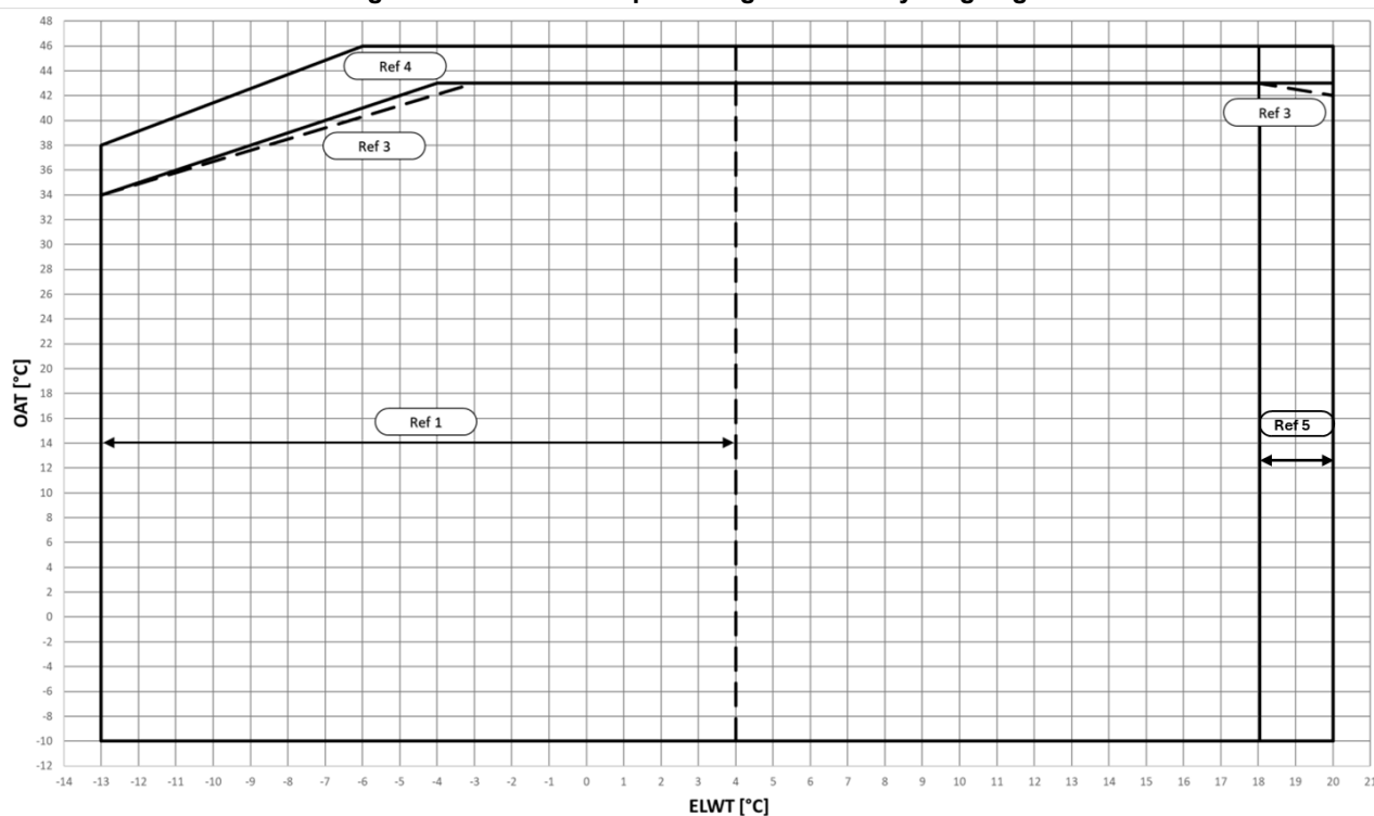
Fig. 7 – EWYTx5B-X Operativa gränser för kylningsläge
