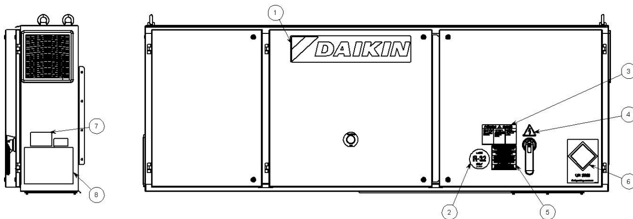
Fig. 5 – Beskrivning av märkningarna applicerade på elpanelen EWYTx0B
