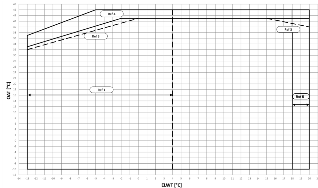
Fig. 6 – EWYTxx5B-S Operativa gränser för kylningsläge
