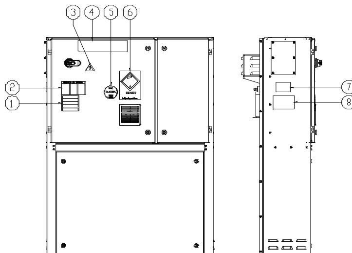
Fig. 4 – Beskrivning av märkningarna applicerade på elpanelen EWYTx5B
