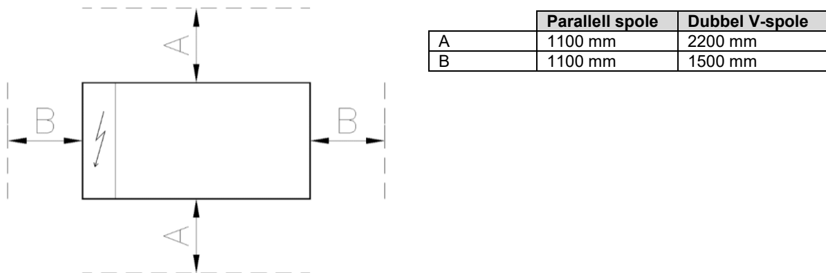
Fig. 16 – Krav på minsta utrymme
