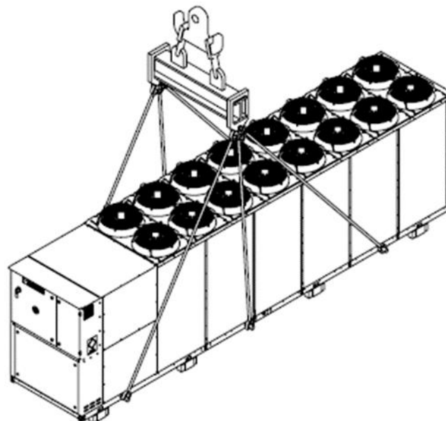
Enhet med 6 lyftpunkter
