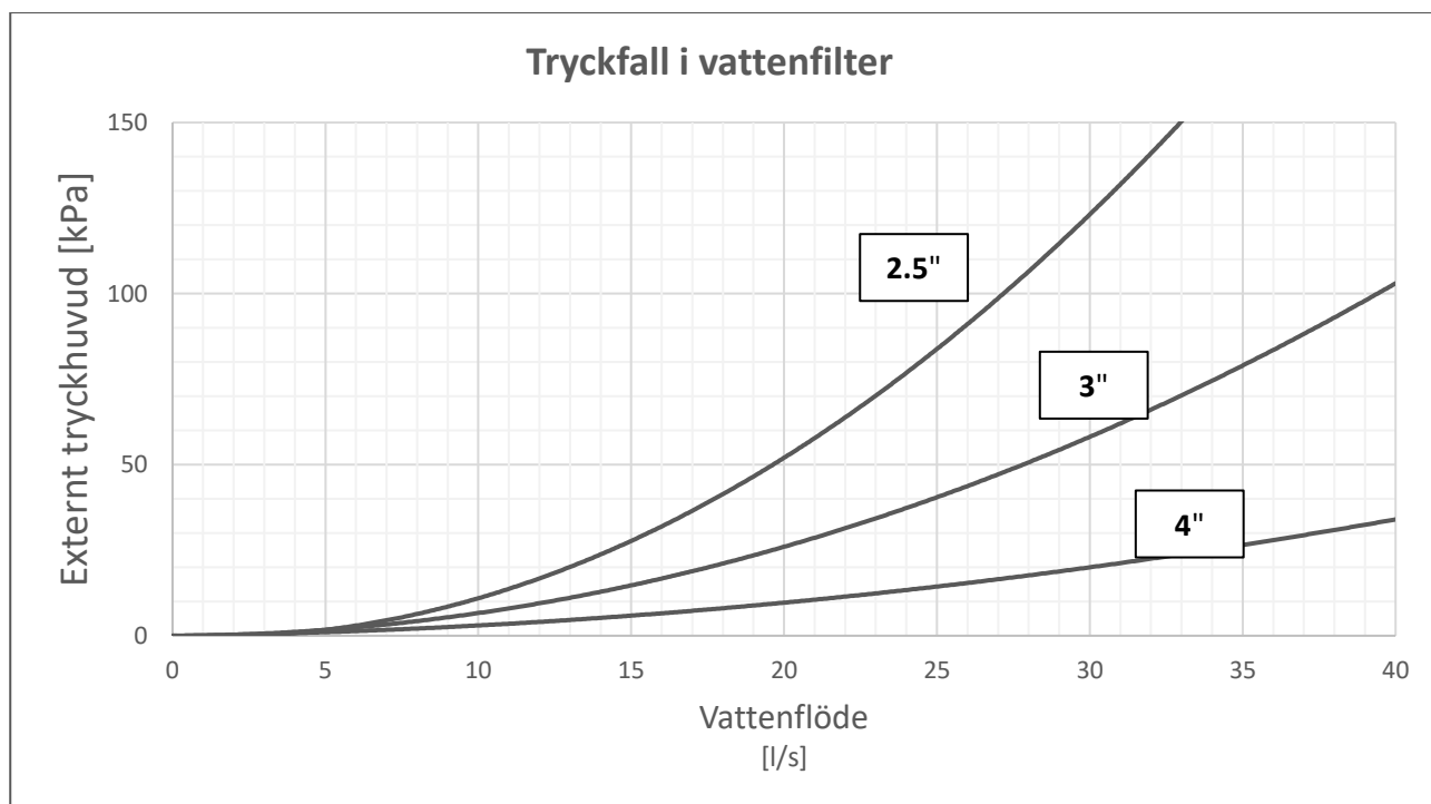
Fig. 18 – Tryckfall i vattenfilter
