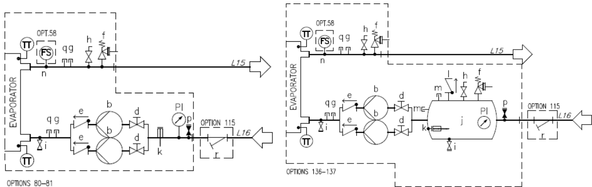
Fig. 23 – Hydrauliskt diagram för dubbelpump (EWYTx5B) (alt. 80-81/136-137) (max arbetstryck 6 bar)
