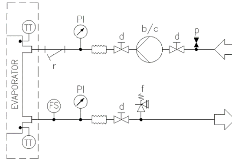
Fig. 21 – Hydrauliskt diagram för enkelpump / dubbelpump (EWYTx5B) (alt. 78-79) (max arbetstryck 6 bar)
