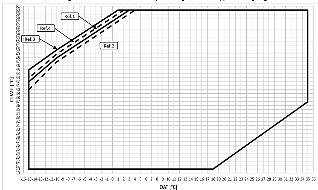
Fig. 13 – EWYT~B-X – OP.204 Operativa gränser för uppvärmningsläge
