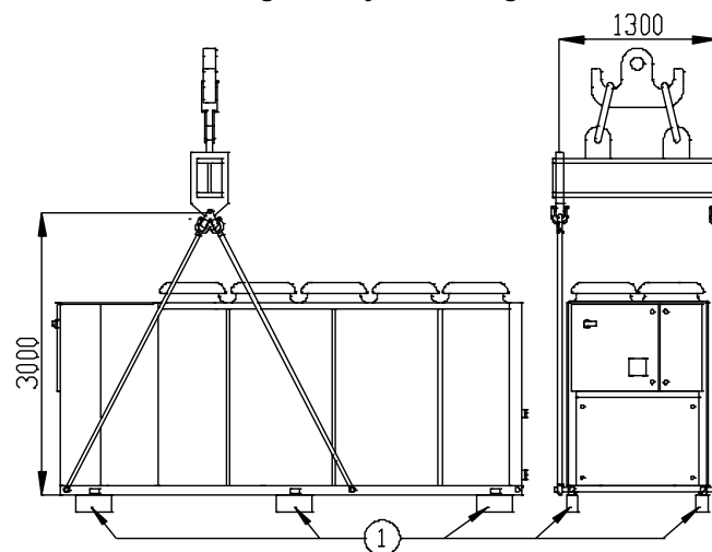
Enhet med 4 lyftpunkter
