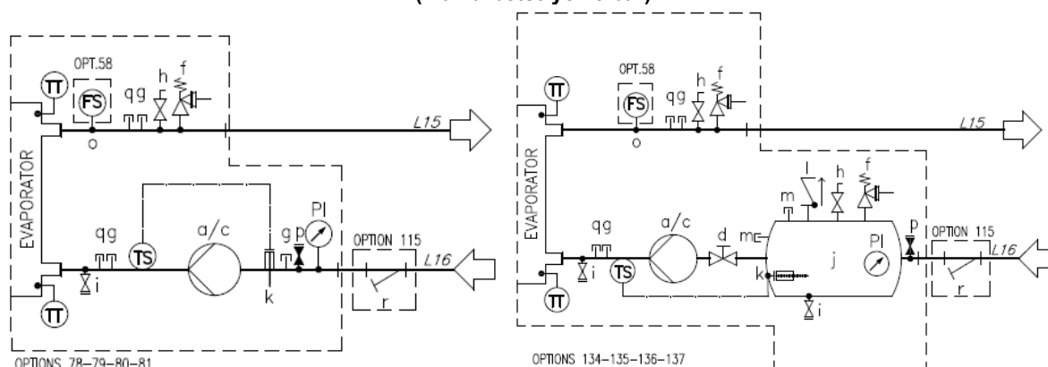
Fig. 24 – Hydrauliskt diagram för enkelpump / dubbelpump (alt. 78-79-80-81/134-135-136-137) (max arbetstryck 6 bar)
