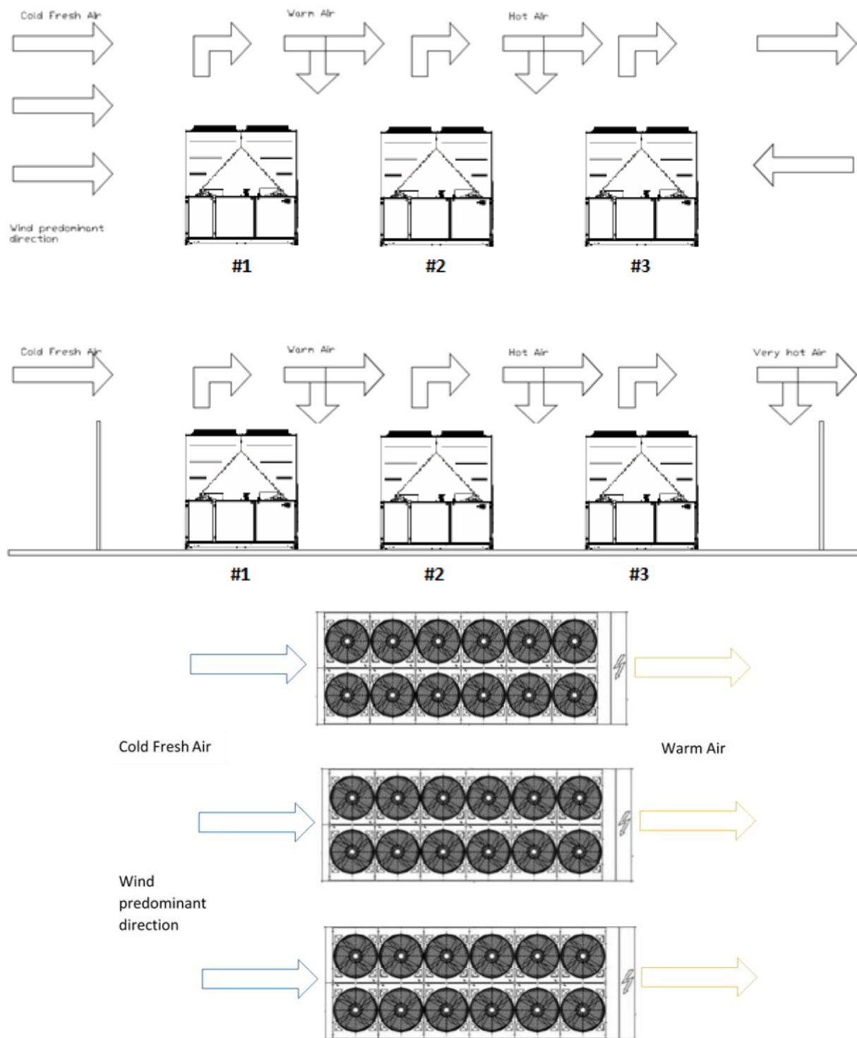
Fig. 17 – Installation av flera kylare
