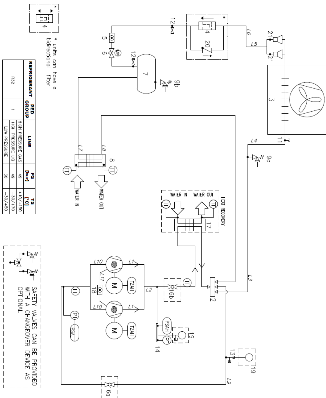
Fig. 1 – Kylkretsdiagram EWYTx5B standard enkelkretsenshet (P&ID)
