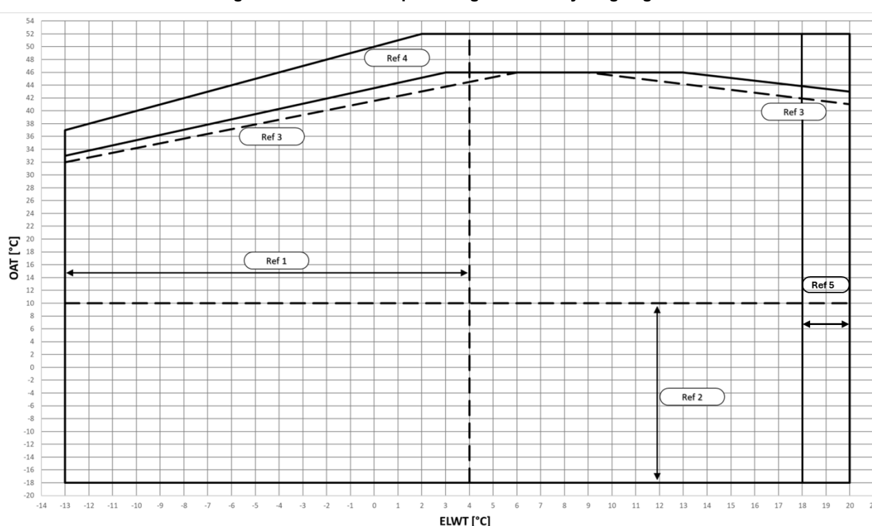
Fig. 8 – EWYTx0B-S Operativa gränser för kylningsläge
