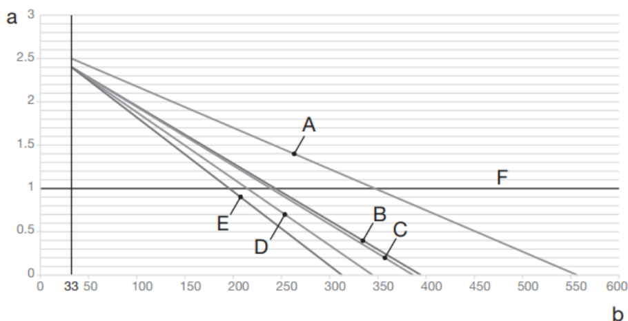
Obrázek 17 - Počáteční tlak expanzní nádoby podle maximálního objemu vody
