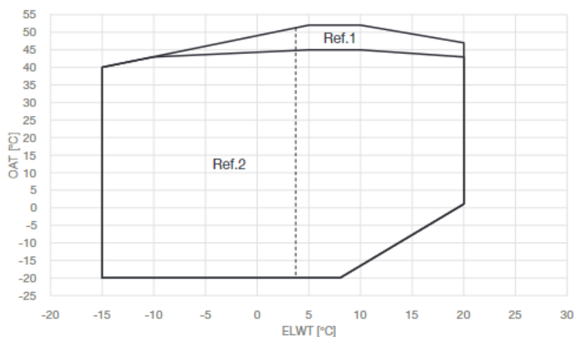
Εικόνα 15 - Όρια λειτουργίας στο EWT-CZ σε λειτουργία ψύξης
