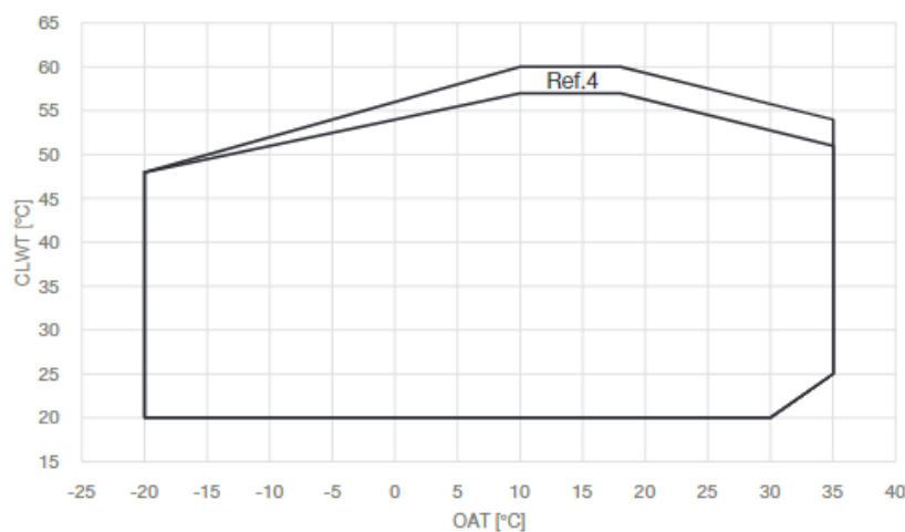
Εικόνα 16 - Όρια λειτουργίας στο EWT-CZ σε λειτουργία θέρμανσης
