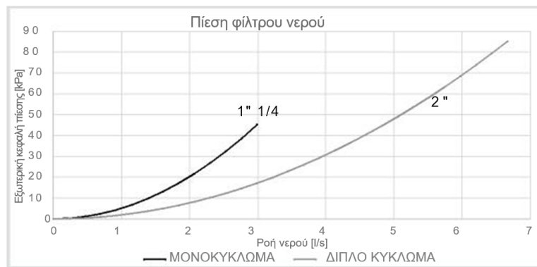
Εικόνα 11 - Πτώσεις πίεσης του φίλτρου νερού
