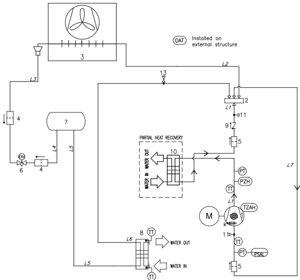
Εικόνα 18 - Διάγραμμα κυκλώματος ψυκτικού μέσου (P&ID) για μονάδα ΜΟΝΟΥ κυκλώματος ΕWYT~CZ
