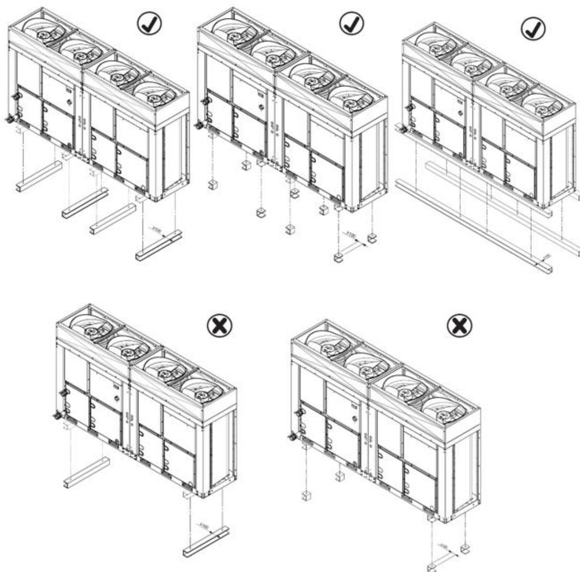
Εικόνα 4 – Τοποθέτηση ΔΙΠΛΗΣ μονάδας
