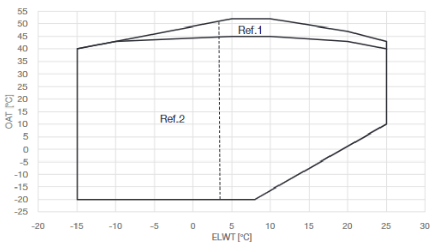
Figura 14 –Límites operativos en EWATCZ
