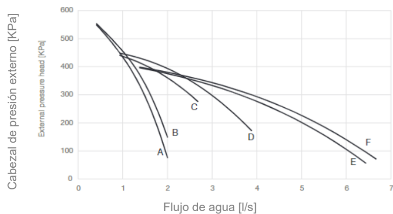
Figura 13 - Presión externa de bomba de elevación alta
