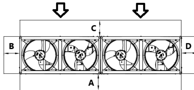
Figura 6 – Unidad DOBLE
