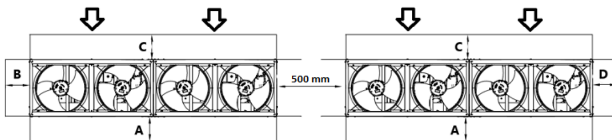
7. ábra – Rövid oldaluk – B vagy D – mentén egymás mellé telepített egységek
