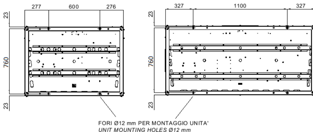
5. ábra – Szerelőnyílások elhelyezkedése (alulnézet)
