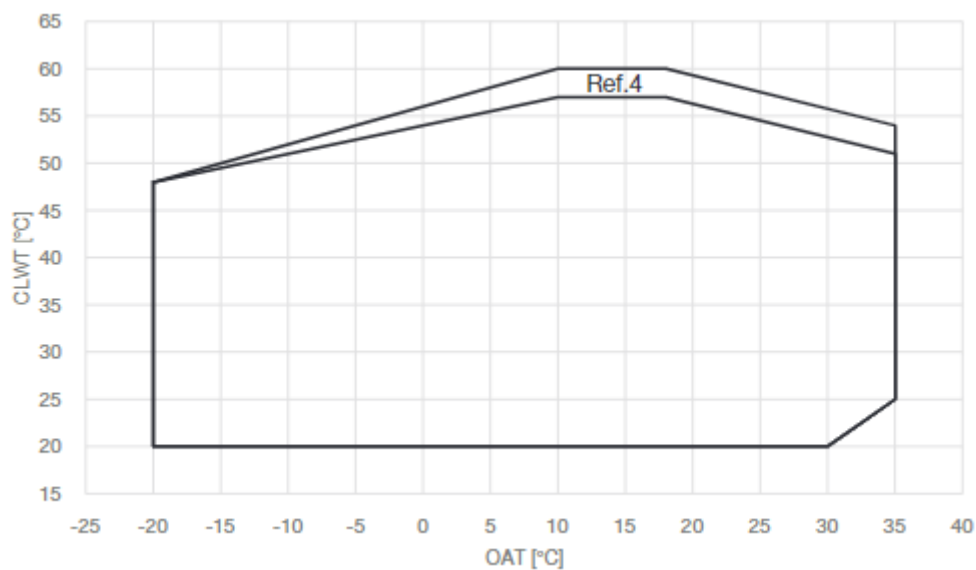
16. ábra - EWYTCZ üzemeltetési határértékei fűtés módban
