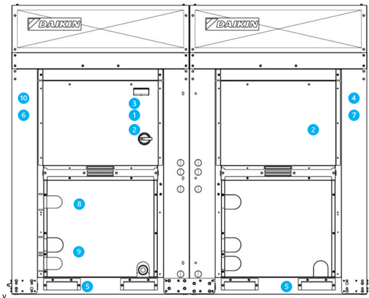
Rysunki 22 - Tabliczki na opakowaniu jednostki
