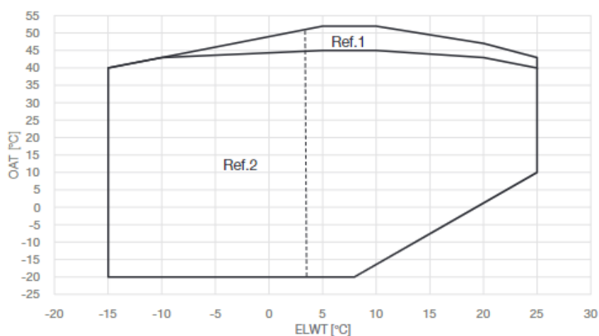
Rysunki 14 – Ograniczenia robocze EWATCZ
