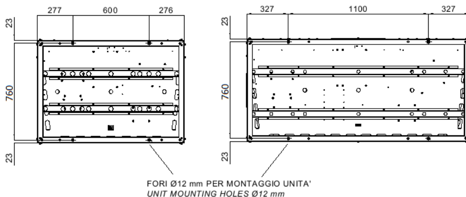
Rysunki 5 – Rozmieszczenie otworów montażowych (widok z dołu)
