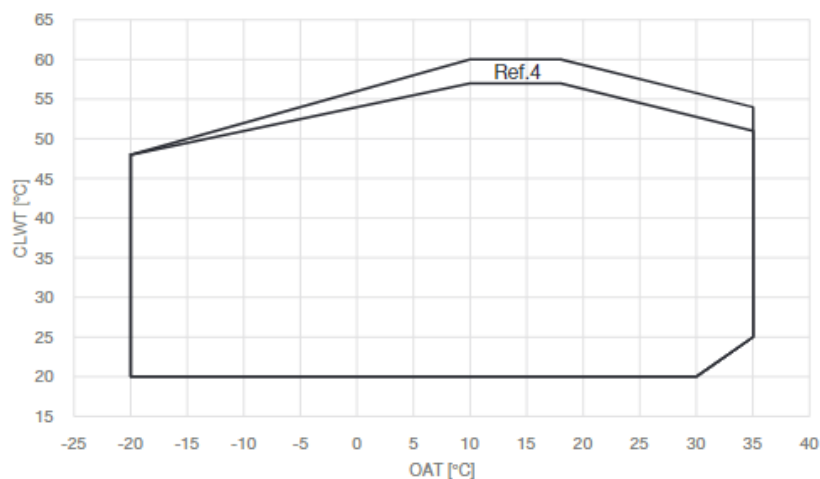
Rysunki 16 - Ograniczenia robocze EWTYCZ w trybie ogrzewania
