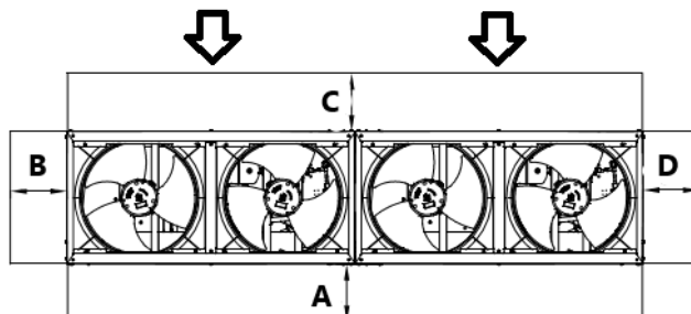
Rysunki 6 – Jednostka DUAL
