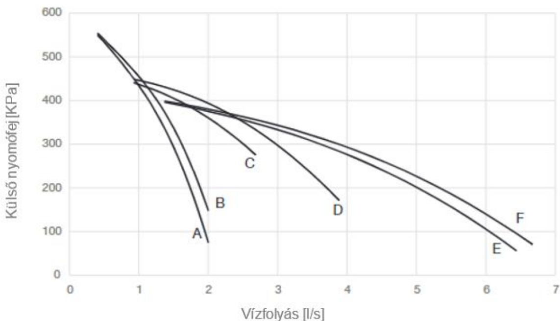
13. ábra - Nagy emelőmagasságú szivattyú külső nyomáscúcsa
