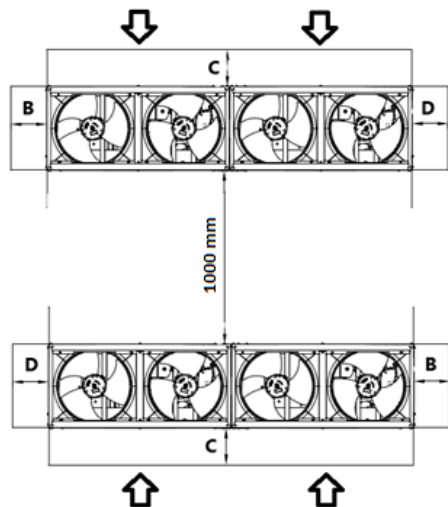
8. ábra – Hosszú oldaluk – 1. vagy 2. példa – mentén egymás mellé telepített egységek
