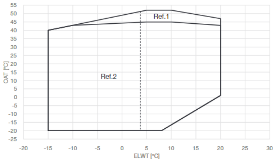
15. ábra - EWYT-CZ üzemeltetési határértékei hűtés módban
