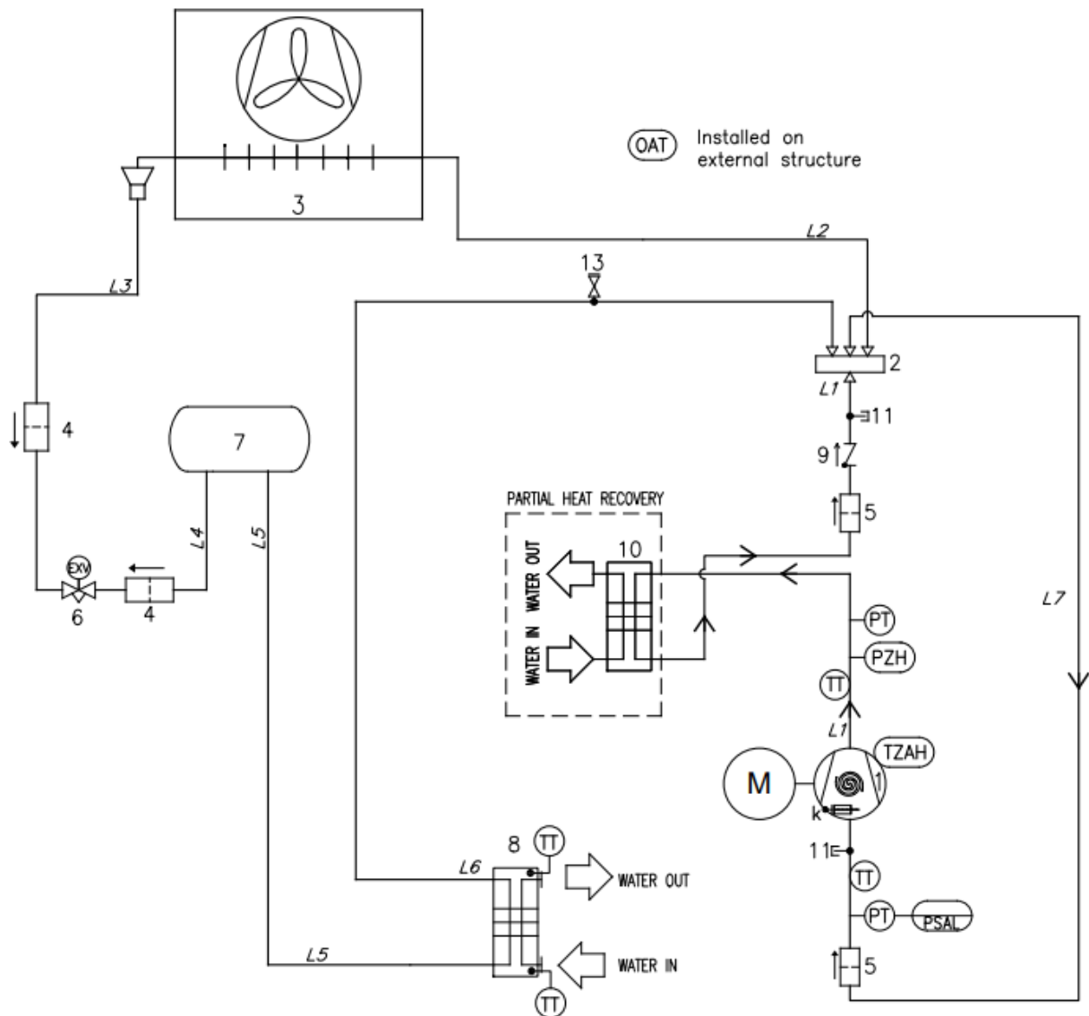
Figura 18 - Esquema do circuito de refrigeração (P&ID) para a unidade EWYT ~CZ circuito MONO
