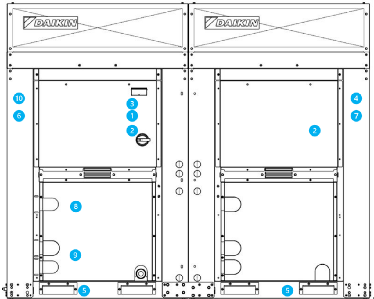
Figura 22 - Etiquetas na unidade
