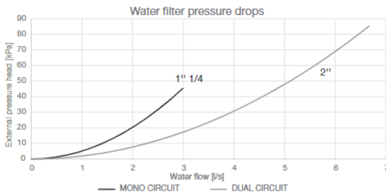
Figura 11 - Perda de carga do filtro de água
