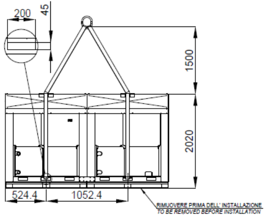
Figura 2 –Levantamento da unidade DUAL
