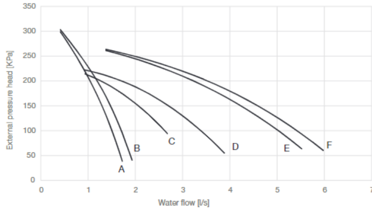
Figura 12 - Cabeçote de pressão externa de elevação baixa da bomba
