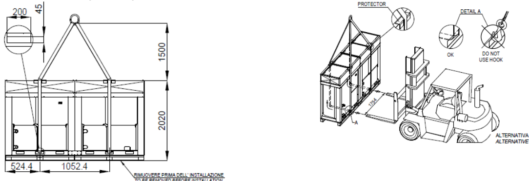
Obrázek 2 – Zvedání jednotky DUAL
