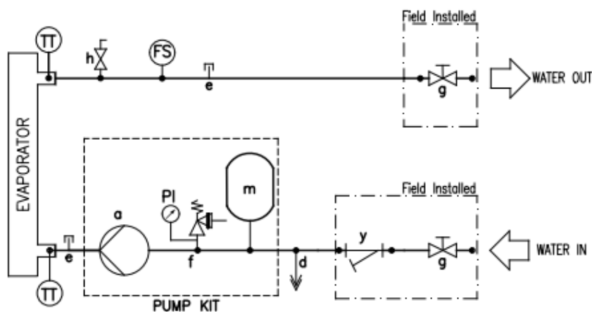
Obrázek 10 – Hydraulické schéma
