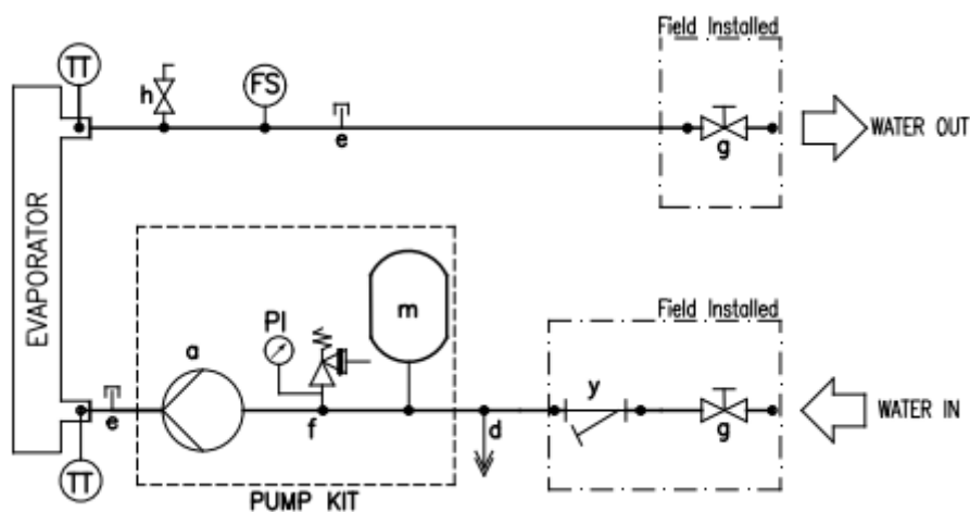
Εικόνα 10 – Υδραυλικό διάγραμμα
