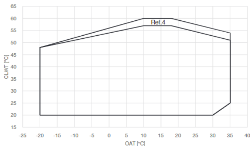
Εικόνα 16 - Όρια λειτουργίας στο EWYTCZ σε λειτουργία θέρμανσης
