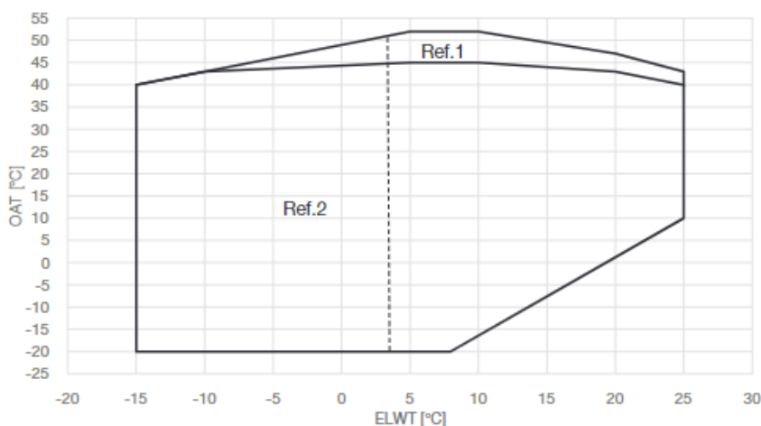
Εικόνα 14 - Όρια λειτουργίας στο EWATCZ
