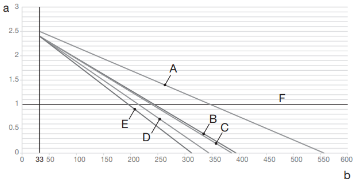
17. ábra - Tágulási tartály kezdeti nyomása a maximális víztérfogat alapján
