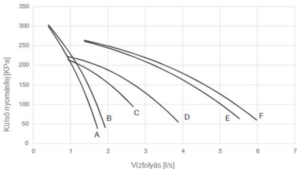
12. ábra - Kis emelőmagasságú szivattyú külső nyomáscsúcsa
