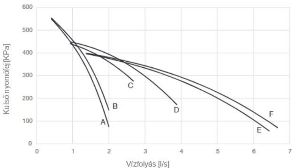
13. ábra - Nagy emelőmagasságú szivattyú külső nyomáscsúcsa
