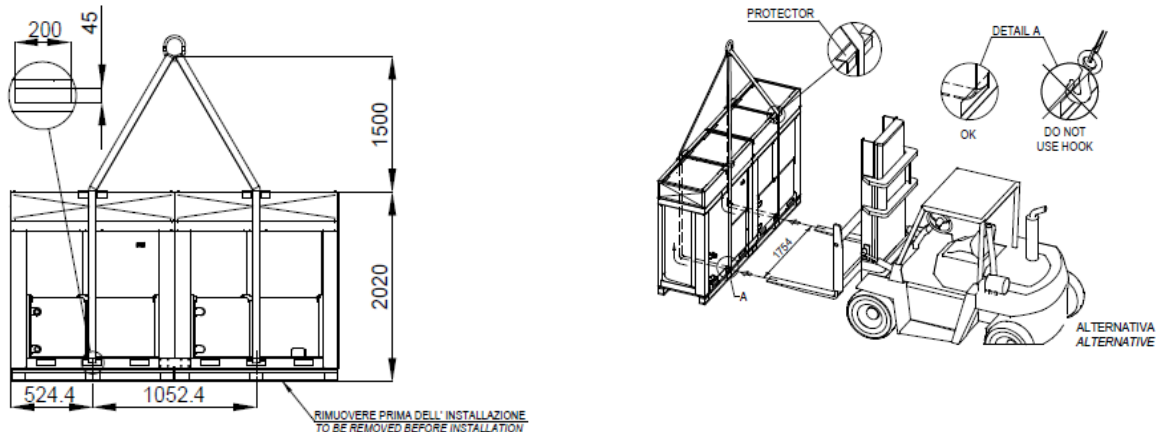
Figura 2 –Levantamento da unidade DUAL
