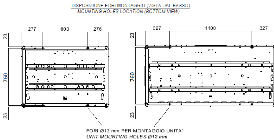
Figura 5 –Localização dos orifícios de montagem (vista inferior)
