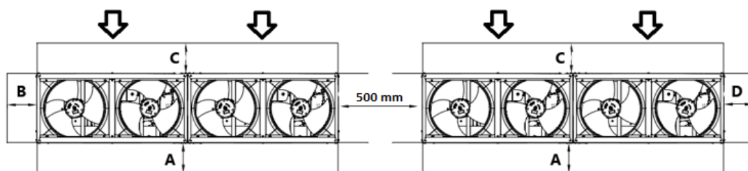
Figura 7 –Unitățile instalate alăturat pe laturile mai scurte, B sau D
