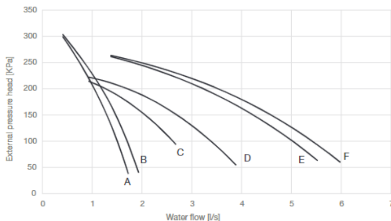
Figura 12 - Căderea relativă de presiune externă a pompei de presiune joasă
