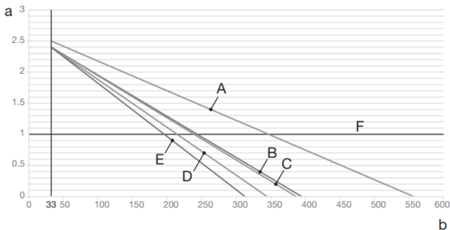
Figur 17 - Utgångstryck för expansionskärl på grundval av maximal vattenvolym
