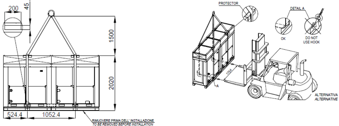
Figur 2 –Lyft av DUAL-enheten
