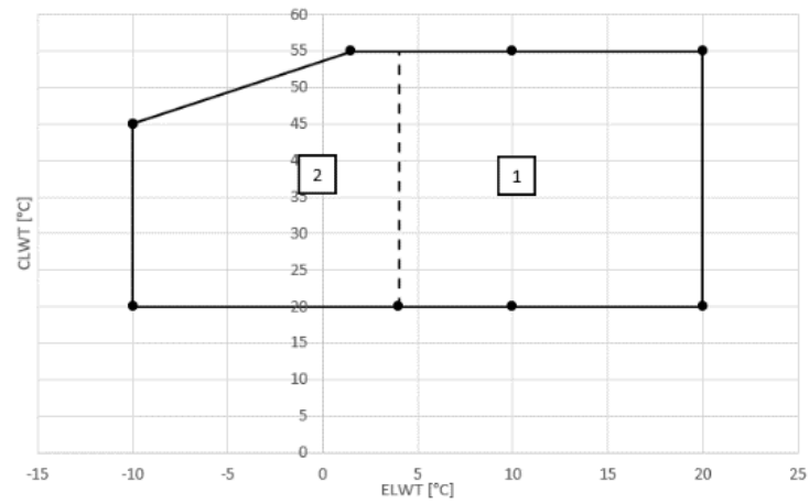
Εικόνα 4 - Όρια λειτουργίας EWWQ049-064
