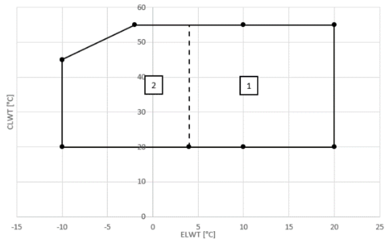
Εικόνα 4 - Όρια λειτουργίας EWWQ049-064
