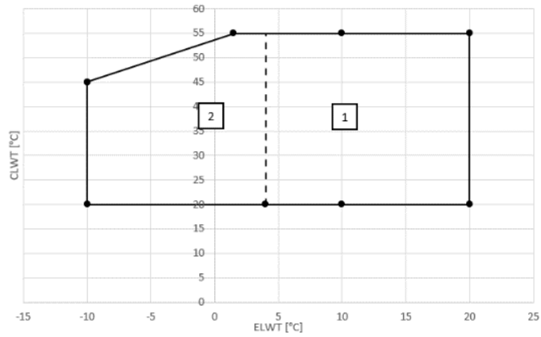
Figur 4- Driftsgränser EWWQ049-064
