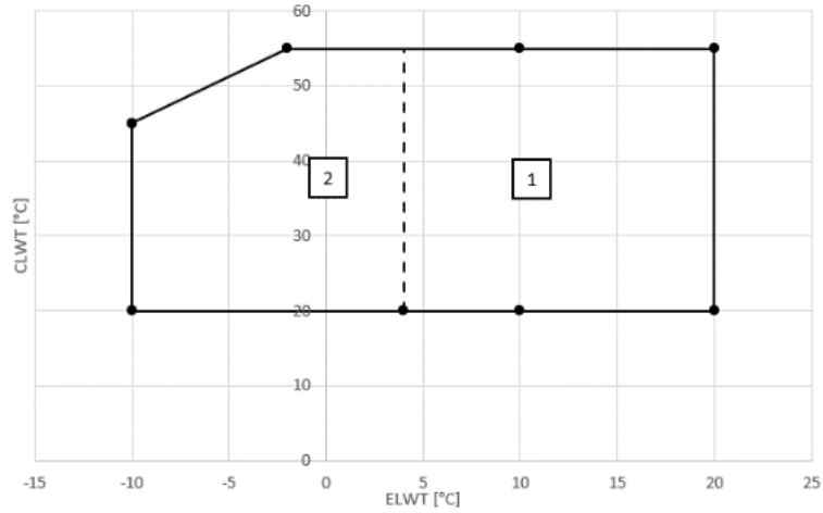
Figur 4- Driftsgränser EWWQ049-064
