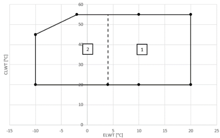
Abbildung 4 - Betriebsgrenzen EWWQ049-064
