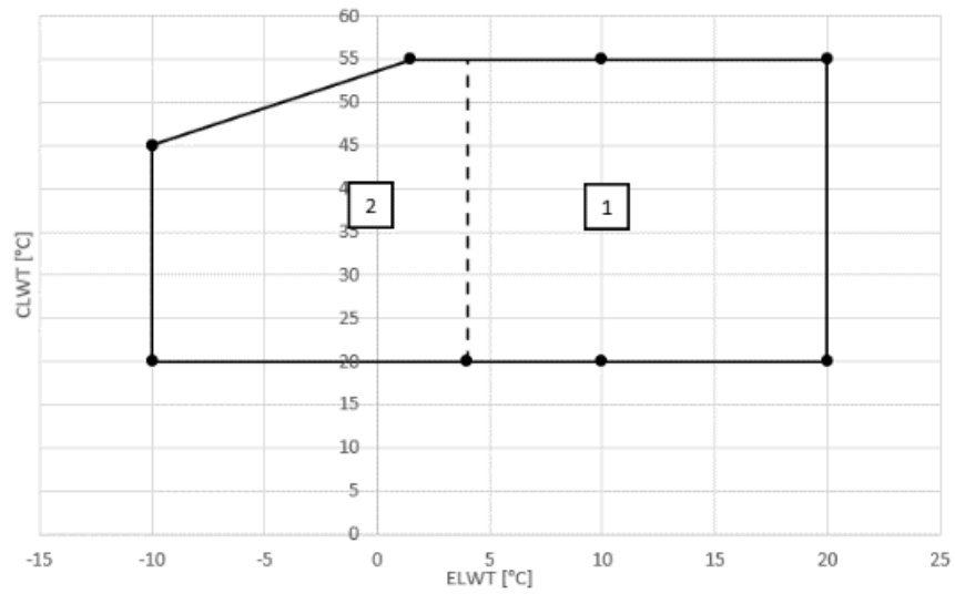
Figure 3- Plage de fonctionnement EWWQ014-033
