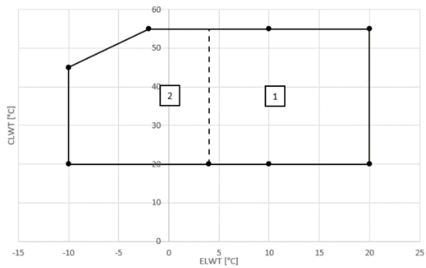
Figure 4- Plage de fonctionnement EWWQ049-064
