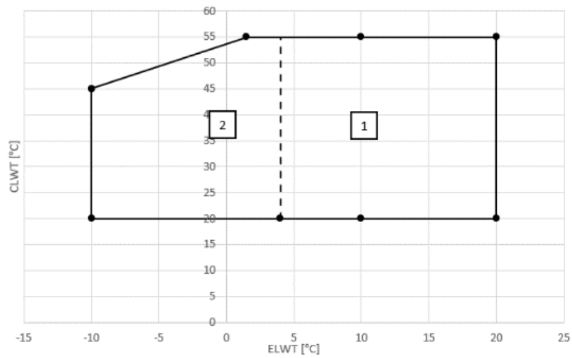
Rysunek 3 - Ograniczenia robocze w przypadku EWWQ014-033
