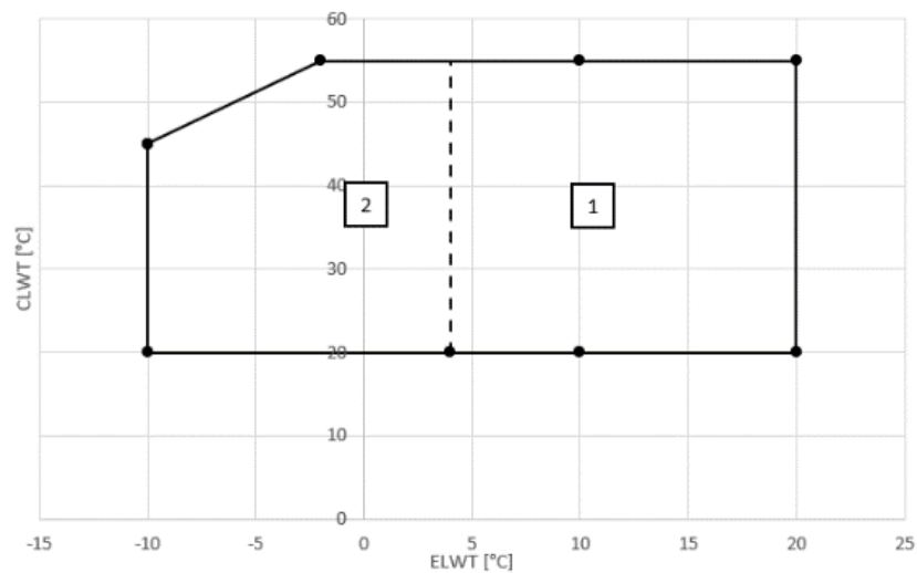
Rysunek 4 - Ograniczenia robocze w przypadku EWWQ049-064
