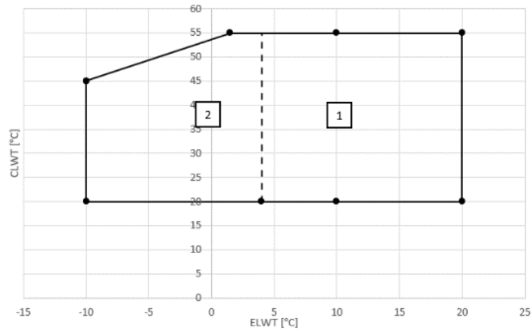
Figura 3 - Limites operativos em EWWQ014-033
