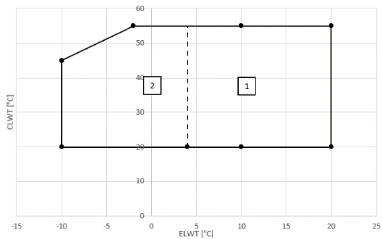
Figura 4 - Limites operativos EWWQ049-064
