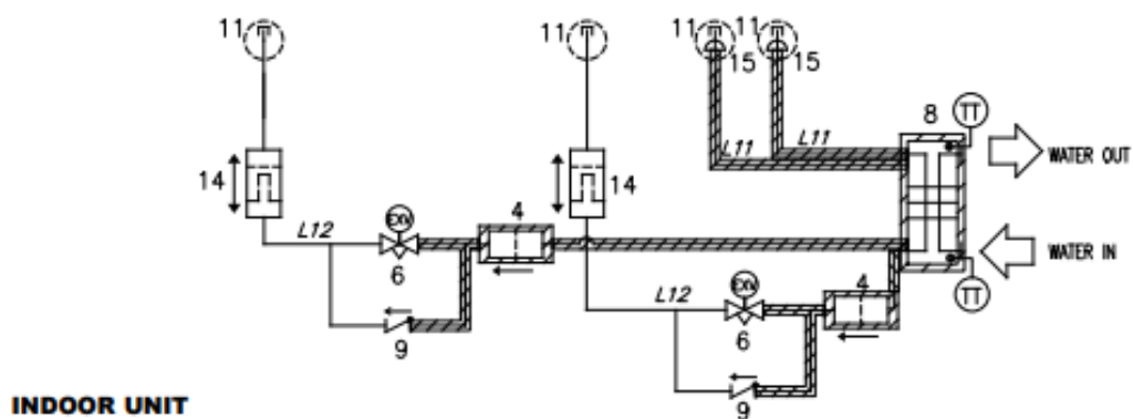
Εικόνα 25 – Διάγραμμα κυκλώματος ψυκτικού μέσου (P&ID) για εσωτερική μονάδα ΔΙΠΛΟΥ κυκλώματος EWYT-CZ
