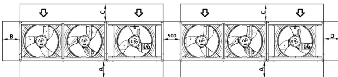
Afbeelding 10 – Eenheden naast elkaar geïnstalleerd langs hun kortere zijden, B of D
