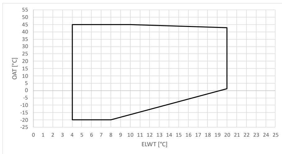
Rysunek 1 – Ograniczenia robocze EWYT_CZ w trybie chłodzenia
